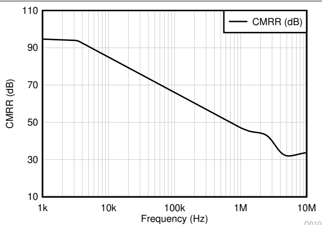
图 5-27. CMRR 与频率之间的关系
