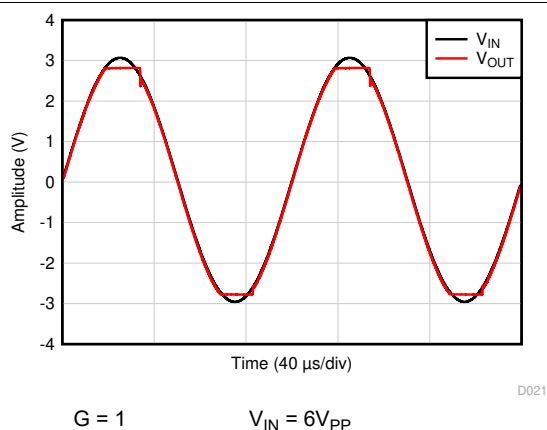
图 5-41. 无相位反转
