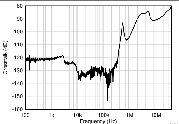
图 5-53. 通道隔离
