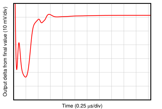
图 5-45. 小信号阶跃响应
