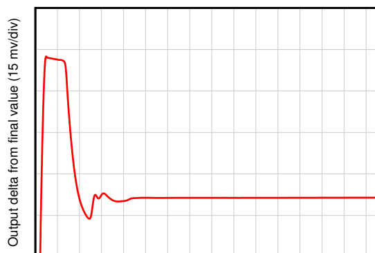
图 5-46. 大信号阶跃响应
