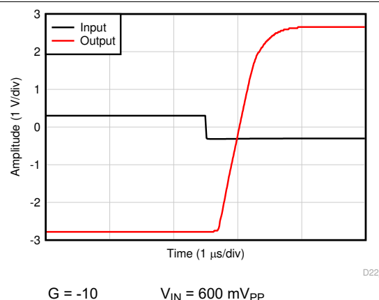
图 5-42. 过载恢复
