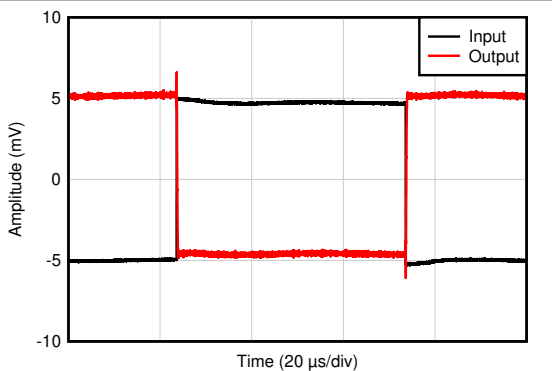
图 5-43. 过载恢复
