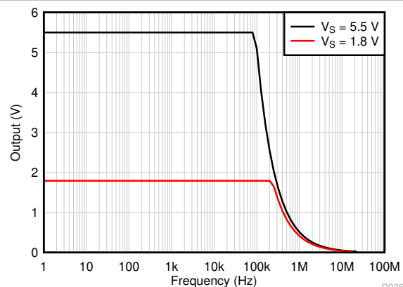
图 5-50. 最大输出电压与频率间的关系
