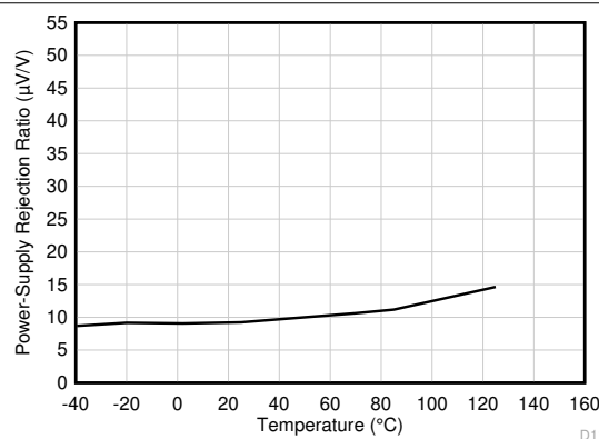
图 5-26. 直流 PSRR 与温度间的关系
