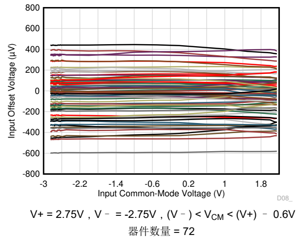
图 5-10. 失调电压与共模间的关系
