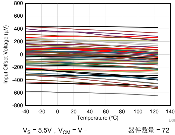
图 5-7. 输入失调电压与温度间的关系
