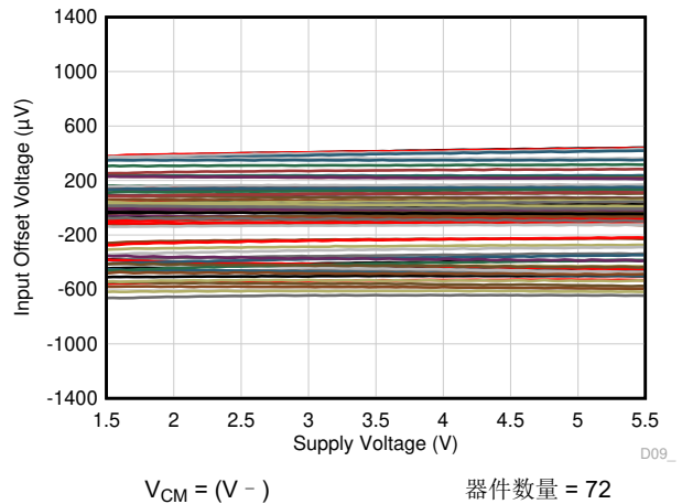
图 5-12. 偏移电压与电源电压间的关系
