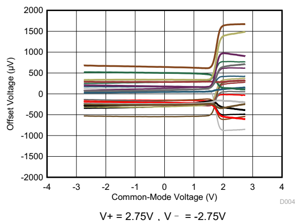
图 6-2. TLV900x 失调电压与共模间的关系
