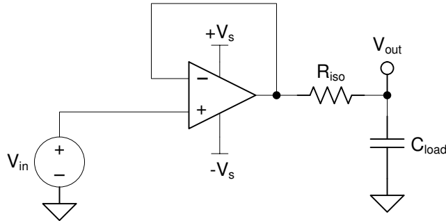
图 6-3. 增强容性负载驱动能力
