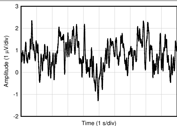
图 5-29. 0.1Hz 至 10Hz 时域电压噪声
