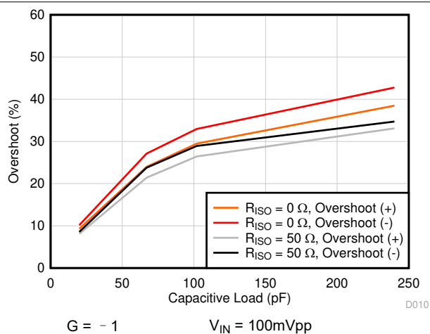
图 5-38. 小信号过冲与容性负载间的关系
