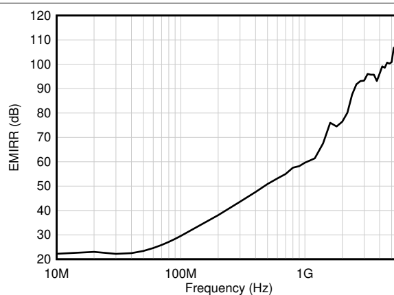
图 5-52. 以同相输入为基准的电磁干扰抑制比 (EMIRR+) 与频率间的关系
