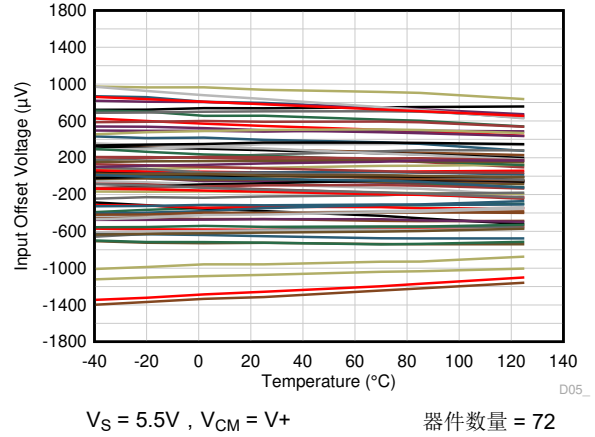
图 5-8. 输入失调电压与温度间的关系
