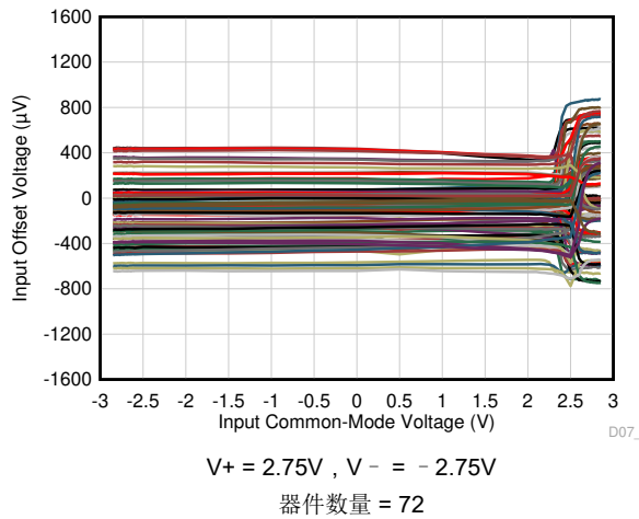
图 5-9. 失调电压与共模间的关系
