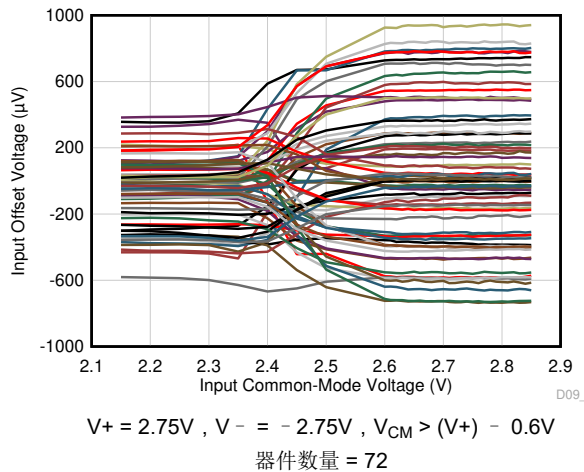
图 5-11. 失调电压与共模间的关系
