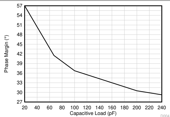
图 5-40. 相位裕度与容性负载间的关系
