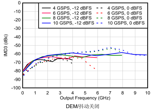
图 6-145. NRZ/RF 模式下 IMD3 与频率和采样速率间的关系
