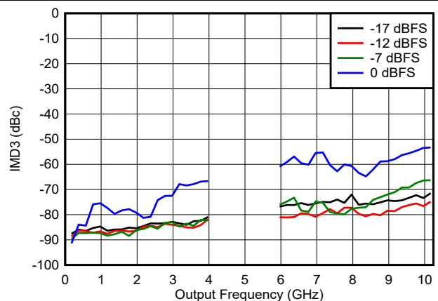
图 6-135. NRZ/RF 模式下 IMD3 与频率和数字振幅间的关系
