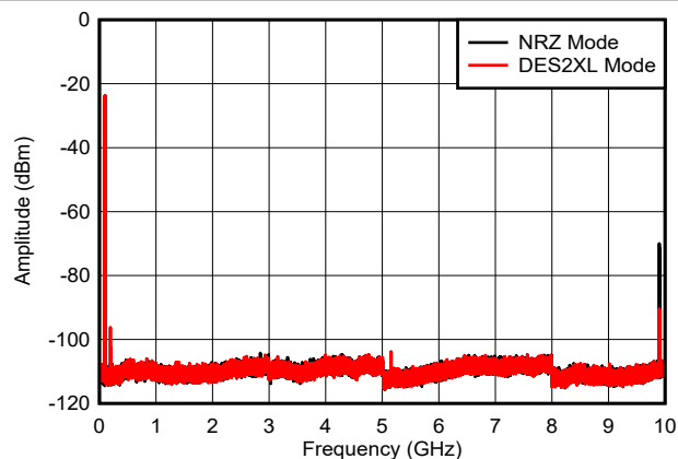
图 6-39. 双音， f_{\text{OUT}} = 97\text{MHz} ， -6\text{dBFS} ( 0 - f_{\text{CLK}} )
