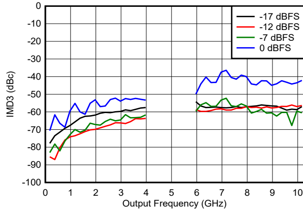
图 6-138. DES2X 模式下 IMD3 与频率和数字振幅间的关系
