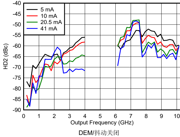
图 6-158. DES2X 模式下 HD2 与频率和输出电流间的关系
