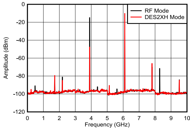
图 6-31. f_{\text{OUT}} = 6097\text{MHz} ，0dBFS
