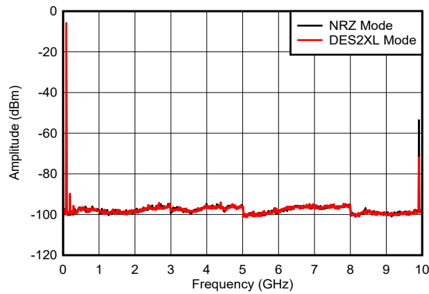
图 6-19. f_{\text{OUT}} = 97\text{MHz} ，0dBFS
