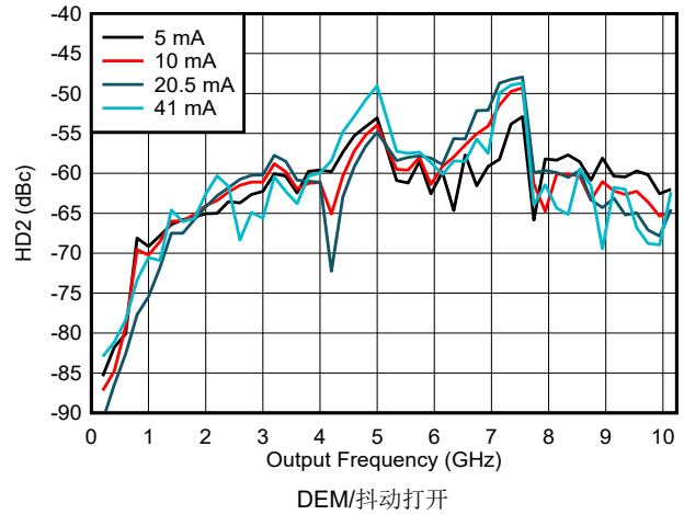
图 6-157. NRZ/RF 模式下 HD2 与频率和输出电流间的关系
