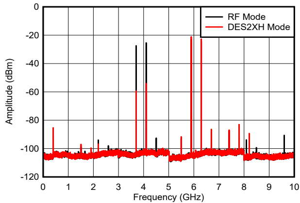
图 6-51. 双音， f_{\text{OUT}} = 3497\text{MHz} ，-12dBFS
