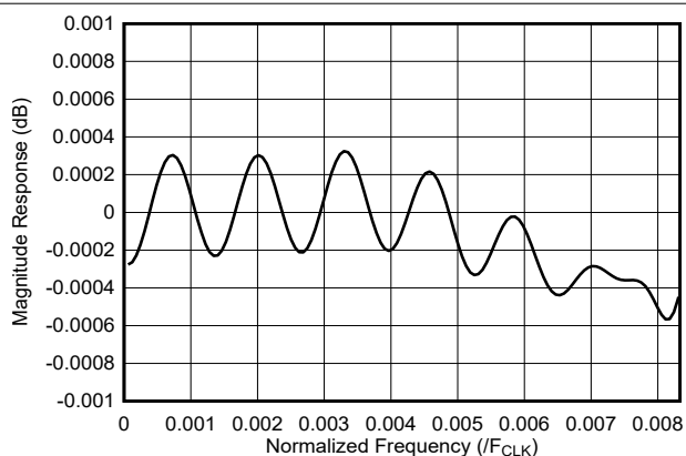
图 7-33. 48 倍内插滤波器通带响应
