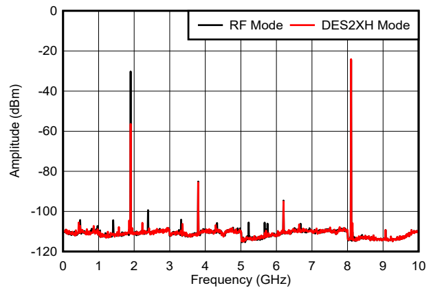
图 6-34. f_{\text{OUT}} = 8097\text{MHz} ，0dBFS
