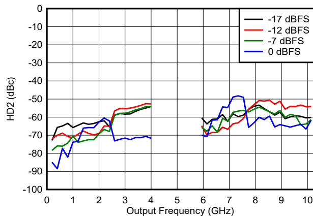
图 6-164. DES2X 模式下 HD2 与频率和数字振幅间的关系
