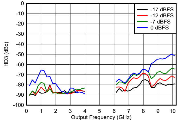
图 6-181. DES2X 模式下 HD3 与频率和数字振幅间的关系
