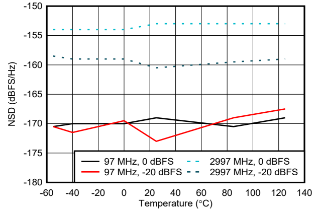
图 6-81. NSD 与温度间的关系
