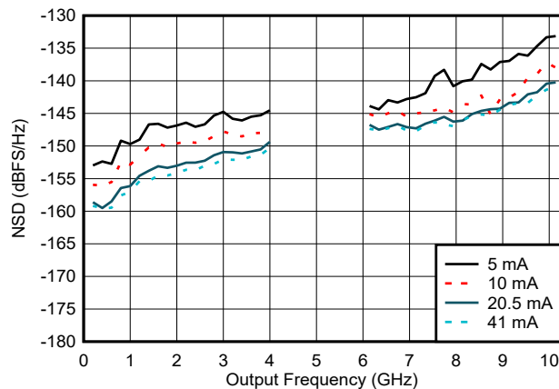
图 6-62. NSD 与输出频率和输出电流间的关系
