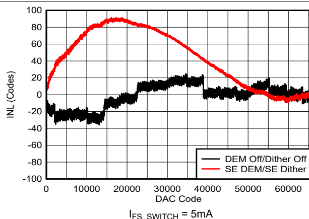
图 6-14. INL 与 DAC 代码间的关系：5mA
