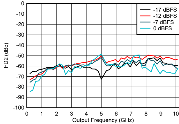
图 6-162. NRZ/RF 模式下 HD2 与频率和数字振幅间的关系
