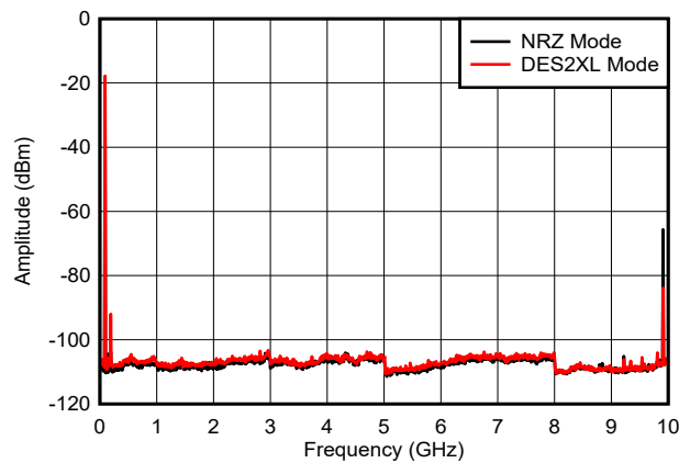
图 6-19. f_{\text{OUT}} = 97\text{MHz} ，0dBFS
