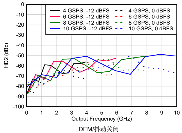
图 6-171. DES2X 模式下 HD2 与频率和采样速率间的关系
