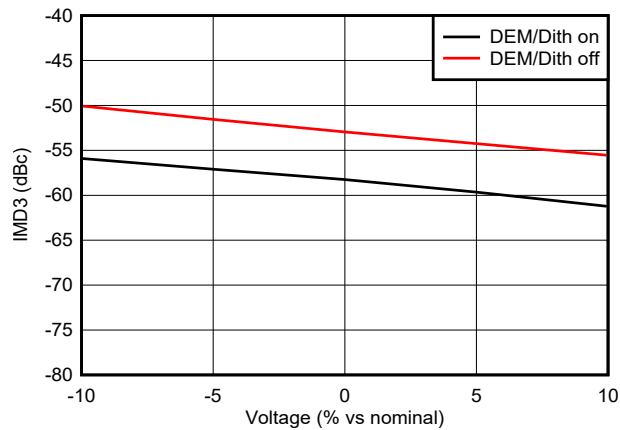
图 6-154. 7247MHz RF 模式下 IMD3 与电压间的关系
