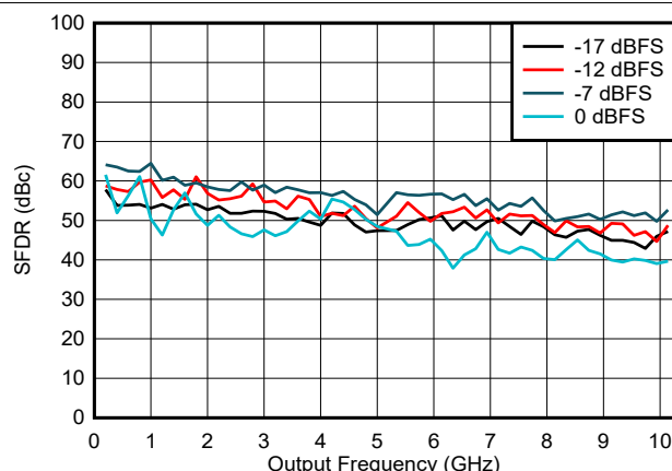
图 6-116. NRZ/RF 模式下 SFDR 与频率和数字振幅间的关系
