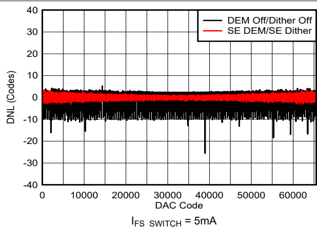
图 6-12. DNL 与 DAC 代码间的关系：5mA
