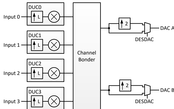
图 7-13. 具有实数输出的 DUC 块
