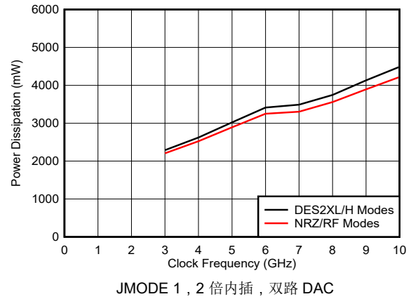
图 6-92. 功率损耗与时钟频率和 DAC 模式间的关系
