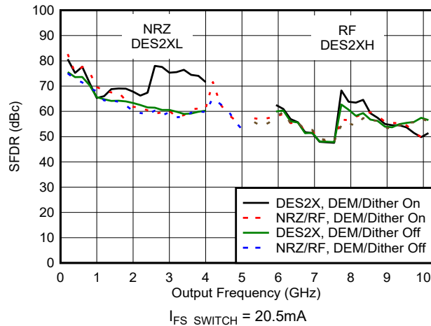
图 6-104. SFDR 与频率和模式间的关系
