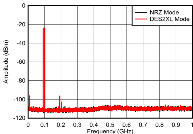
图 6-40. 双音， f_{\text{OUT}} = 97\text{MHz} ， -6\text{dBFS} ( 0\text{GHz} 至 1\text{GHz} )
