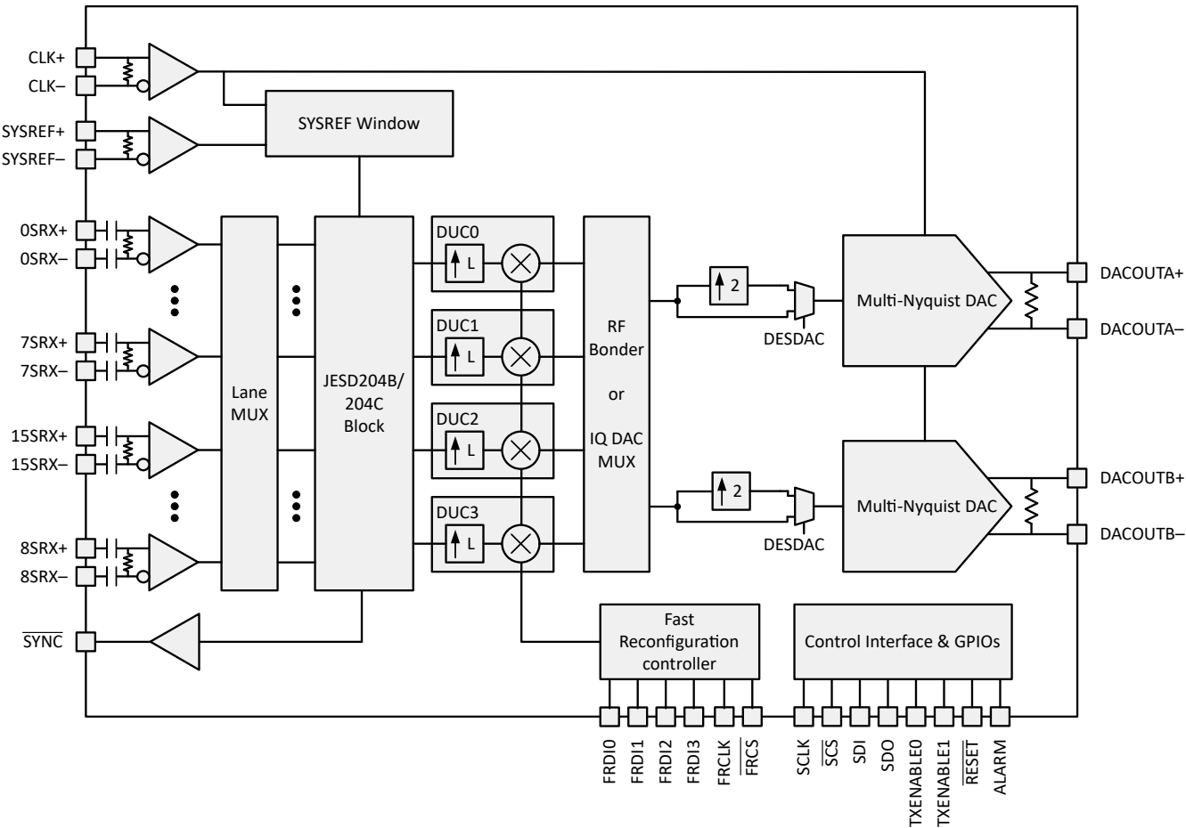
图 7-1. 双通道器件
