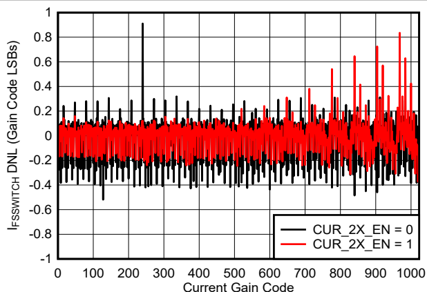
图 6-18. I_{\text{FS\_SWITCH}} 误差差分非线性与增益代码间的关系
