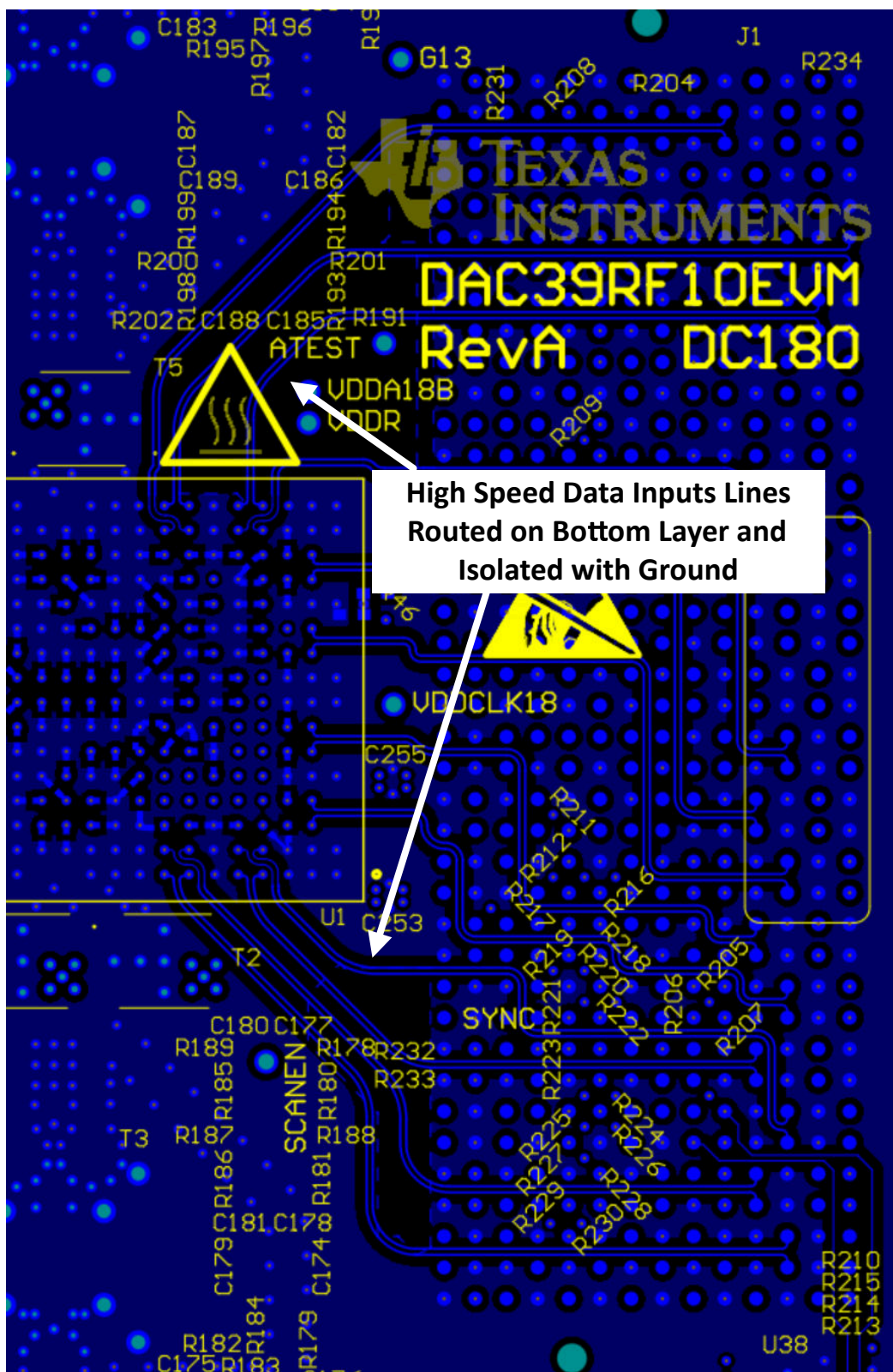
图 8-30. 具有接地隔离的串行器/解串器底层布线
