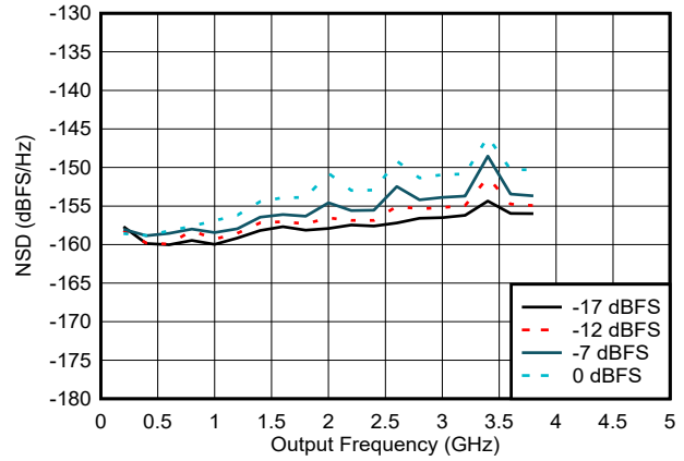
图 6-75. NSD 与输出频率和数字振幅间的关系
