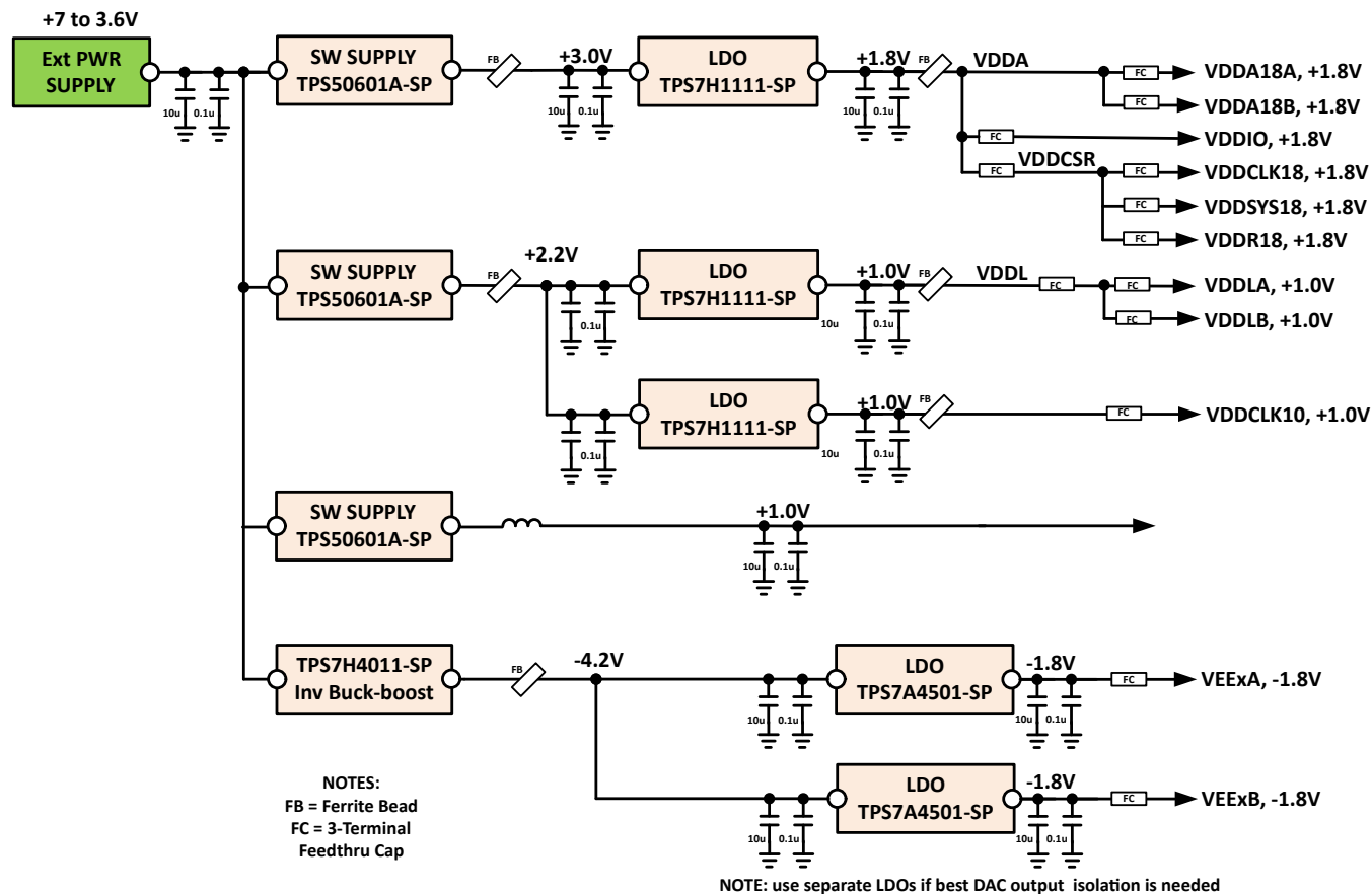
图 8-22. 推荐的 -SP 电源方框图
