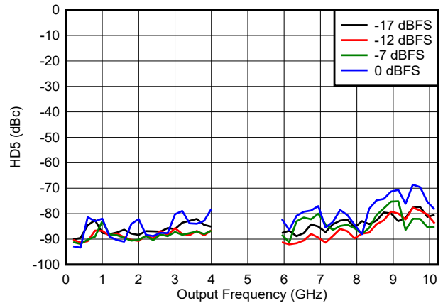
图 6-199. NRZ/RF 模式下 HD5 与频率和数字振幅间的关系
