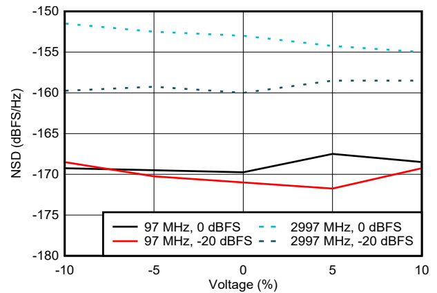
图 6-85. NSD 与电源电压间的关系
