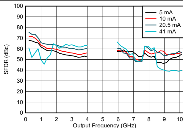
图 6-114. DES2X 模式下 SFDR 与频率和输出电流间的关系
