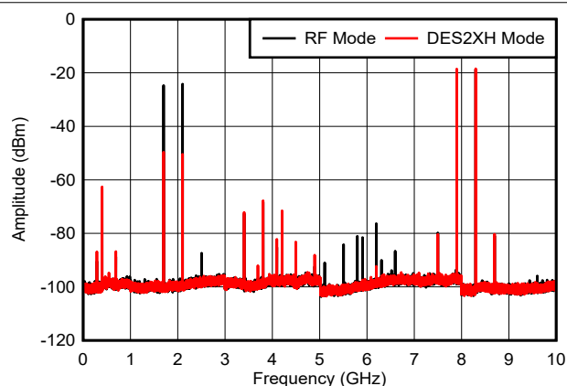
图 6-55. 双音， f_{\text{OUT}} = 8097\text{MHz} ，0dBFS
