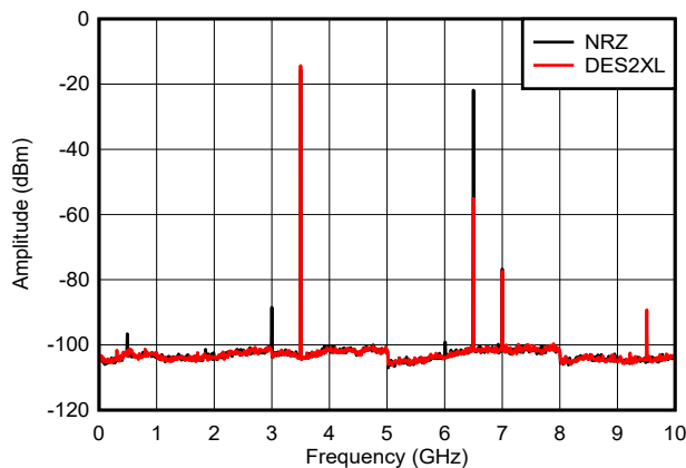
图 6-27. f_{\text{OUT}} = 2097\text{MHz} ，-12dBFS
