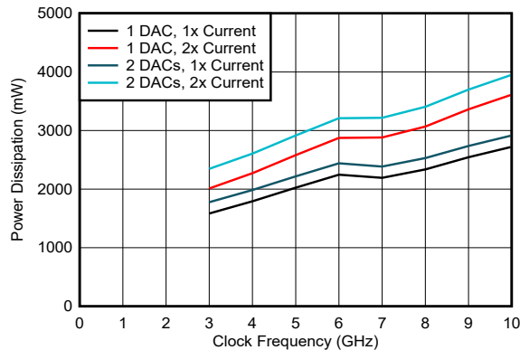
图 6-93. 功率损耗与时钟频率和 DAC 模式间的关系
