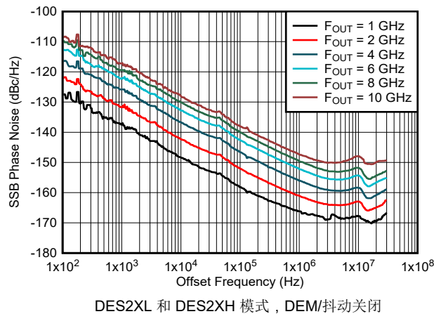
图 6-218. 相位噪声与偏移频率和输出频率间的关系
