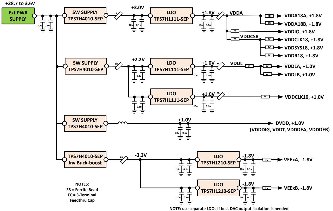
图 8-23. 推荐的 -SEP 电源方框图
