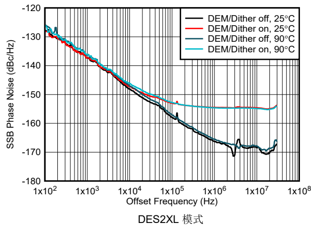
图 6-220. 1GHz 条件下相位噪声与偏移频率间的关系
