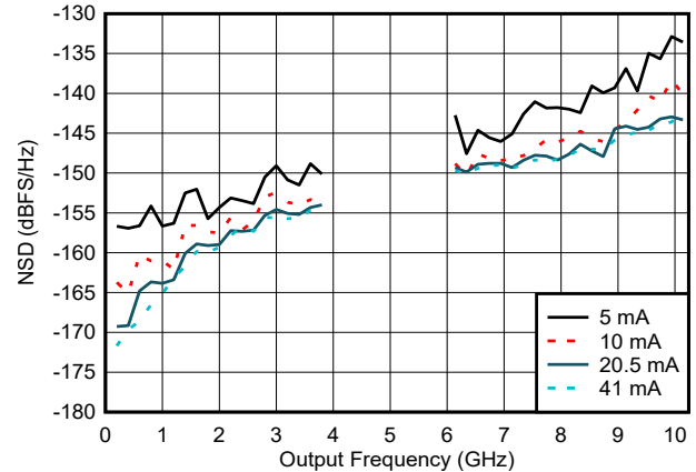
图 6-63. NSD 与输出频率和输出电流间的关系
