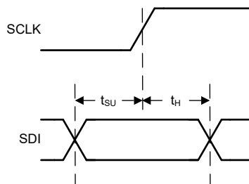
图 6-2. SPI 数据输入时序图
