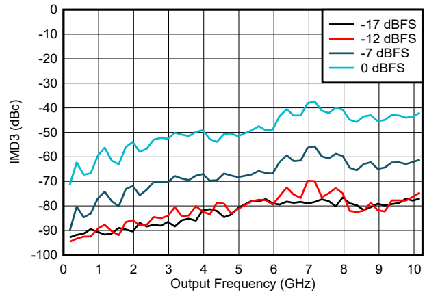
图 6-133. NRZ/RF 模式下 IMD3 与频率和数字振幅间的关系
