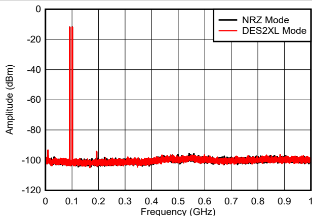
图 6-38. 双音， f_{\text{OUT}} = 97\text{MHz} ， 0\text{dBFS} ( 0\text{GHz} 至 1\text{GHz} )
