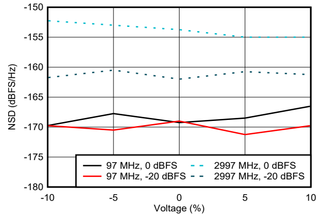
图 6-87. NSD 与电源电压间的关系
