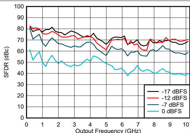
图 6-117. NRZ/RF 模式下 SFDR 与频率和数字振幅间的关系
