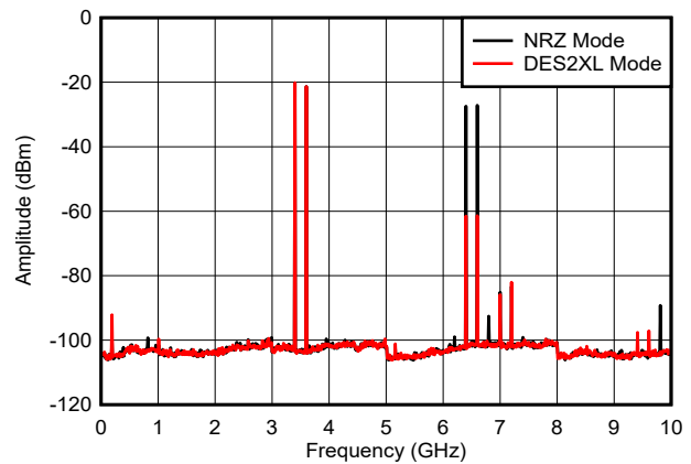
图 6-48. 双音， f_{\text{OUT}} = 2097\text{MHz} ， -12\text{dBFS}
