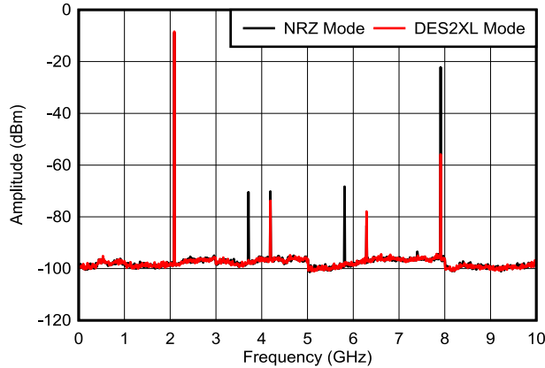
图 6-25. f_{\text{OUT}} = 2097\text{MHz} ，0dBFS
