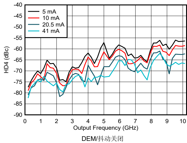
图 6-188. NRZ/RF 模式下 HD4 与频率和输出电流间的关系
