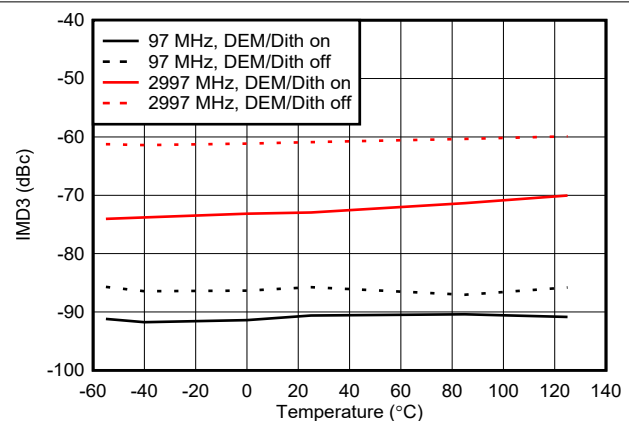
图 6-149. DES2XL 模式下 IMD3 与温度间的关系
