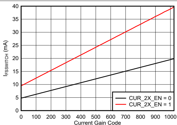
图 6-15. I_{\text{FS\_SWITCH}} 与增益代码间的关系
