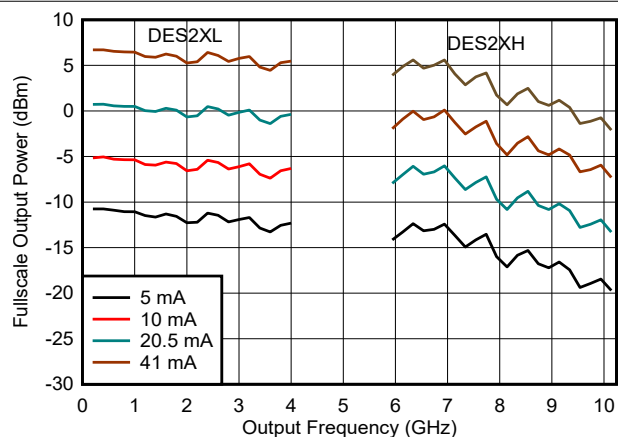
图 6-8. 输出响应与频率间的关系
