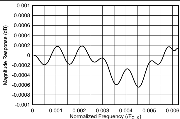
图 7-35. 64 倍内插滤波器通带响应
