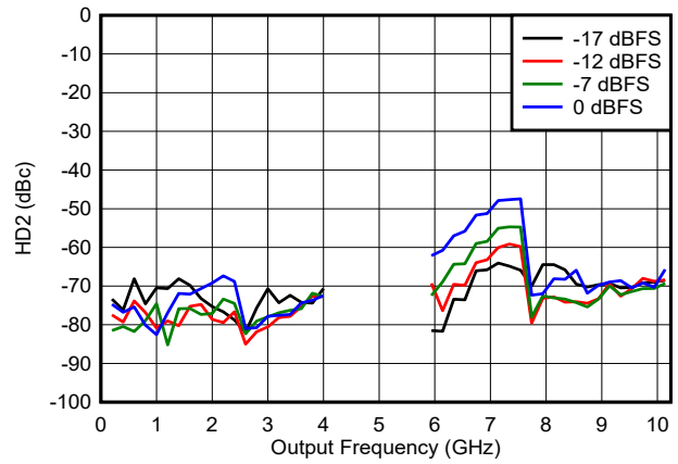
图 6-163. NRZ/RF 模式下 HD2 与频率和数字振幅间的关系
