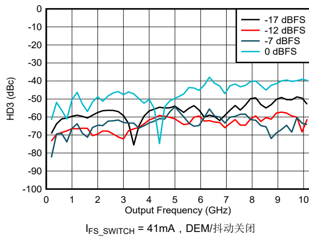
图 6-178. NRZ/RF 模式下 HD3 与频率和数字振幅间的关系
