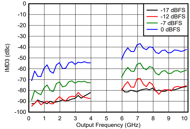
图 6-139. DES2X 模式下 IMD3 与频率和数字振幅间的关系
