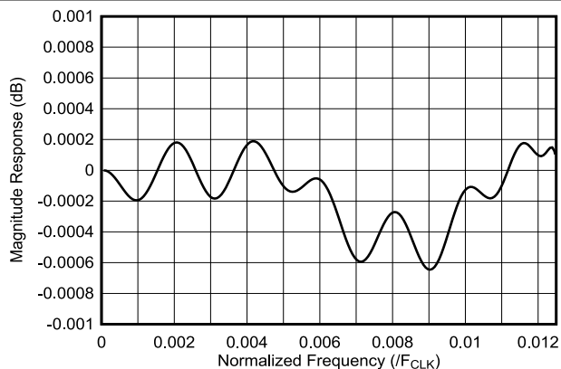
图 7-31. 32 倍内插滤波器通带响应
