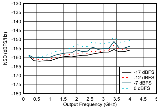
图 6-74. NSD 与输出频率和数字振幅间的关系
