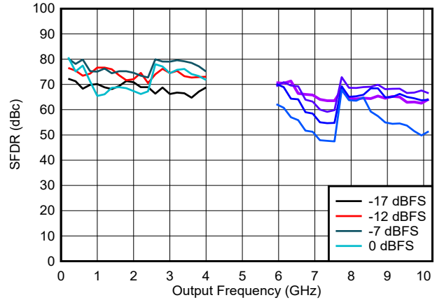
图 6-121. DES2X 模式下 SFDR 与频率和数字振幅间的关系
