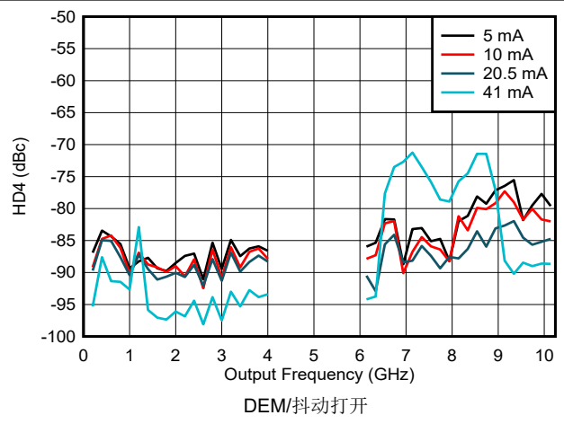
图 6-191. DES2X 模式下 HD4 与频率和输出电流间的关系
