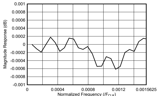
图 7-43. 256 倍内插滤波器通带响应
