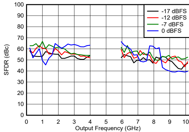
图 6-120. DES2X 模式下 SFDR 与频率和数字振幅间的关系
