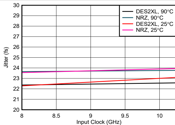
图 6-222. 抖动与输入时钟间的关系
