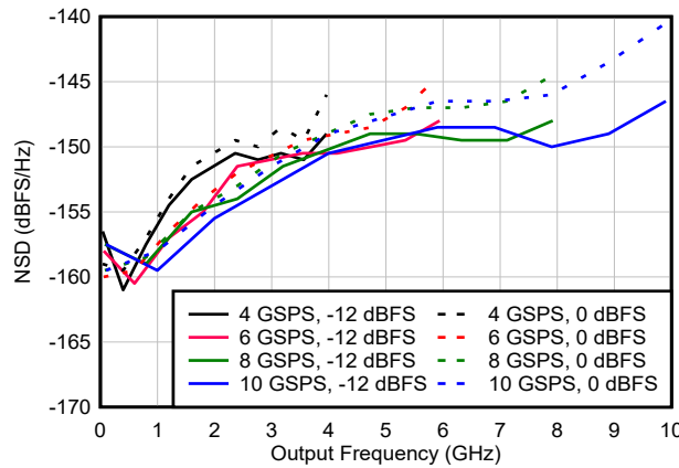
图 6-76. NSD 与输出频率和数字振幅间的关系
