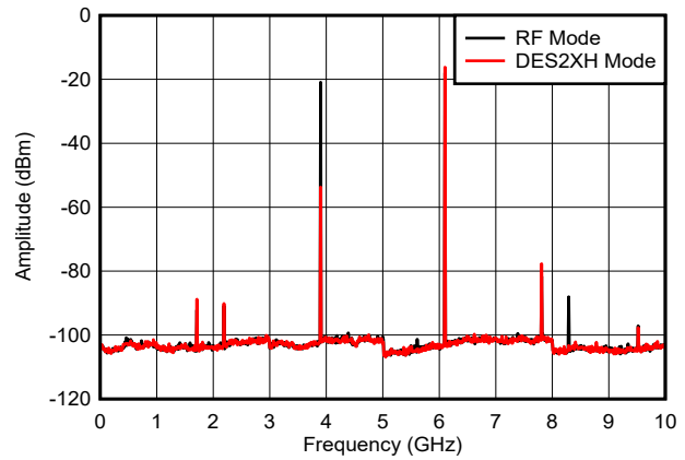
图 6-32. f_{\text{OUT}} = 6097\text{MHz} ，-6dBFS
