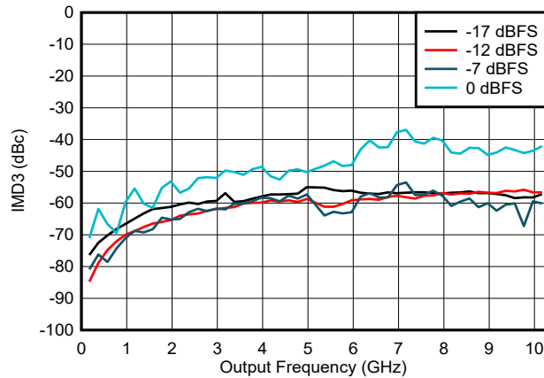
图 6-132. NRZ/RF 模式下 IMD3 与频率和数字振幅间的关系
