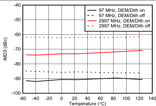
图 6-148. NRZ 模式下 IMD3 与温度间的关系
