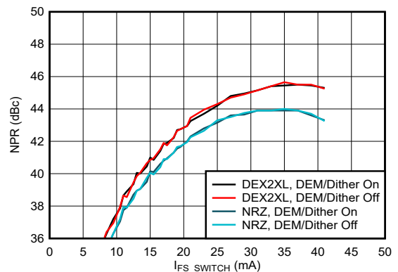
图 6-215. 电源抑制比与输出电流间的关系：第二奈奎斯特区域
