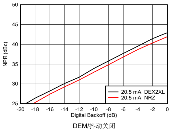
图 6-212. 噪声功率比与数字退避间的关系：第二奈奎斯特区域
