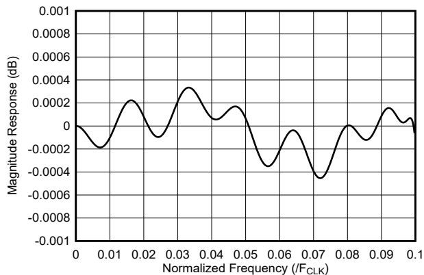
图 7-19. 4 倍内插滤波器通带响应
