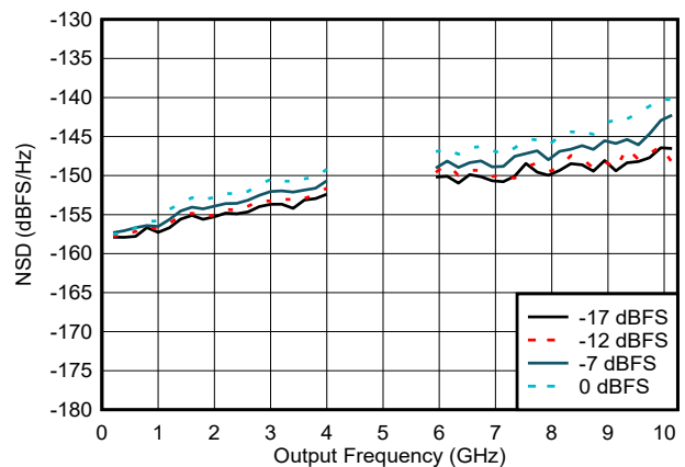
图 6-71. NSD 与输出频率和数字振幅间的关系
