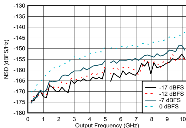
图 6-64. NSD 与输出频率和输出电流间的关系
