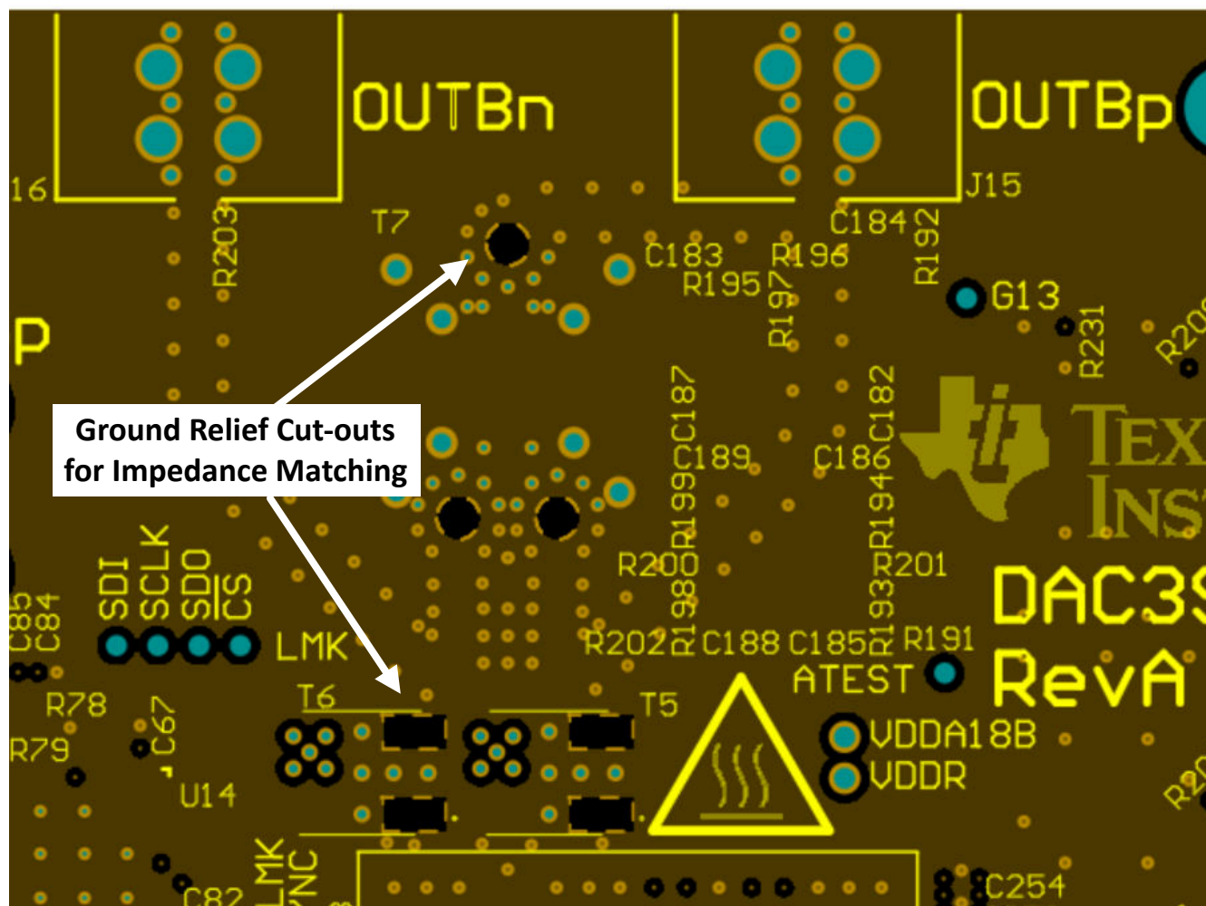
图 8-25. 平衡-非平衡变压器和 Bias-T 引脚下方的接地开孔
