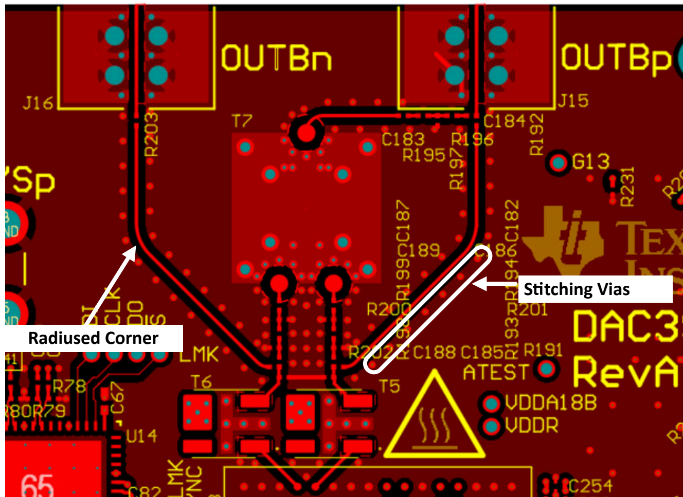
图 8-24. 高速信号布线旁边的半径角和拼接过孔
