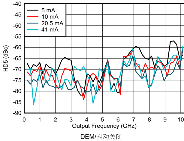
图 6-192. NRZ/RF 模式下 HD5 与频率和输出电流间的关系
