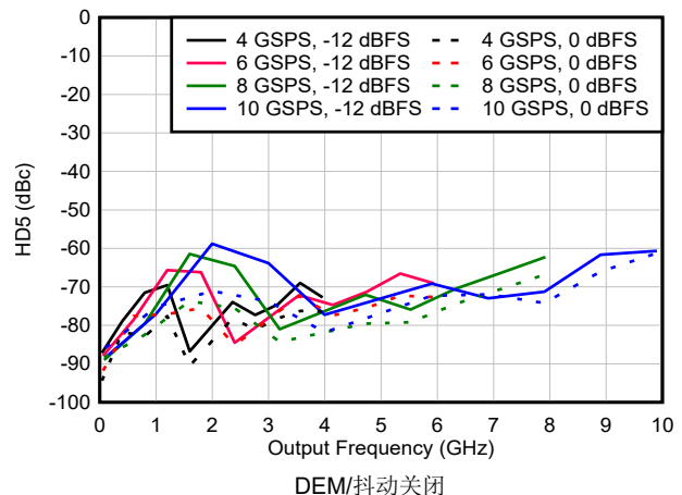
图 6-207. DES2X 模式下 HD5 与频率和采样速率间的关系
