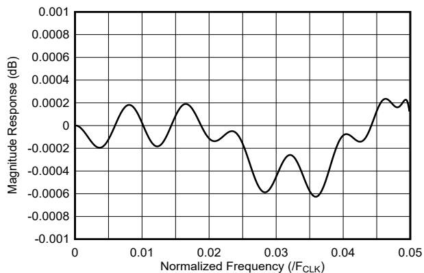
图 7-23. 8 倍内插滤波器通带响应
