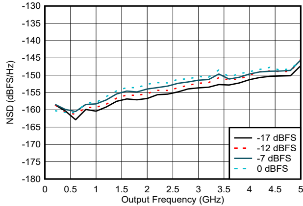
图 6-68. NSD 与输出频率和数字振幅间的关系
