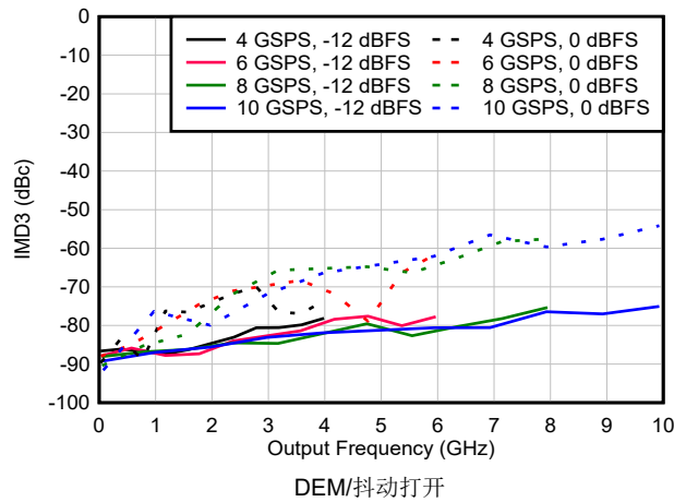
图 6-146. DES2X 模式下 IMD3 与频率和采样速率间的关系
