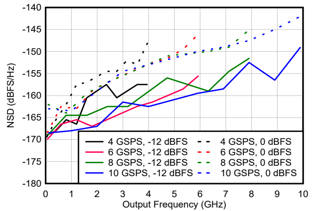
图 6-77. NSD 与输出频率和采样速率间的关系
