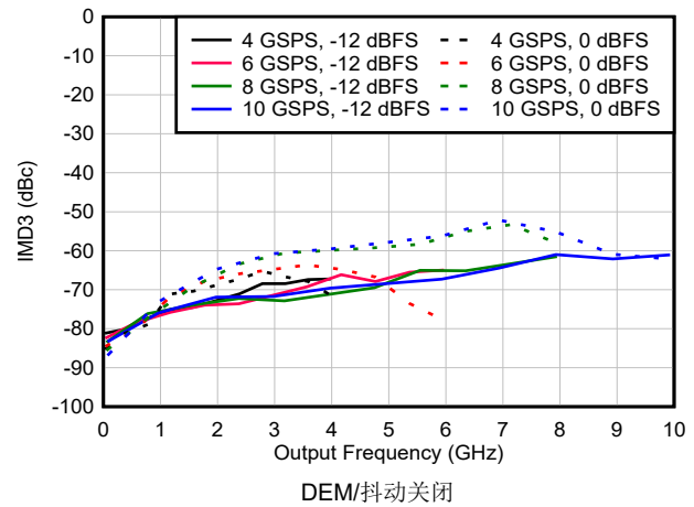
图 6-147. DES2X 模式下 IMD3 与频率和采样速率间的关系
