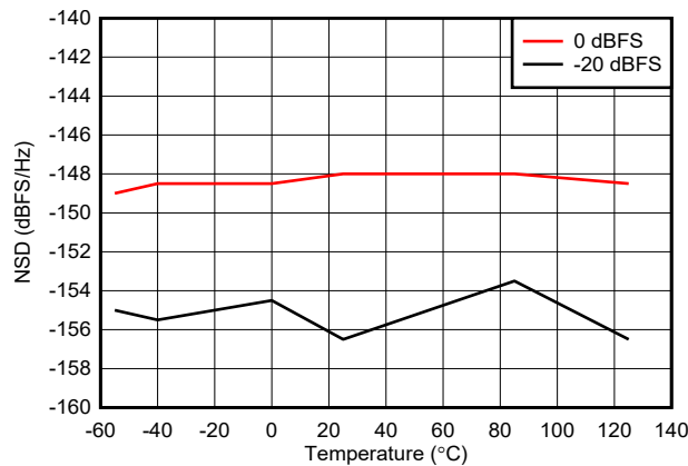
图 6-82. NSD 与温度间的关系
