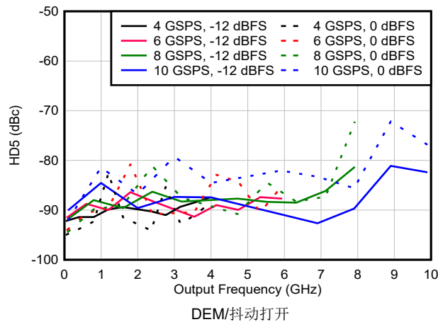
图 6-206. DES2X 模式下 HD5 与频率和采样速率间的关系
