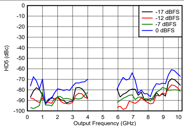
图 6-201. DES2X 模式下 HD5 与频率和数字振幅间的关系
