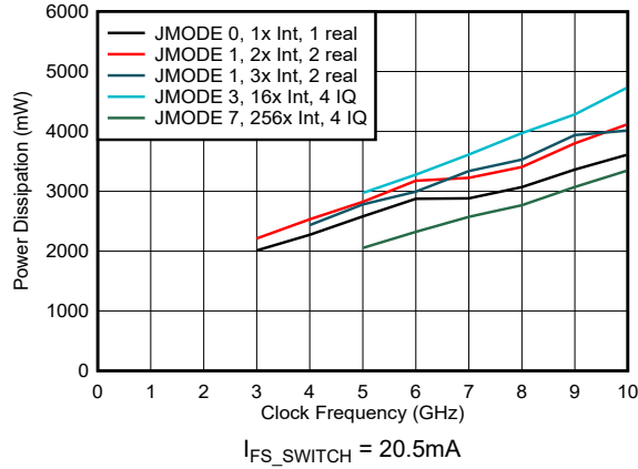
图 6-89. 功率损耗与时钟频率和数字模式间的关系
