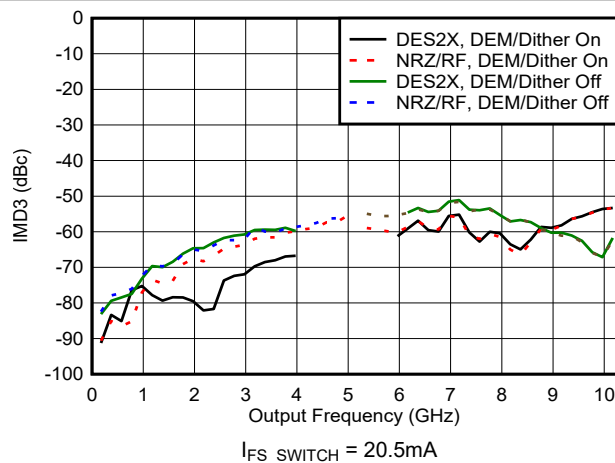
图 6-106. IMD3 与频率和模式间的关系
