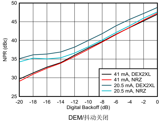
图 6-210. 噪声功率比与数字退避间的关系：第一奈奎斯特区域
