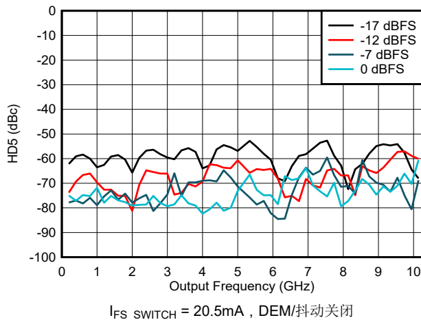
图 6-196. NRZ/RF 模式下 HD5 与频率和数字振幅间的关系
