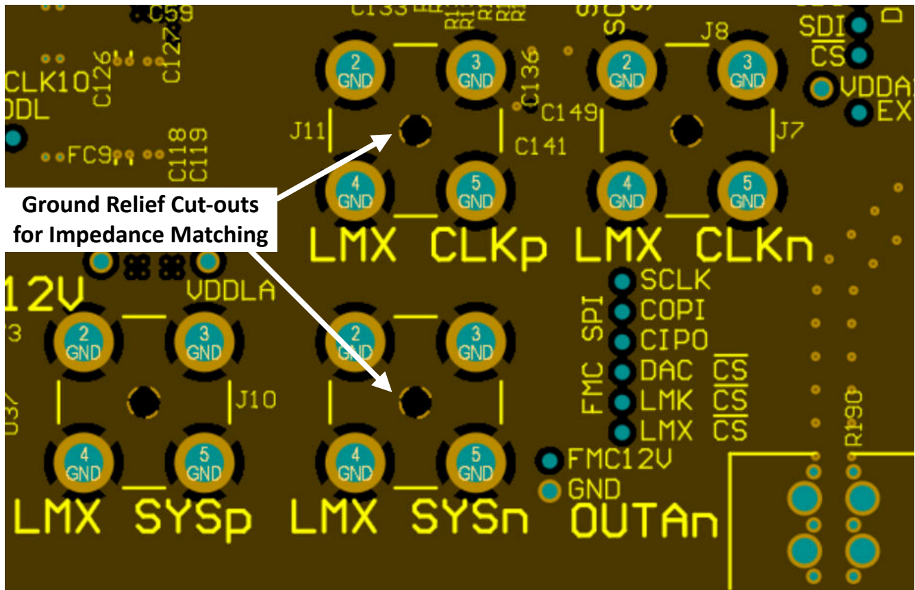
图 8-26. SMA 连接器中心引脚下方的接地开孔
