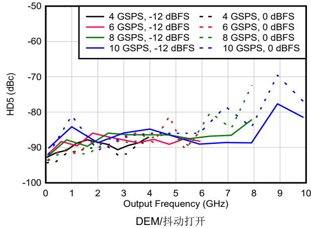
图 6-204. NRZ/RF 模式下 HD5 与频率和采样速率间的关系
