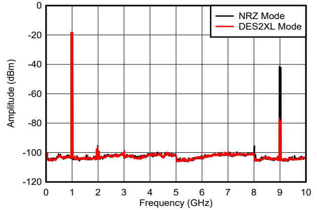
图 6-44. 双音， f_{\text{OUT}} = 997\text{MHz} ，-6dBFS
