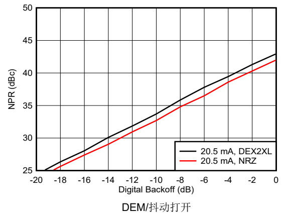
图 6-213. 噪声功率比与数字退避间的关系：第二奈奎斯特区域
