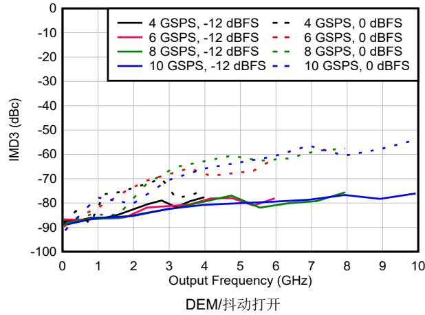
图 6-144. NRZ/RF 模式下 IMD3 与频率和采样速率间的关系
