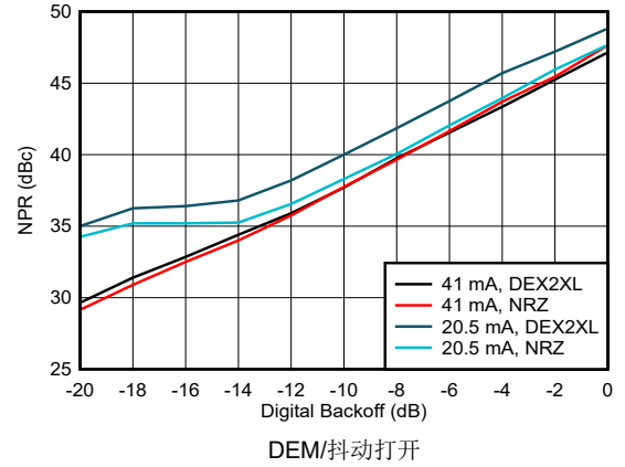
图 6-211. 噪声功率比与数字退避间的关系：第一奈奎斯特区域
