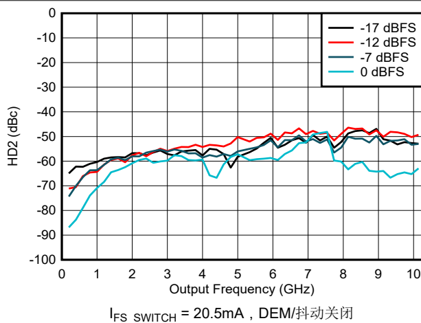
图 6-160. NRZ/RF 模式下 HD2 与频率和数字振幅间的关系
