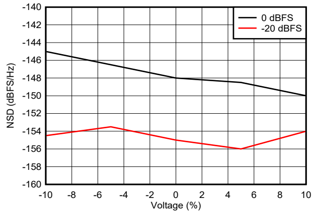
图 6-86. NSD 与电源电压间的关系
