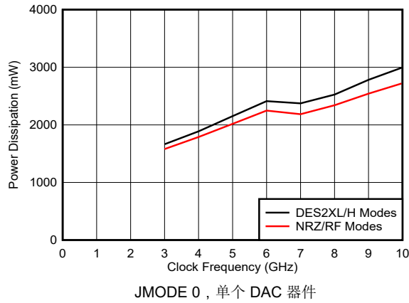
图 6-91. 功率损耗与时钟频率和 DAC 模式间的关系
