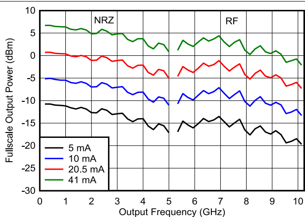
图 6-9. 输出功率与频率间的关系 (NRZ/RF 模式)
