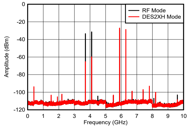
图 6-52. 双音， f_{\text{OUT}} = 6097\text{MHz} ，0dBFS
