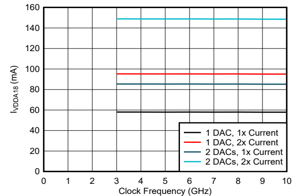
图 6-94. VDDA18 电流与时钟频率和 DAC 模式间的关系
