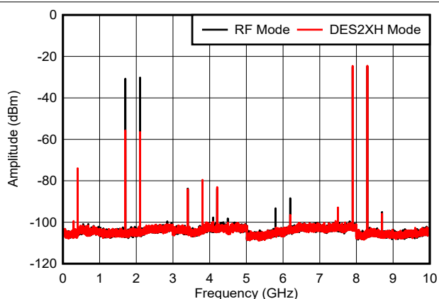
图 6-56. 双音， f_{\text{OUT}} = 8097\text{MHz} ，-6dBFS
