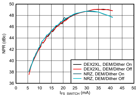
图 6-214. 电源抑制比与输出电流间的关系：第一奈奎斯特区域
