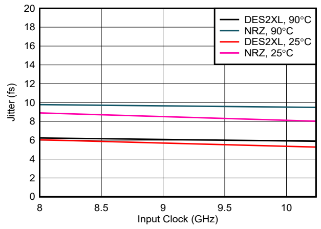
图 6-221. 抖动与输入时钟间的关系
