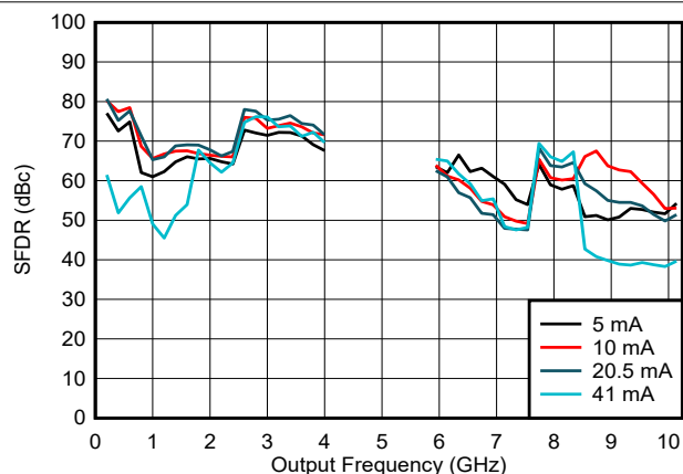
图 6-115. DES2X 模式下 SFDR 与频率和输出电流间的关系
