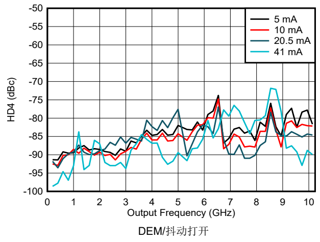
图 6-189. NRZ/RF 模式下 HD4 与频率和输出电流间的关系
