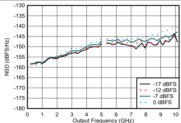
图 6-65. NSD 与输出频率和数字振幅间的关系
