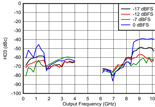
图 6-180. DES2X 模式下 HD3 与频率和数字振幅间的关系
