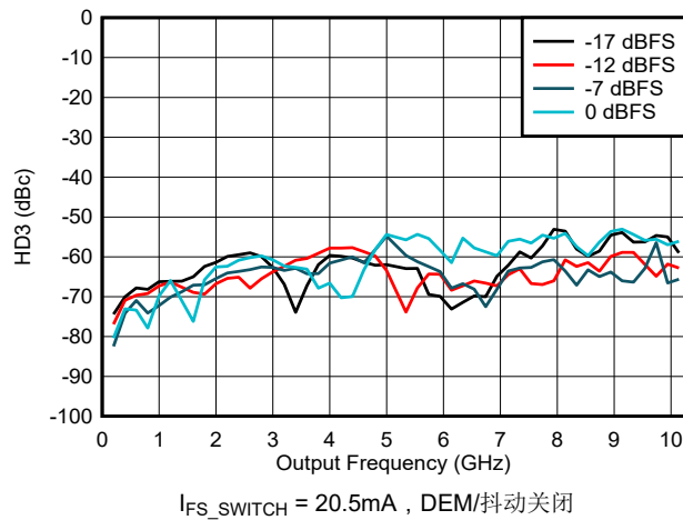
图 6-176. NRZ/RF 模式下 HD3 与频率和数字振幅间的关系
