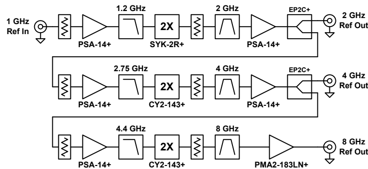
图 8-10. 基准乘法器链
