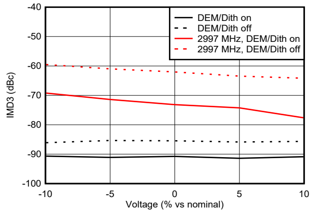
图 6-152. NRZ 模式下 IMD3 与电压间的关系
