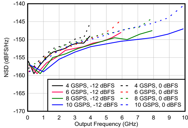
图 6-80. NSD 与输出频率和采样速率间的关系
