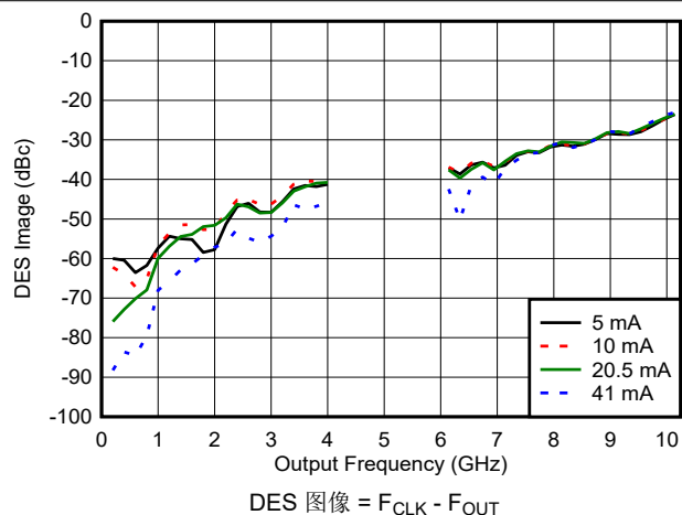
图 6-208. DES2X 模式下 DES 图像与频率和输出电流间的关系
