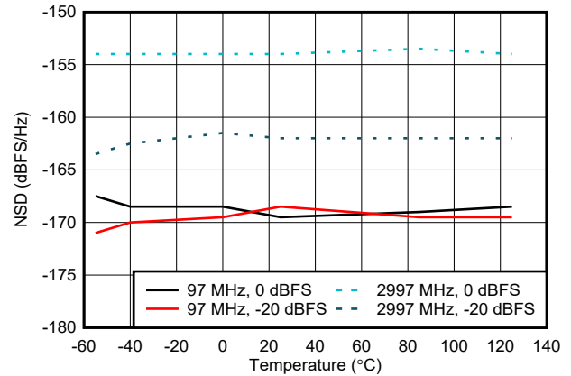
图 6-83. NSD 与温度间的关系
