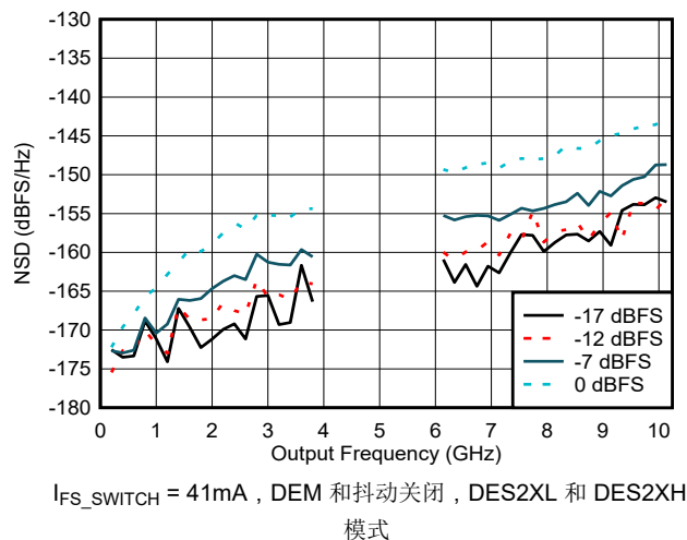
图 6-72. NSD 与输出频率和数字振幅间的关系
