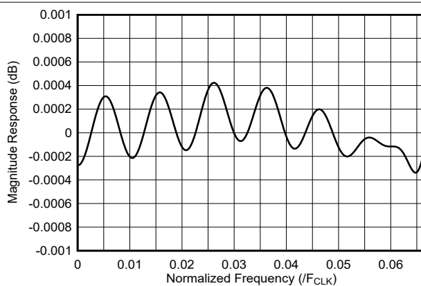
图 7-21. 6 倍内插滤波器通带响应
