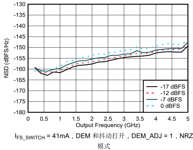
图 6-70. NSD 与输出频率和数字振幅间的关系
