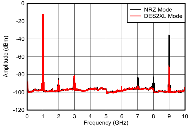
图 6-43. 双音， f_{\text{OUT}} = 997\text{MHz} ，0dBFS
