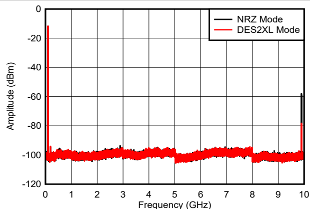
图 6-37. 双音， f_{\text{OUT}} = 97\text{MHz} ， 0\text{dBFS} ( 0 - f_{\text{CLK}} )
