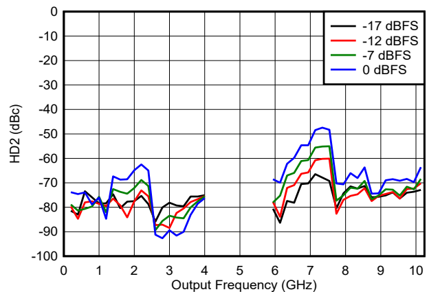
图 6-165. DES2X 模式下 HD2 与频率和数字振幅间的关系
