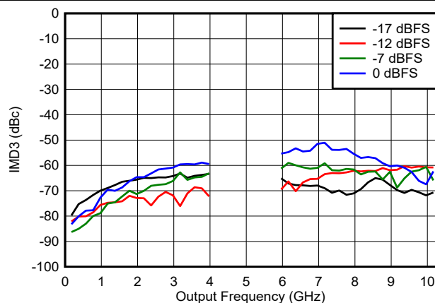
图 6-134. NRZ/RF 模式下 IMD3 与频率和数字振幅间的关系
