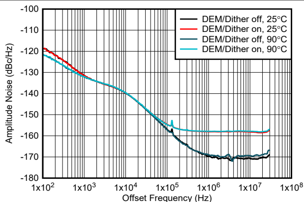
图 6-225. 1GHz 条件下振幅噪声与偏移频率和温度间的关系
