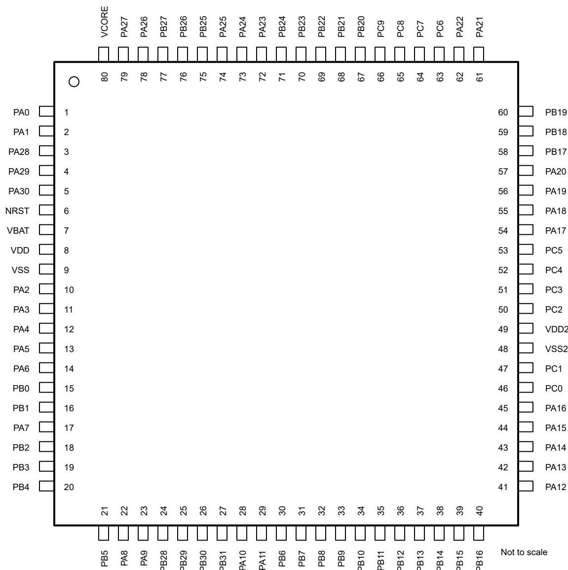
图 6-1. 80 引脚 PNA (0.4mm) 和 PN (0.5mm) (LQFP) 封装
