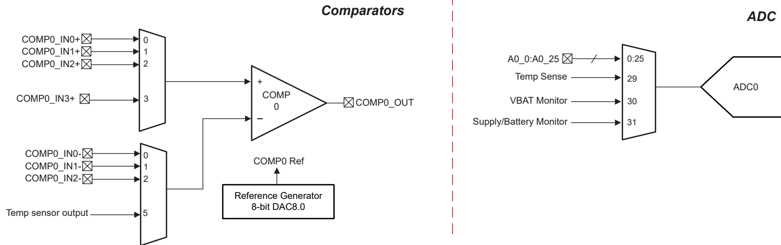
图 8-1. 器件模拟连接
