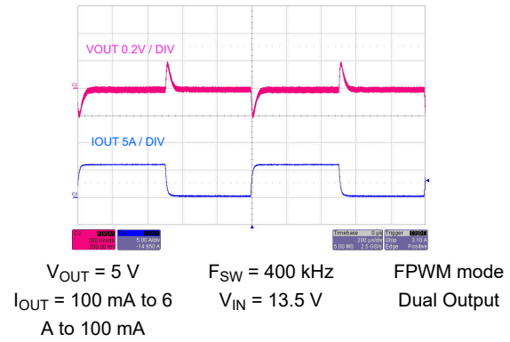
图 9-46. Load Transient
