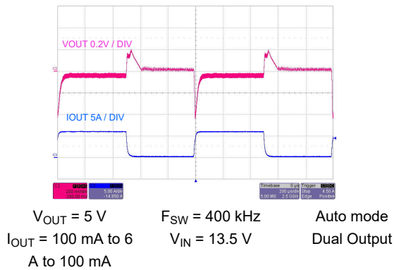
图 9-47. Load Transient
