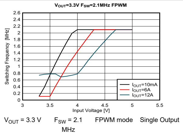
图 9-36. Dropout
