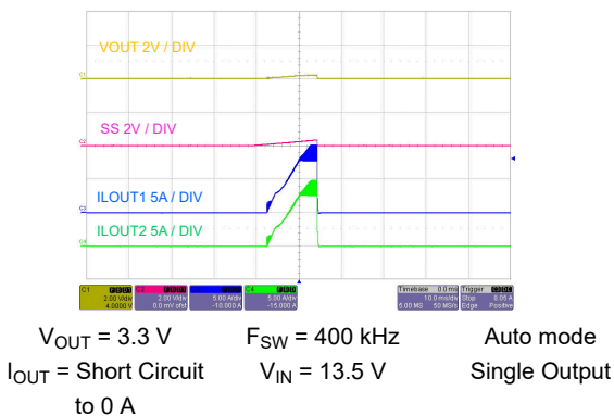
图 9-43. Short-Circuit Hiccup
