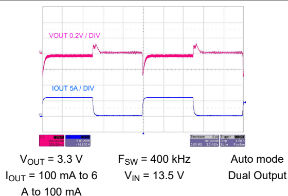
图 9-53. Load Transient
