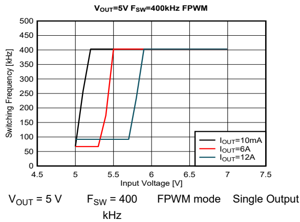
图 9-33. Dropout
