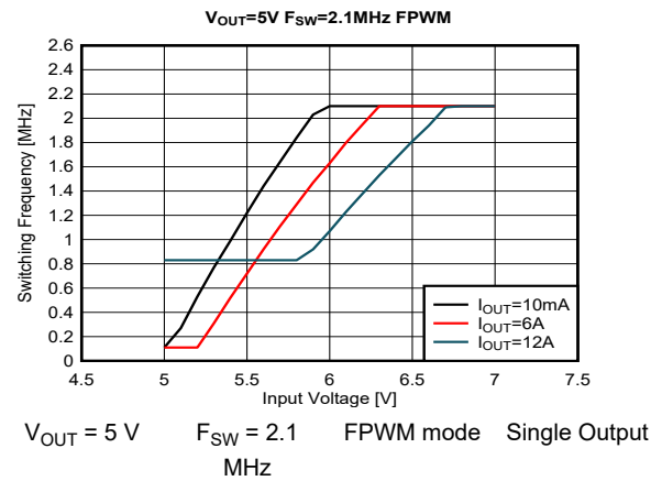
图 9-34. Dropout
