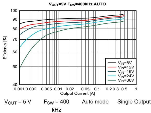
图 9-9. Efficiency
