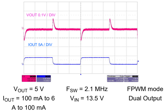
图 9-45. Load Transient
