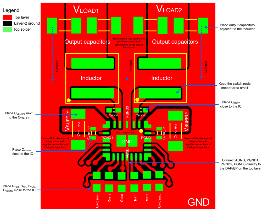
图 9-71. Layout Example
