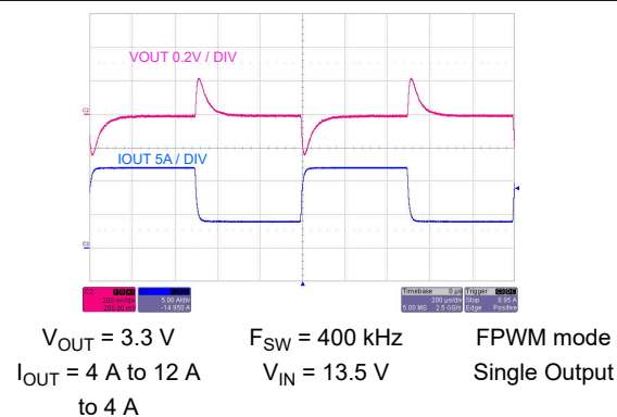
图 9-55. Load Transient
