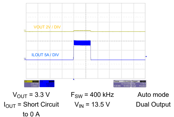
图 9-44. Short-Circuit Hiccup
