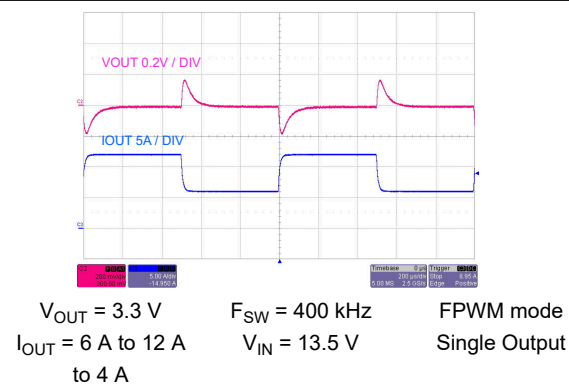
图 9-56. Load Transient
