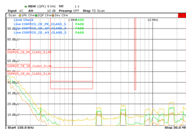
CISPR 25 传导发射， V_{OUT} = 3.3V ，2.1MHz，12A
