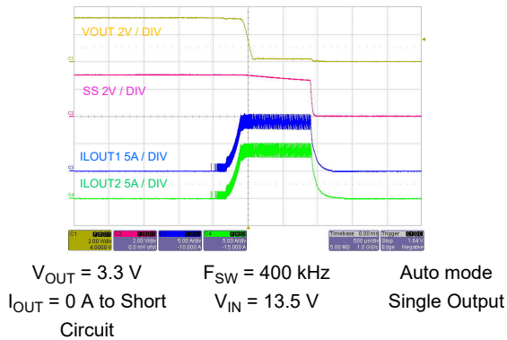
图 9-41. Short-Circuit Protection
