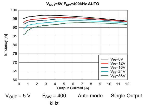
图 9-10. Efficiency
