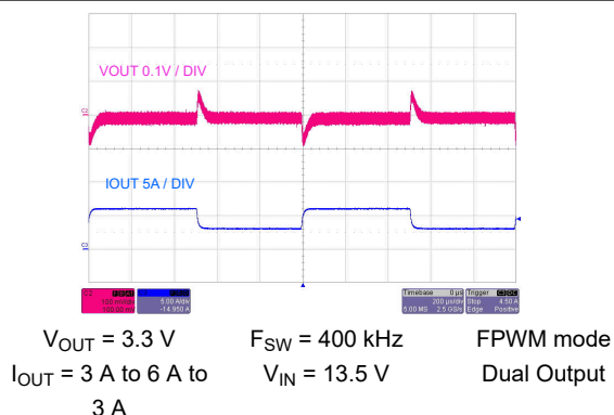
图 9-54. Load Transient
