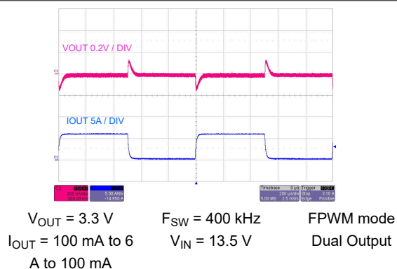
图 9-52. Load Transient
