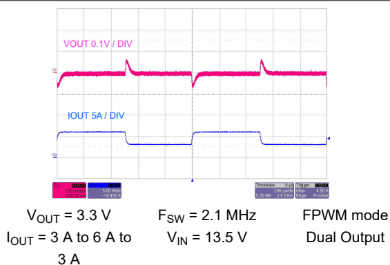
图 9-51. Load Transient
