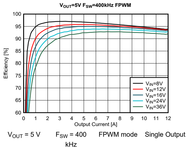
图 9-11. Efficiency
