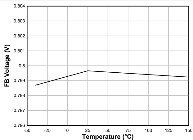
图 7-1. Feedback Voltage
