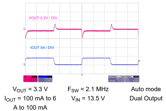
图 9-50. Load Transient
