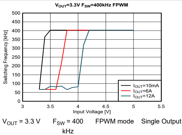
图 9-35. Dropout
