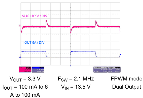
图 9-49. Load Transient
