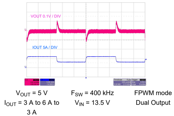
图 9-48. Load Transient
