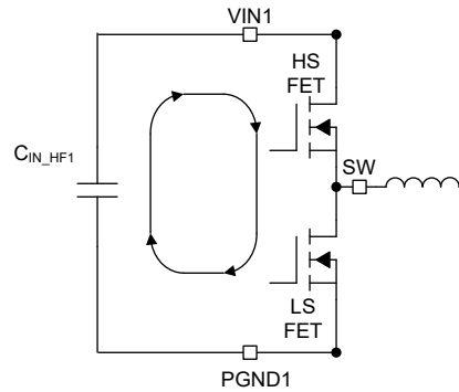
图 9-70. Input Current Loop
