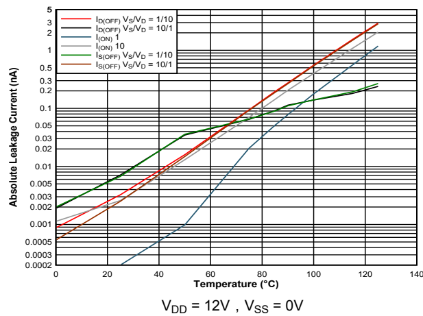
图 5-11. 漏电流与温度间的关系
