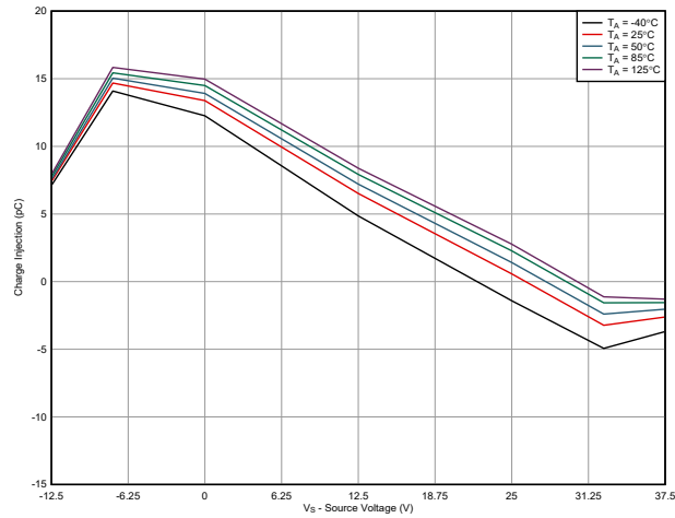
图 5-21. 电荷注入与源极电压间的关系
