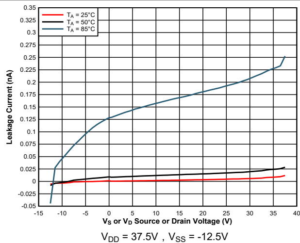
图 5-19. 导通漏电流与源极或漏极电压间的关系
