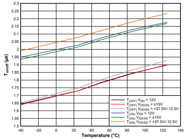
图 5-22. 导通/关断时间与温度间的关系
