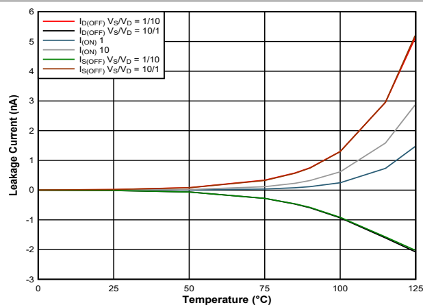
图 5-13. 漏电流与温度间的关系
