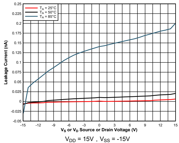
图 5-18. 导通漏电流与源极或漏极电压间的关系
