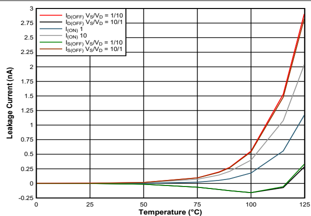
图 5-14. 漏电流与温度间的关系
