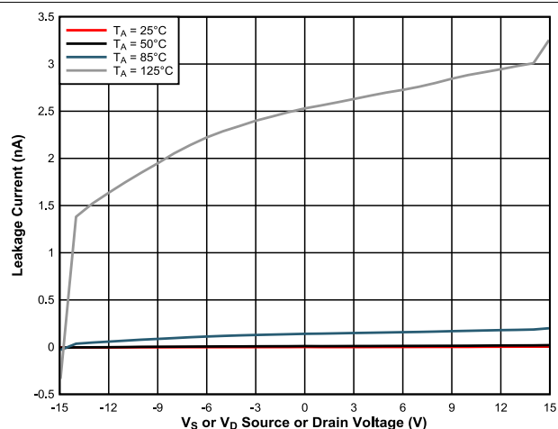
图 5-16. 导通漏电流与源极或漏极电压间的关系
