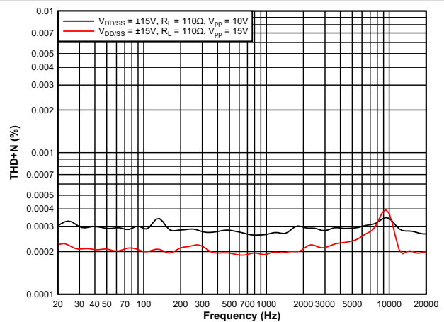
图 5-26. THD+N 与频率间的关系
