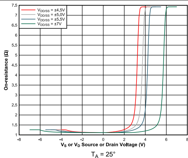
图 5-3. 导通电阻与源极或漏极电压之间的关系
