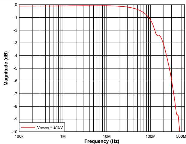
图 5-25. 带宽与频率间的关系
