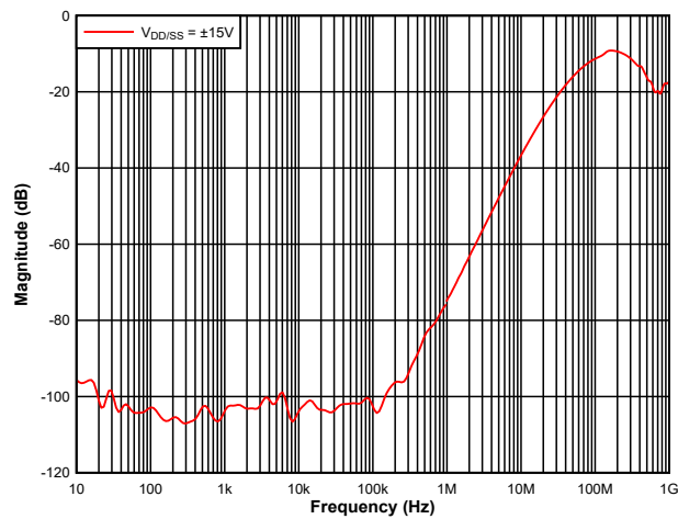
图 5-23. 关断隔离与频率间的关系
