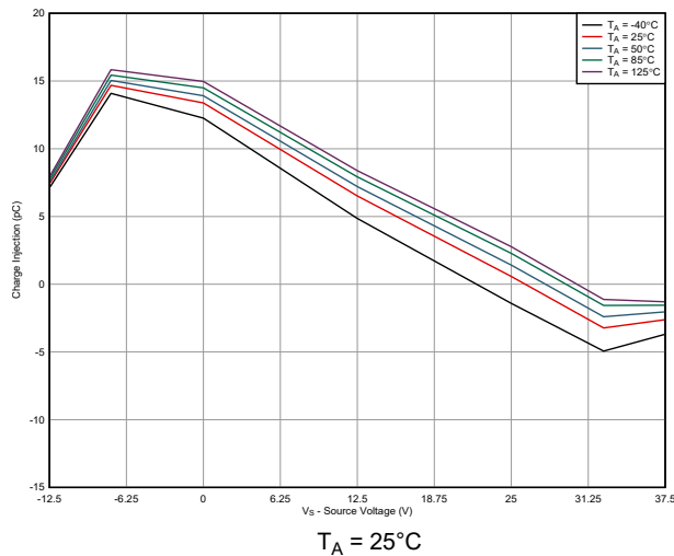
图 8-2. 电荷注入与源极电压间的关系
