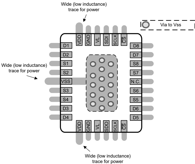
图 8-5. TMUXS7614D 布局示例
