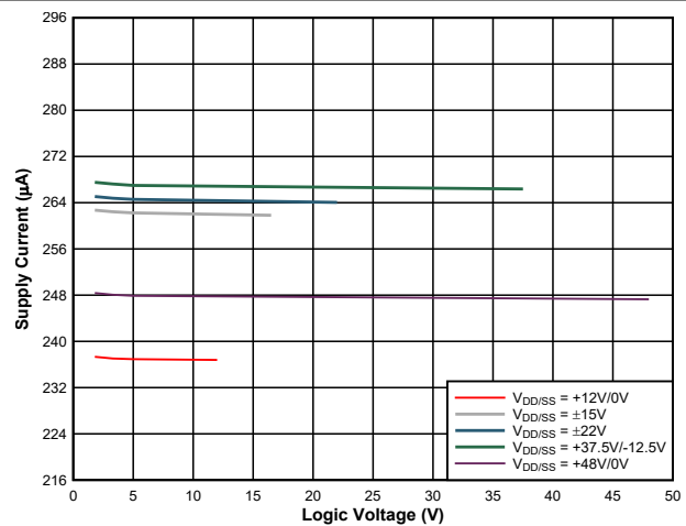
图 5-20. 电源电流与逻辑电压间的关系
