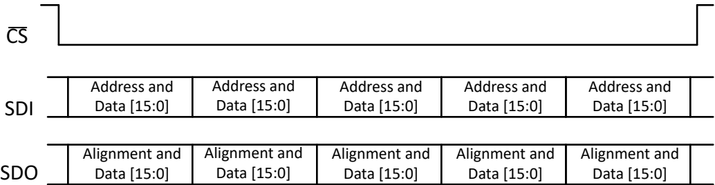
图 7-3. SPI 突发模式示例
