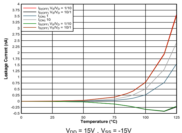
图 5-12. 漏电流与温度间的关系
