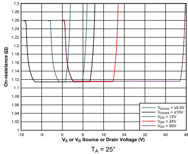
图 5-7. 导通电阻与源极或漏极电压之间的关系
