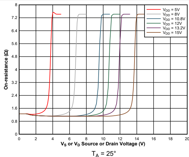
图 5-5. 导通电阻与源极或漏极电压之间的关系
