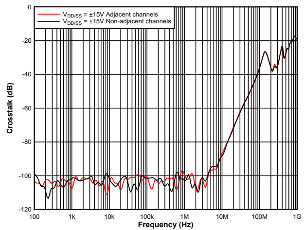
图 5-24. 串扰与频率间的关系
