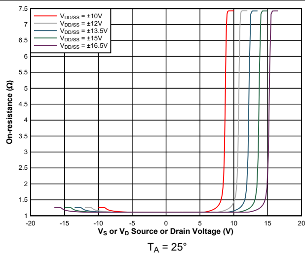
图 5-4. 导通电阻与源极或漏极电压之间的关系
