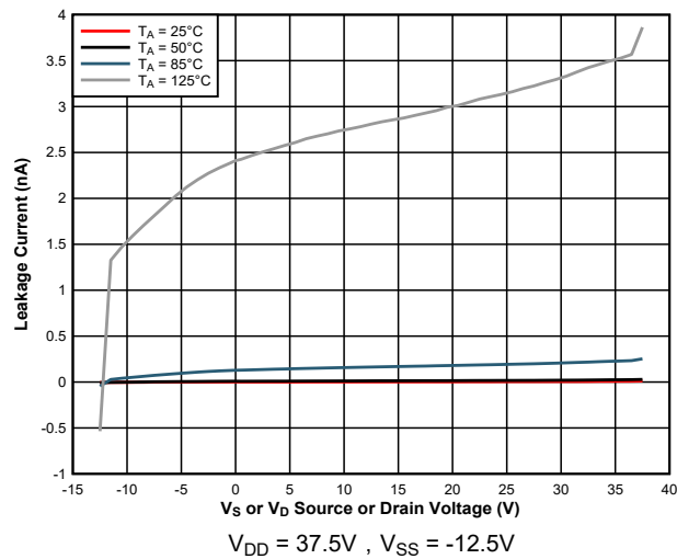
图 5-17. 导通漏电流与源极或漏极电压间的关系
