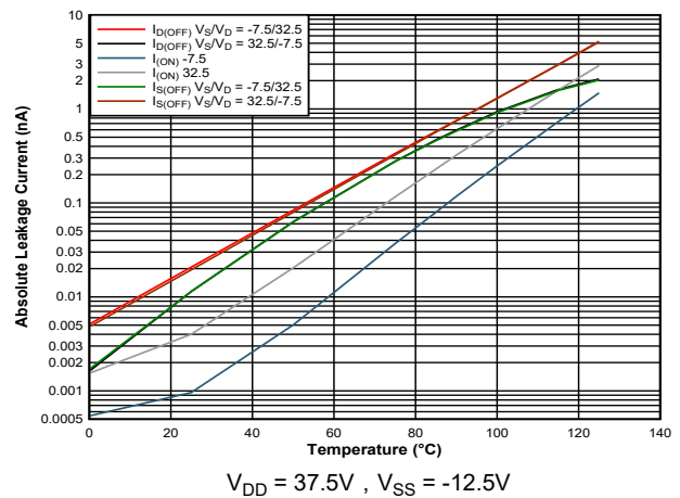
图 5-10. 漏电流与温度间的关系
