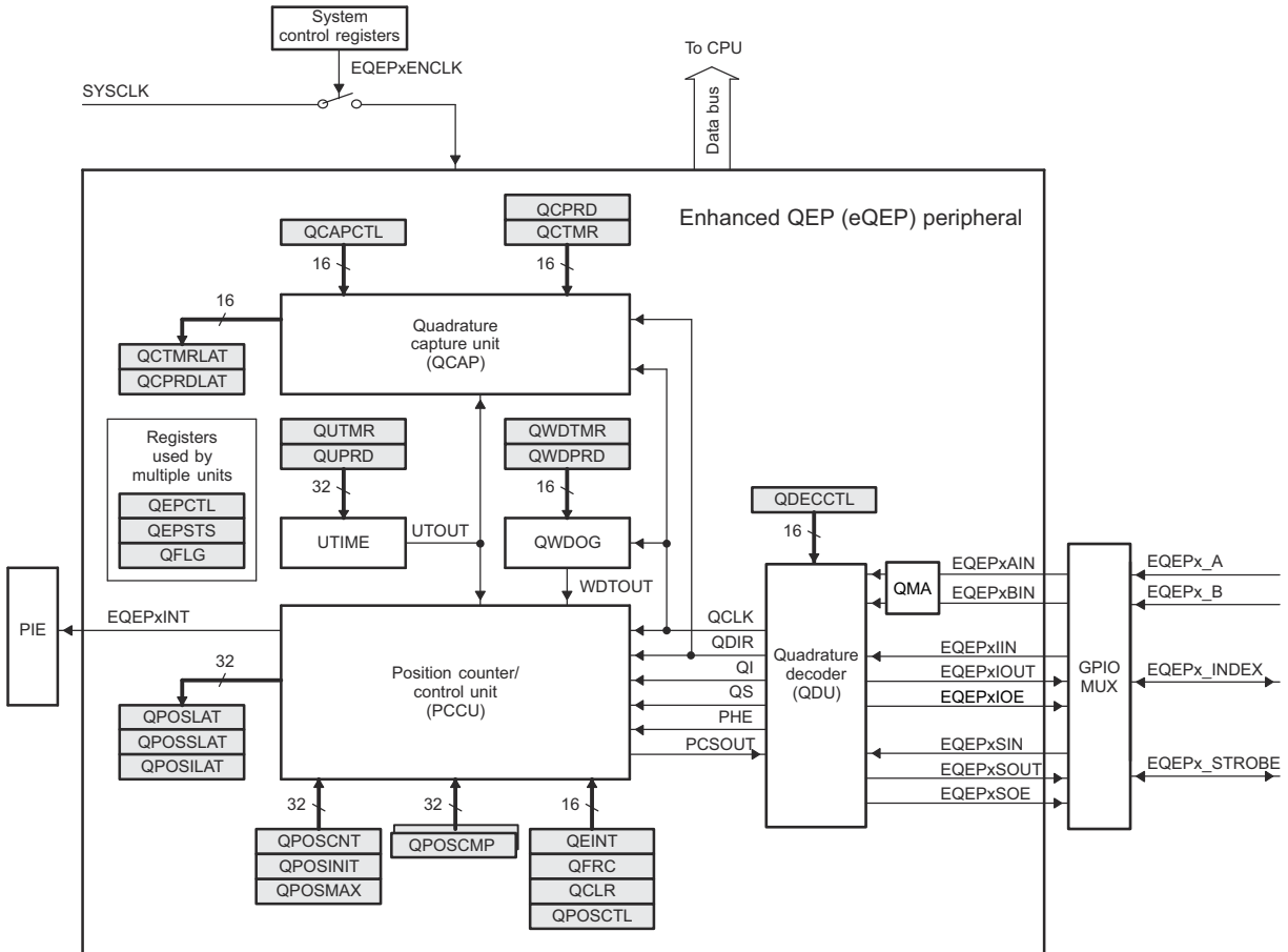
图 6-62. eQEP 方框图
