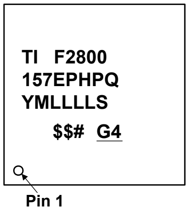
图 9-8. PHP 封装的封装编号法 ( 通过 AEC-Q100 0 级认证 )
