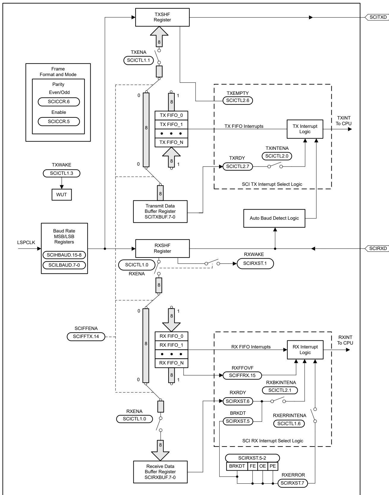
图 6-68. SCI 方框图
