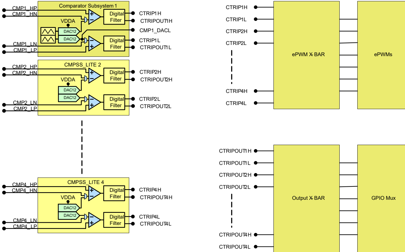
图 6-45. CMPSS 连接
