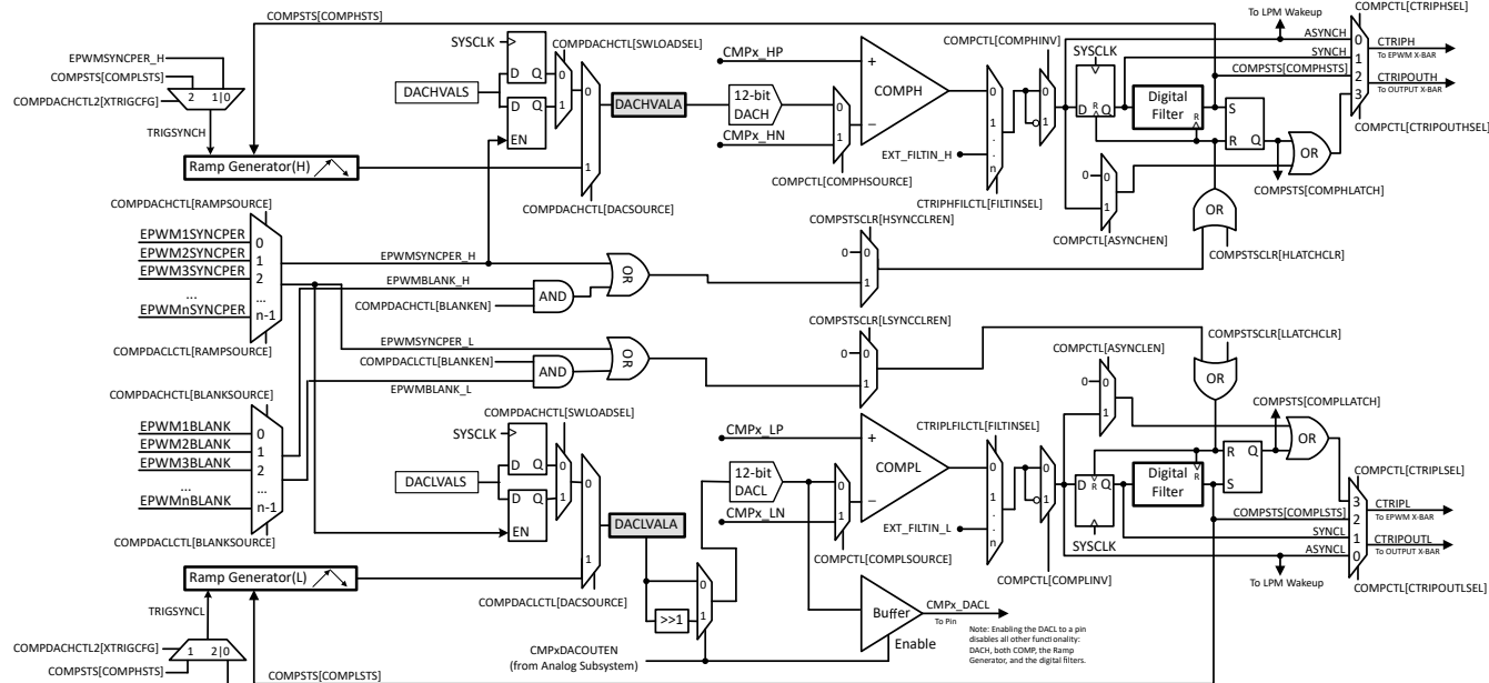
图 6-46. CMPSS 模块方框图
