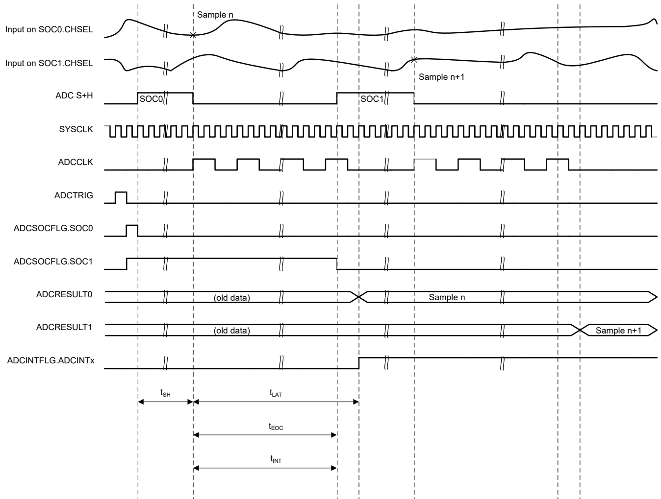
图 6-44. ADC 时序
