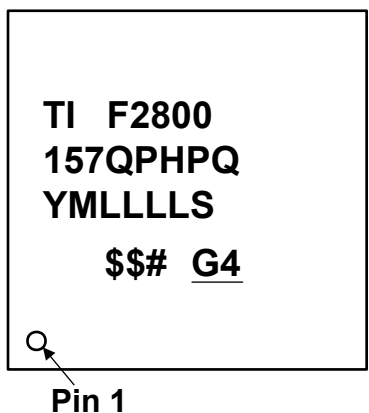
图 9-7. PHP 封装的封装编号法 ( 通过 AEC-Q100 1 级认证 )
