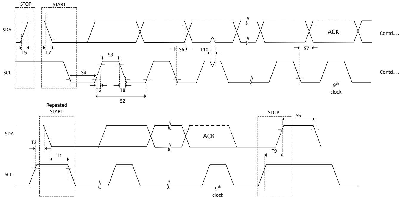
图 6-66. I2C 时序图
