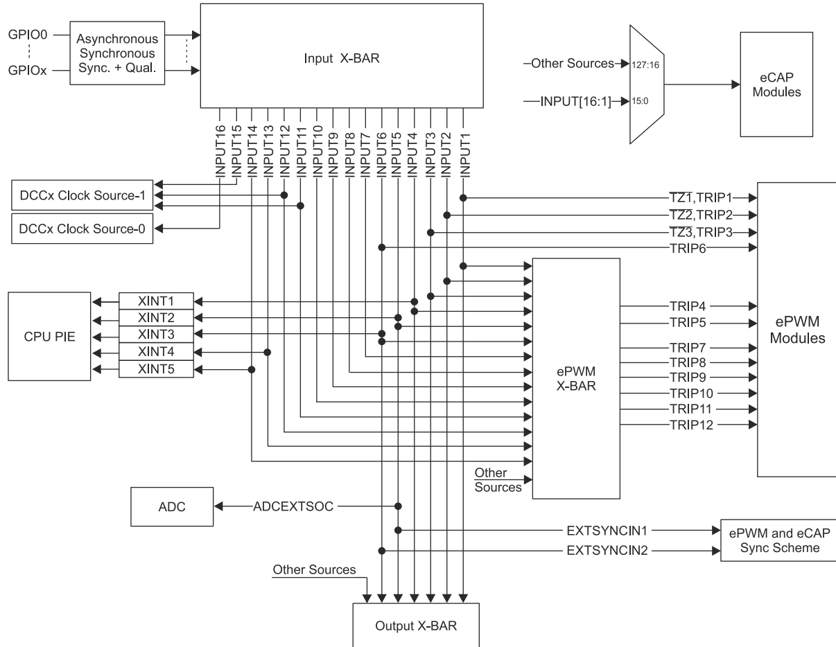
图 5-5. 输入 X-BAR
