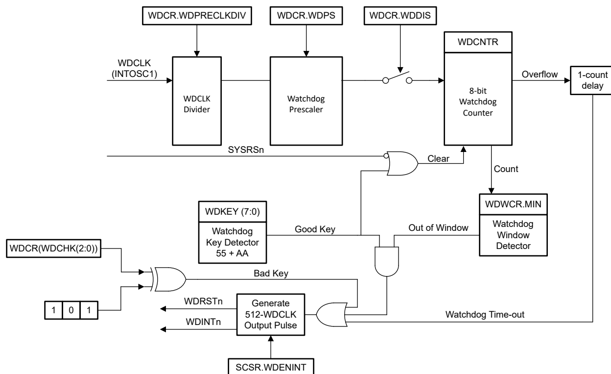
图 7-3. 窗口看门狗
