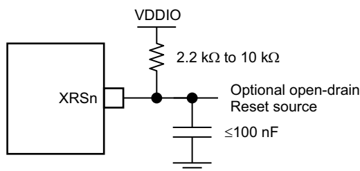
图 6-8. 复位电路
