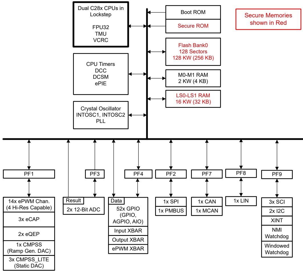
图 7-1. 功能方框图
