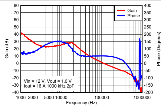
图 7-7. 波特图
