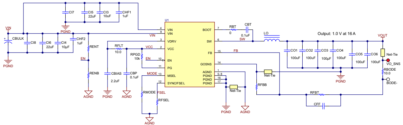
图 7-1. 12V 输入，1.0V 输出，1MHz 原理图
