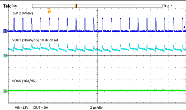
图 7-16. 输出纹波 - 空载
