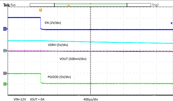
图 7-11. EN 关断
