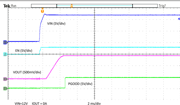
图 7-14. VIN 启动
