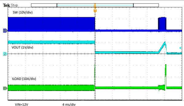
图 7-22. 过流保护 - 断续和恢复
