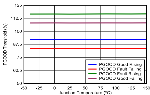
图 5-9. PG 阈值
