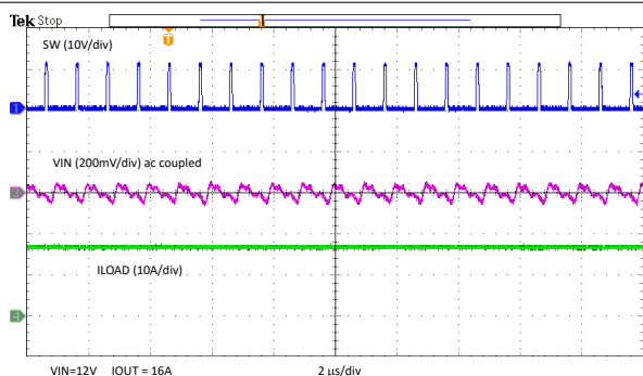
图 7-19. 输入纹波 - 满载
