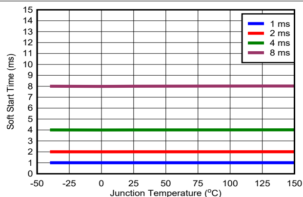
图 5-12. 软启动
