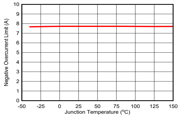
图 5-4. 负过流限制
