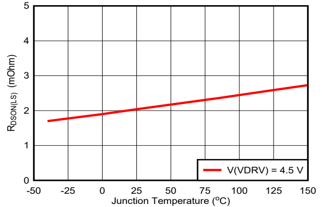
图 5-2. 低侧 FET R_{ds(on)}
