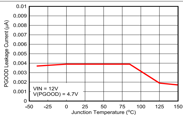
图 5-10. PG 漏电流
