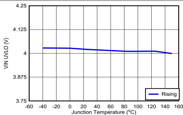
图 5-7. V_{IN} UVLO
