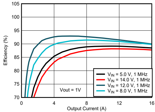
图 7-4. 效率曲线
