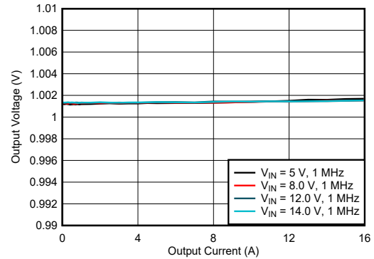
图 7-5. 负载调节
