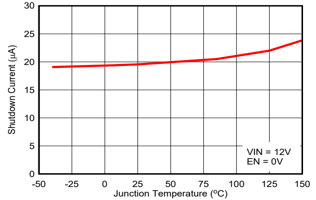
图 5-14. 关断电源电流
