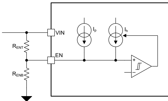
图 6-2. 使用 EN 引脚实现可调 UVLO
