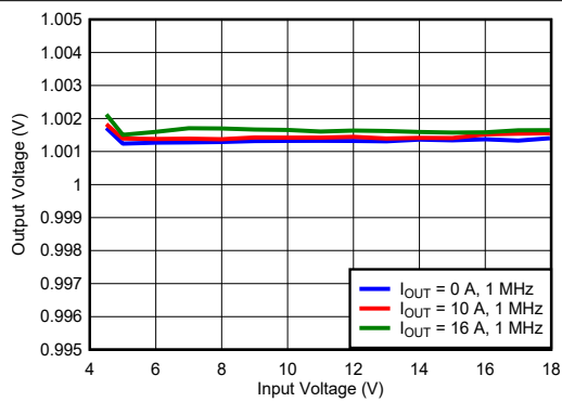
图 7-6. 线性调整率
