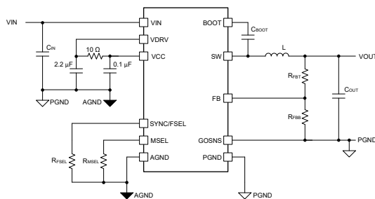
TPS543A26T 简化版应用
