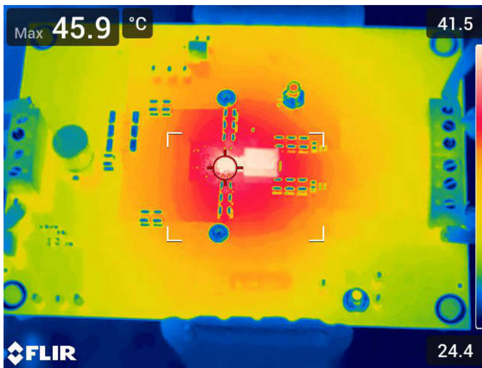
图 7-24. 25^\circ\text{C} 环境温度下的热图像
