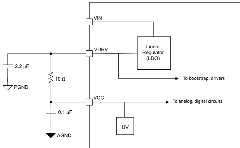
图 6-1. 器件旁路
