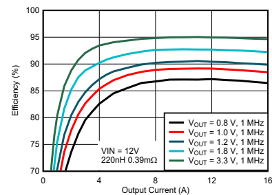
典型应用效率
