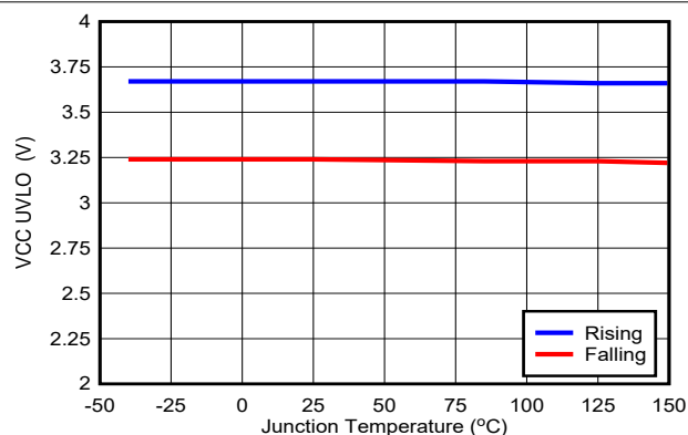
图 5-8. V_{CC} UVLO
