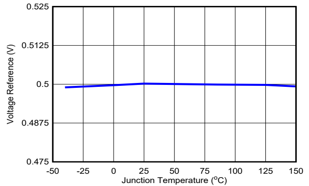
图 5-6. V_{REF}
