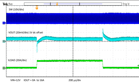
图 7-8. 负载瞬态
