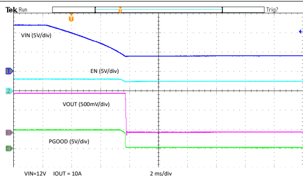
图 7-15. VIN 关断
