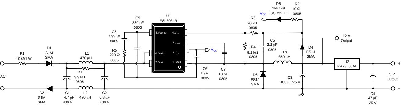
图 31. 原理图
