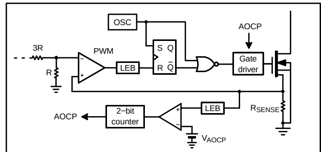
图 23. AOCP 电路
