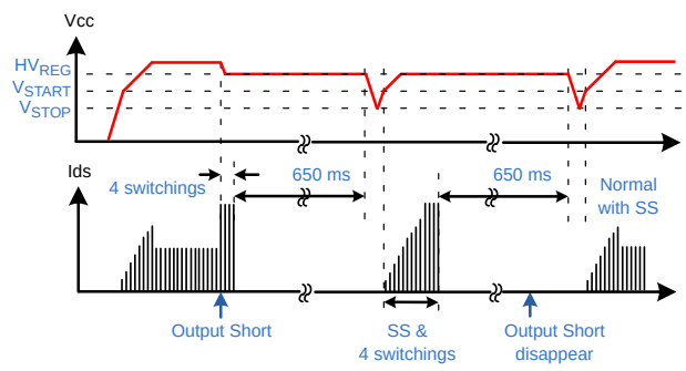
图 24. AOCP 波形
