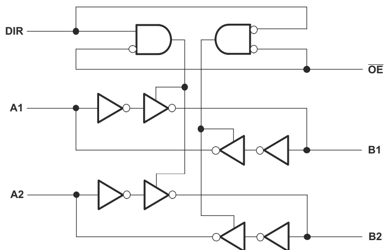
SN74AVC4T774-Q1 半侧逻辑图 (正逻辑)
