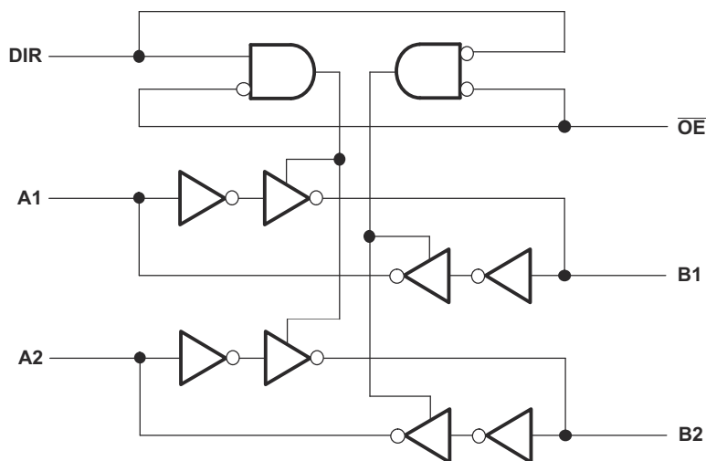
图 7-1. SN74AVC4T774-Q1 半侧逻辑图 (正逻辑)
