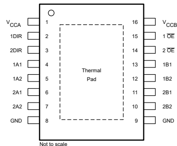
图 4-2. DYY 封装，16 引脚 SOT (顶视图)
