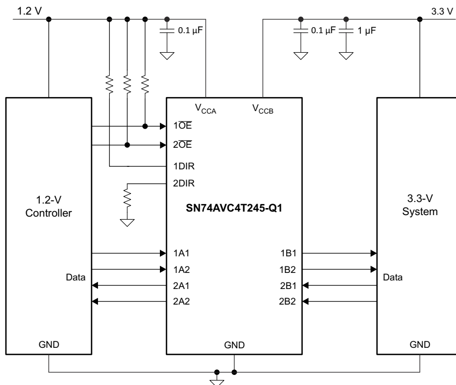
图 8-1. 典型应用图
