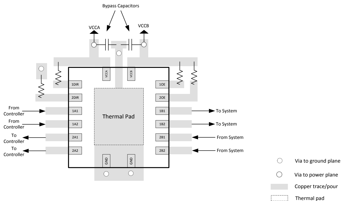
图 8-3. SN74AVC4T774-Q1 RGY 封装布局图
