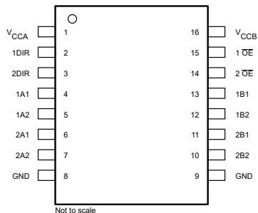
图 4-1. PW 封装，16 引脚 TSSOP (顶视图)
