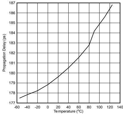
图 5-18. 传播延迟
