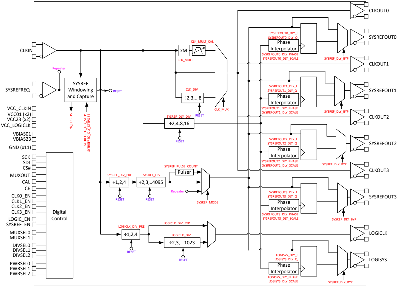
图 6-1. 功能方框图
