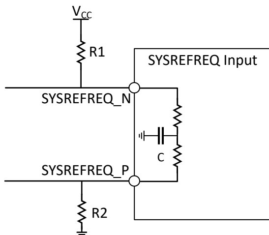
图 6-6. SYSREFREQ 引脚逻辑低电平设置
