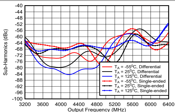
图 5-12. X2 模式下的倍频器 1/2 次谐波
