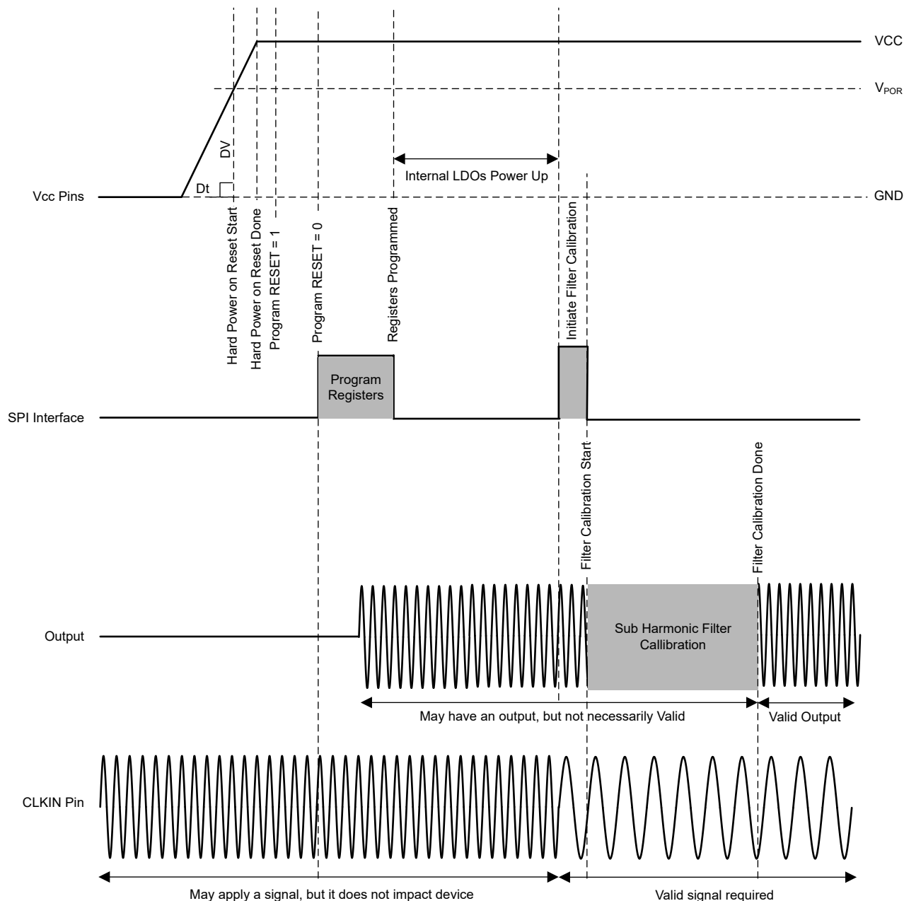
图 7-11. 上电时序
