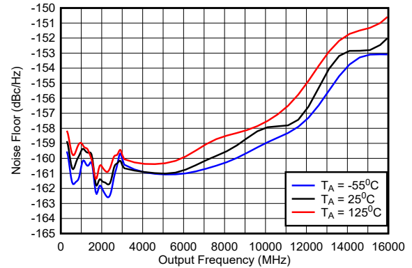
图 5-7. 缓冲器模式下的本底噪声
