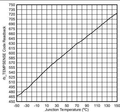
图 5-17. 温度传感器回读
