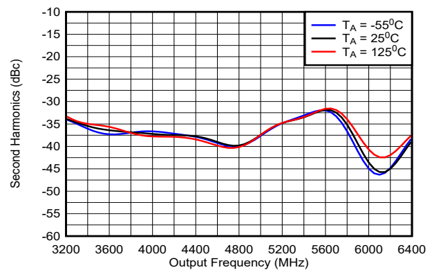
图 5-11. 倍频 X2 模式下的二次谐波 (差分输出)
