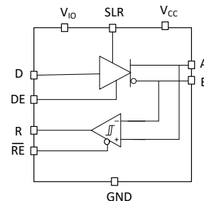
THVD2410V-EP 和 THVD2450V-EP 简化原理图
