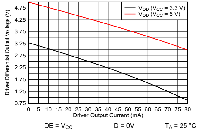
图 5-2. 驱动器差分输出电压与驱动器输出电流的关系
