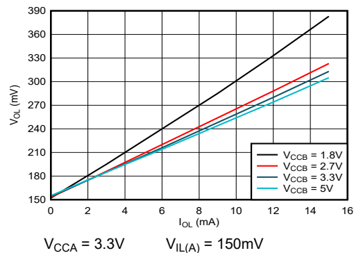
图 5-4. 低电平输出电压 ( V_{OL(Bx)} ) 与低电平电流 ( I_{OL(Bx)} ) 间的关系
