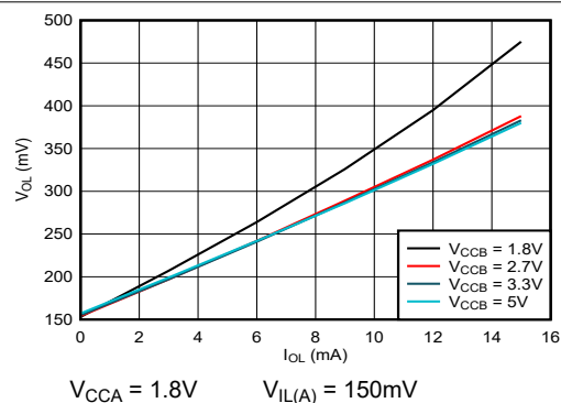
图 5-2. 低电平输出电压 ( V_{OL(Bx)} ) 与低电平电流 ( I_{OL(Bx)} ) 间的关系
