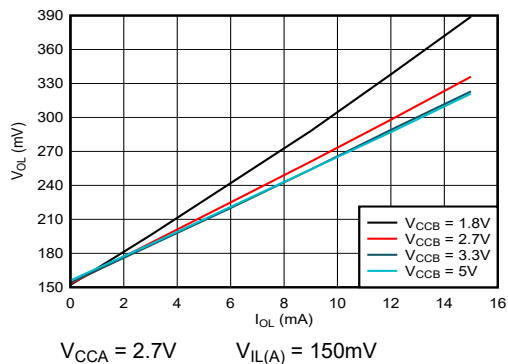
图 5-3. 低电平输出电压 ( V_{OL(Bx)} ) 与低电平电流 ( I_{OL(Bx)} ) 间的关系
