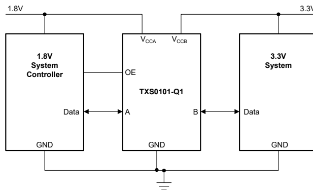
典型工作电路
