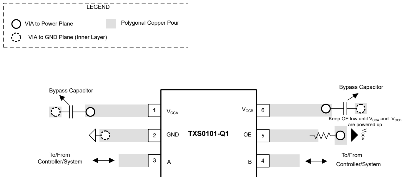
图 8-3. TXS0101-Q1 的典型布局
