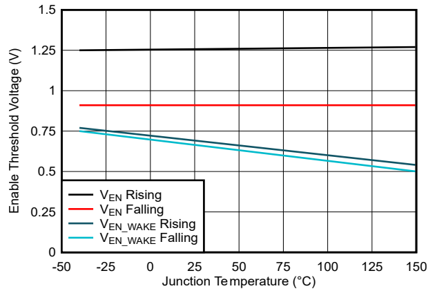
图 6-7. Enable Thresholds
