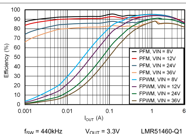
图 6-2. 3.3V 效率与负载电流间的关系
