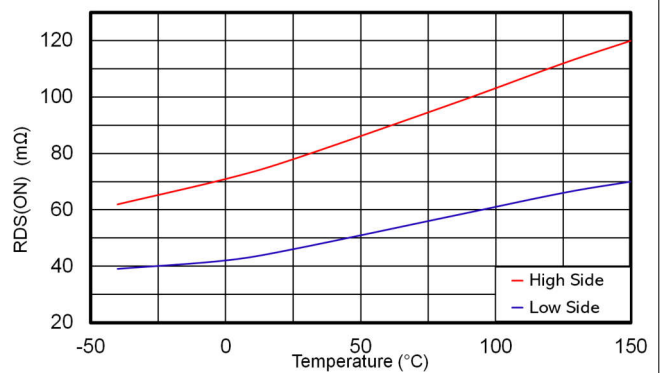
图 6-10. 高侧和低侧开关 R_{DS(on)}
