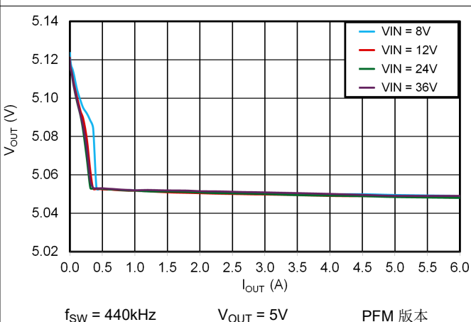
图 6-4. 5V 负载调整
