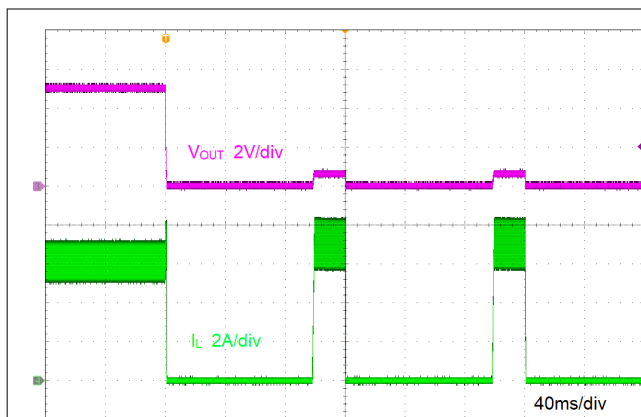
图 8-8. 短路保护
