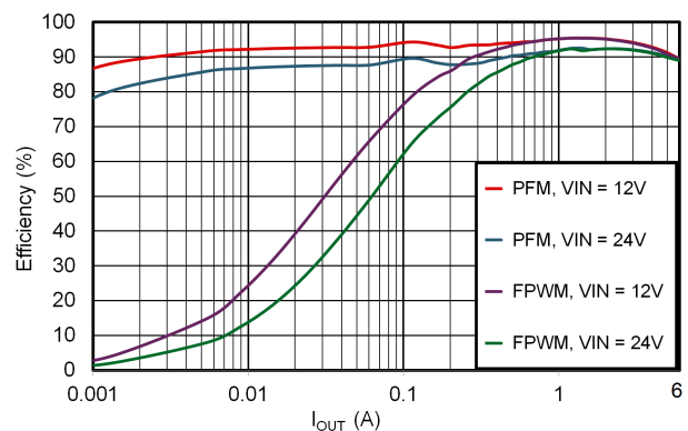
效率与输出电流间的关系 V_{OUT} = 5V , 400kHz
