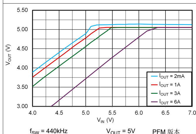
图 6-5. 5V 压降
