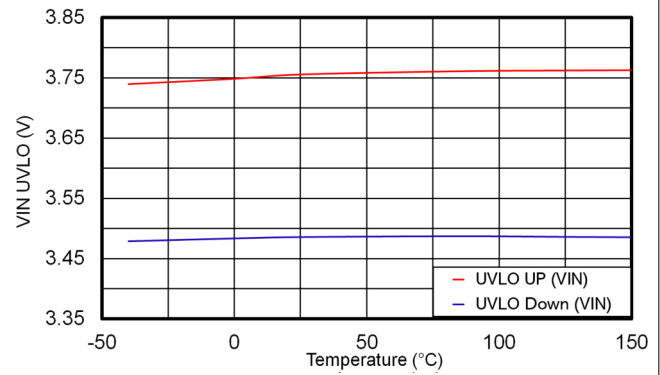
图 6-8. V_{IN} UVLO
