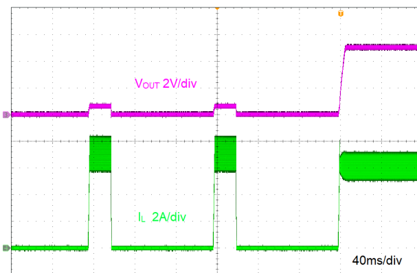
图 8-9. 短路恢复
