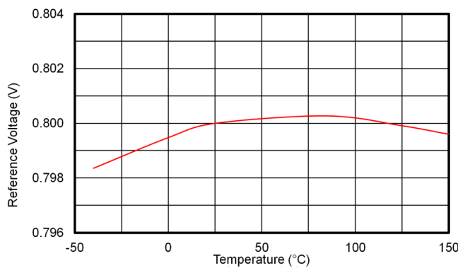
图 6-9. 基准电压
