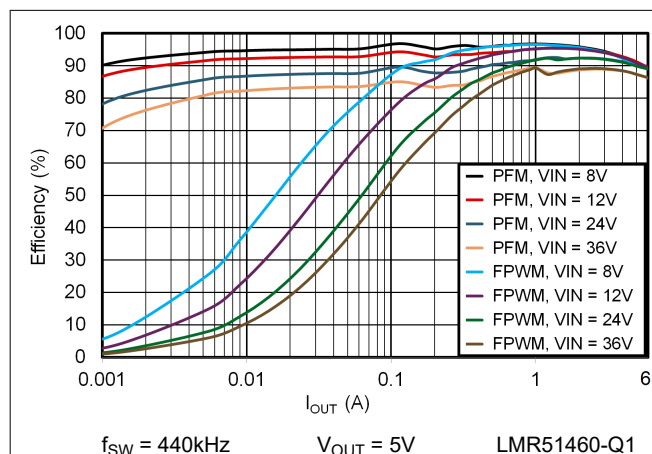
图 6-1. 5V 效率与负载电流间的关系
