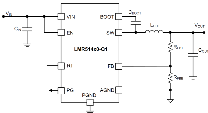
简化原理图
