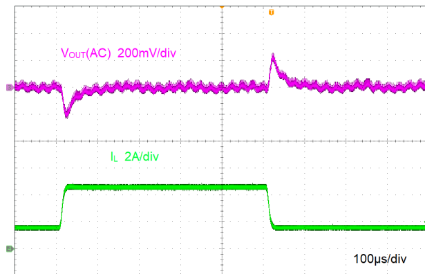
图 8-6. 负载瞬态
