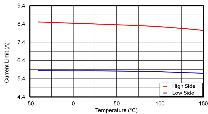
图 6-11. LMR51460-Q1 高侧和低侧电流限值
