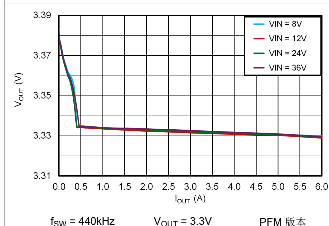
图 6-3. 3.3V 负载调整
