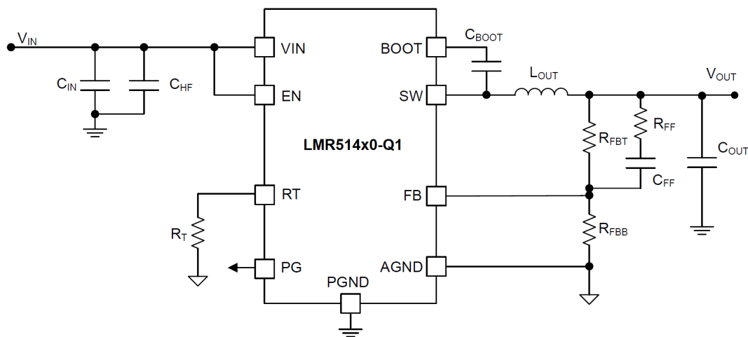
图 8-1. 应用电路
