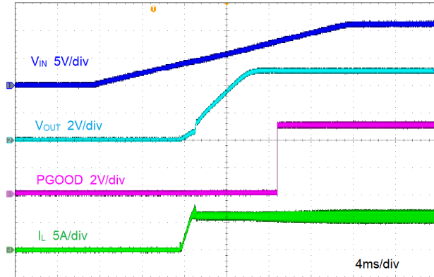
图 8-4. 由 V_{IN} 启动
