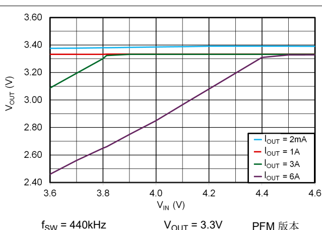
图 6-6. 3.3V 压降
