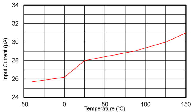
图 6-7. 非开关输入电源电流
