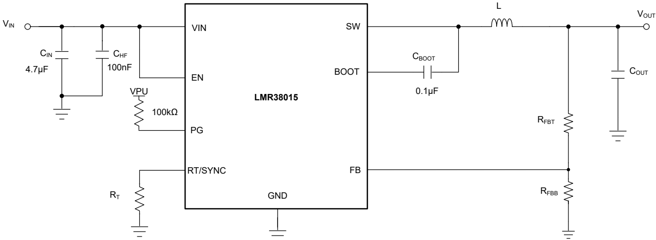
图 8-1. 示例应用电路
