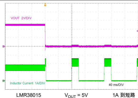
图 8-7. 应用短路
