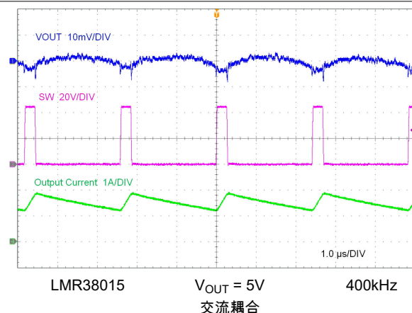
图 8-6. 满载开关
