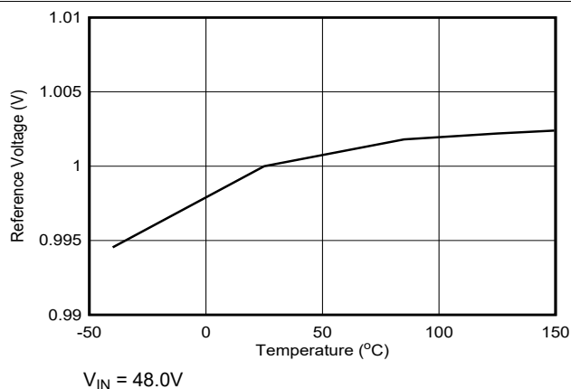
图 6-4. 基准电压与温度间的关系
