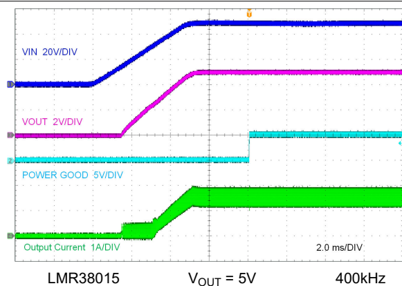
图 8-3. 由 VIN 启动
