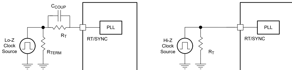
图 7-4. 与外部时钟同步
