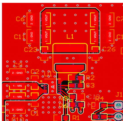
图 8-16. WSON (DRR) 封装的布局示例
