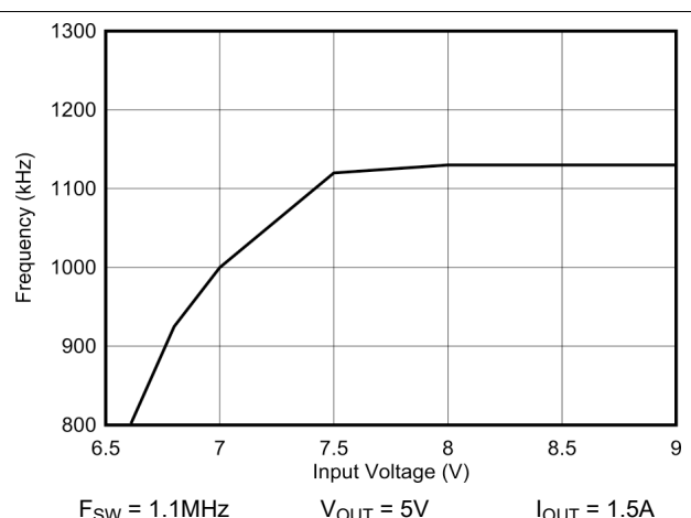
图 7-8. T_{OFF\_MIN} 时的典型频率折返
