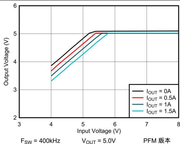
图 6-3. 5V 压降
