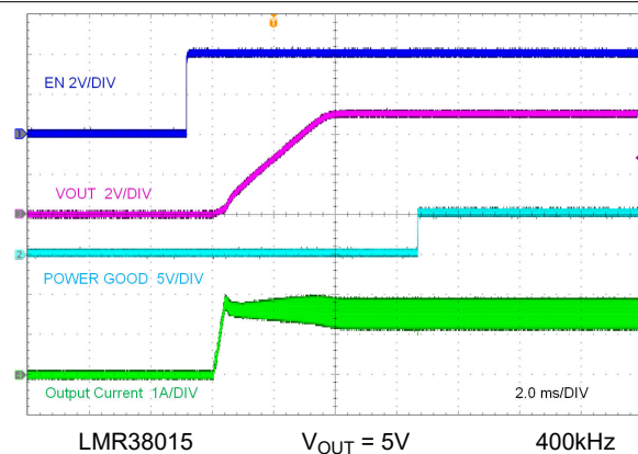
图 8-4. 由 EN 启动
