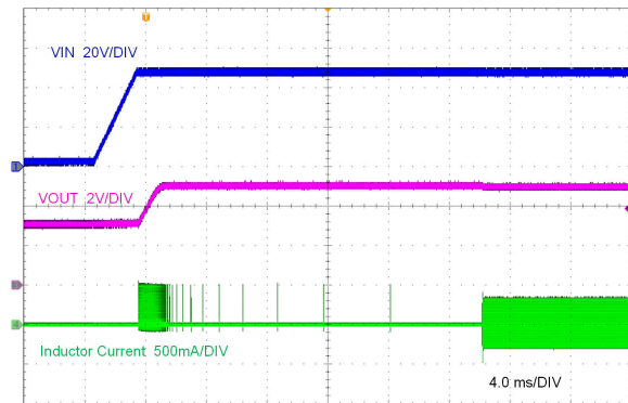
LMR38015 V_{OUT} = 5V 空载 偏置为 3V
