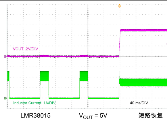
图 8-8. 短路恢复
