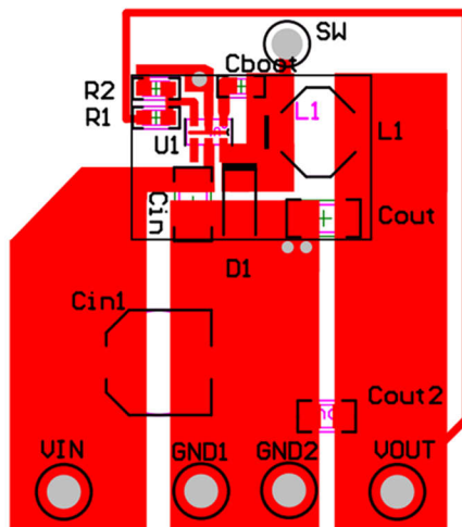
图 8-9. Layout Example
