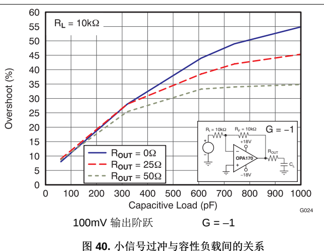
图 40. 小信号过冲与容性负载间的关系
