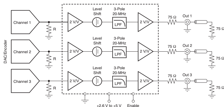
简化的应用电路
