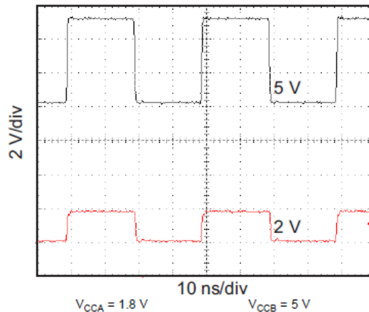
图 8-2. 2.5MHz 信号的电平转换
