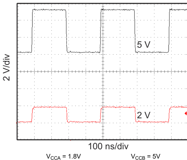
图 8-2. 2.5MHz 信号的电平转换
