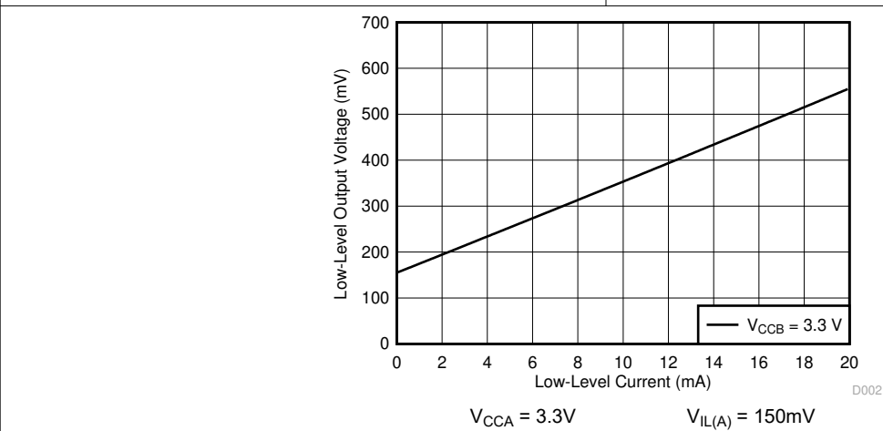
图 5-3. 低电平输出电压 ( V_{OL(Ax)} ) 与低电平电流 ( I_{OL(Ax)} ) 间的关系
