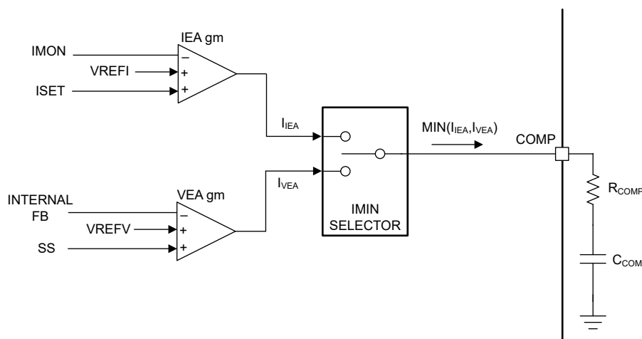
图 6-6. 双环路架构
