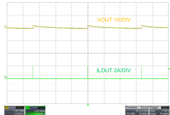
图 7-10. PFM 模式、 V_{SUPPLY} = 48V 、 I_{LOAD} = 0A 条件下的空载运行
