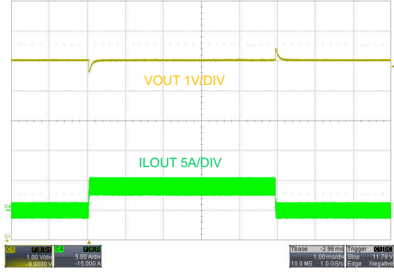
图 7-11. V_{\text{SUPPLY}} = 48\text{V} 、FPWM、从 0A 变为 4A 时的负载瞬态响应
