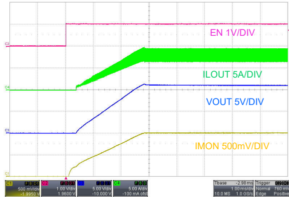
图 7-7. 启动，EN 开启， V_{SUPPLY} = 48V ， I_{LOAD} = 8A 电阻负载
