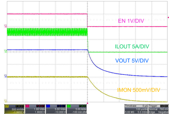
图 7-8. 关断，EN 关闭， V_{SUPPLY} = 48V ， I_{LOAD} = 8A 电阻负载
