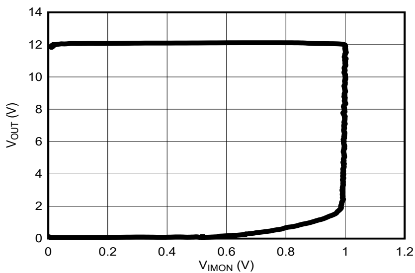
充电瞬态期间的恒流恒压运行
