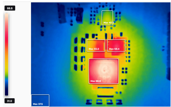
图 7-14. V_{\text{SUPPLY}} = 48\text{V} , I_{\text{LOAD}} = 8\text{A} , T_A = 25^\circ\text{C} , 无气流
