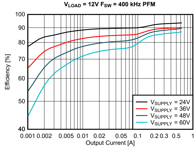
图 7-6. PFM 模式效率，对数标度
