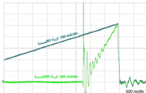
图 30. I_{LIMIT} 波形 (85 V AC 与 460 V AC )
