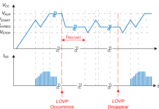
图 25. LOVP 波形
