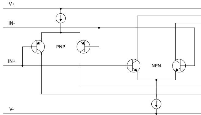
图 6-2. 轨到轨输入级
