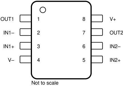
图 4-2. OPA2994-Q1 D 和 DGK 封装， 8 引脚 SOIC 和 VSSOP ( 顶视图 )
