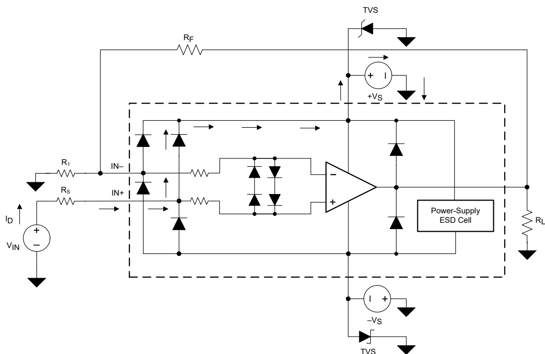
图 6-4. 与典型电路应用相关的等效内部 ESD 电路
