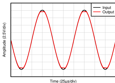
图 6-3. 无相位反转
