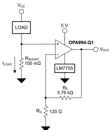
图 7-1. OPAx994-Q1 位于低侧电流检测应用
