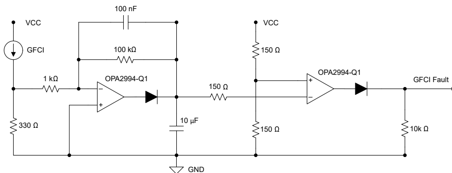
OPAx994-Q1 位于电动汽车服务设备 (EVSE) 接地故障断路器 (GFCI) 故障检测和测试电路中
