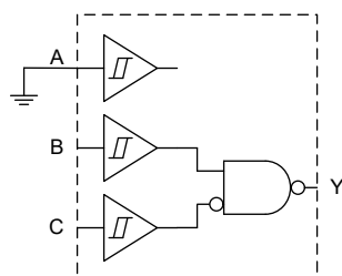
具有 1 个反相输入的双输入与非门
