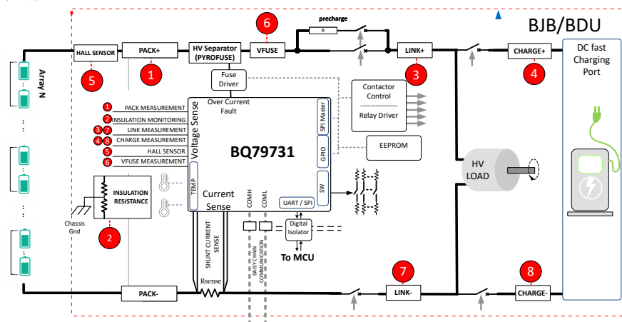
简化版系统图
