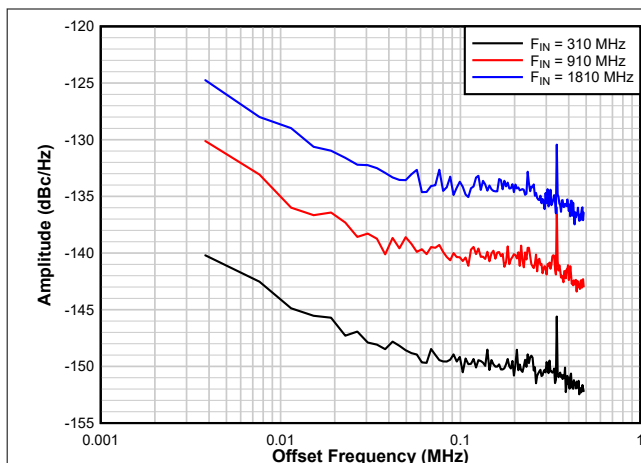
图 7-8. 相位噪声示例
