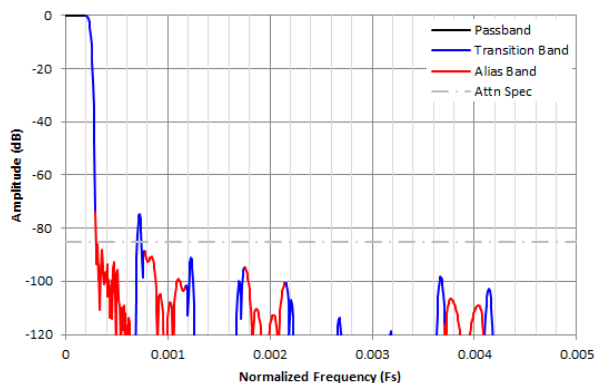
图 7-43. /2048 复数抽取滤波器响应
