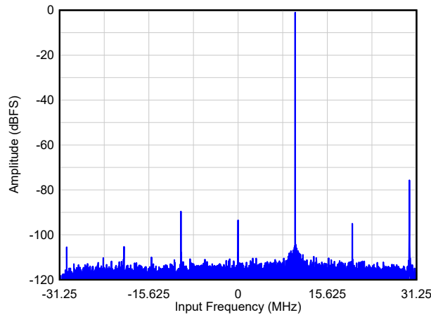
图 8-6. FFT3 : /8 抽取, A_{IN} = -1\text{dBFS}
