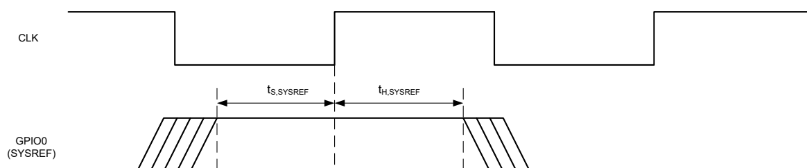
图 7-15. 时序：外部同步输入
