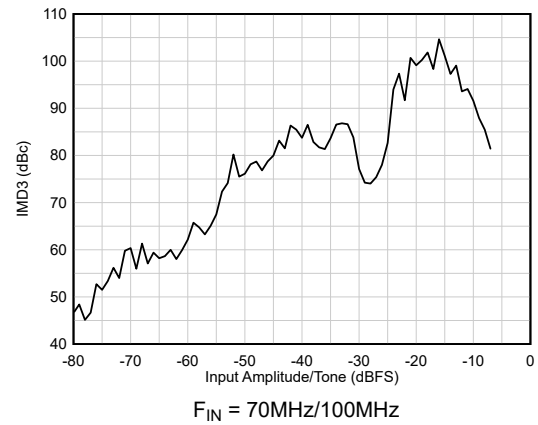
图 5-17. IMD3 与 A_{IN} 间的关系
