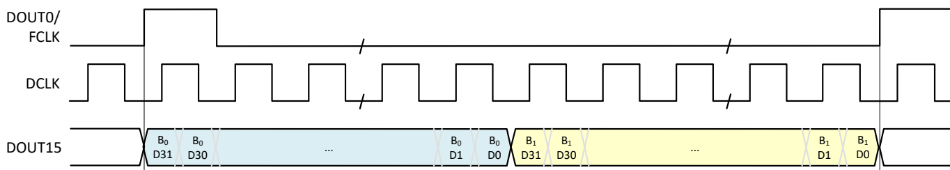
图 7-58. 示例 2 的 SLVDS 帧组装
