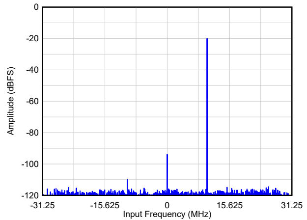
图 8-7. FFT4 : /8 抽取, A_{IN} = -20\text{dBFS}
