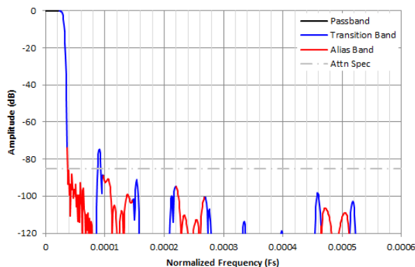
图 7-49. /16384 复数抽取滤波器响应
