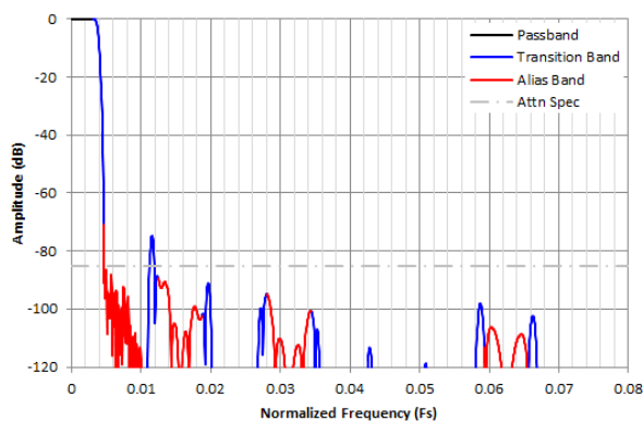
图 7-35. /128 复数抽取滤波器响应
