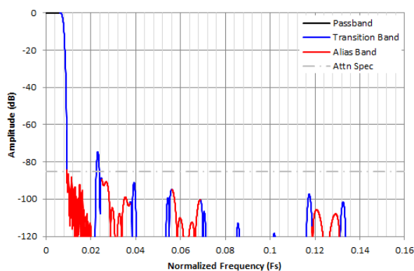
图 7-33. /64 复数抽取滤波器响应
