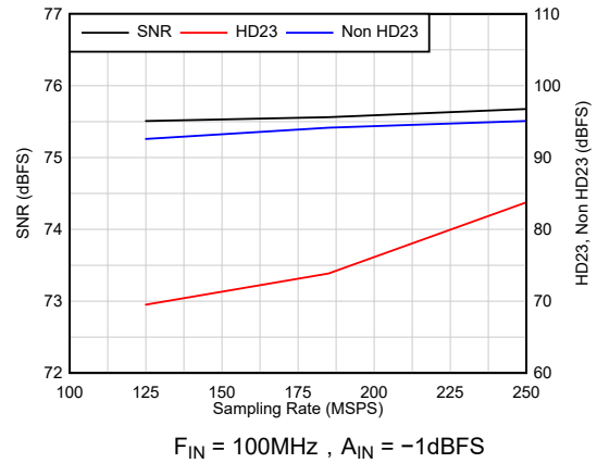
图 5-16. 交流性能与 F_S 间的关系
