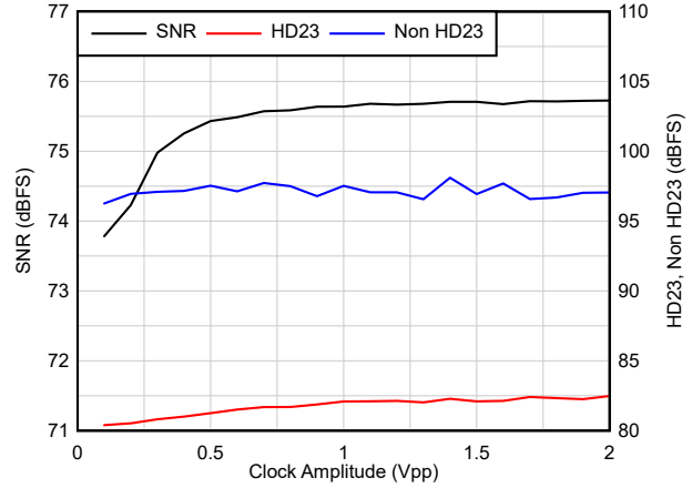
图 8-3. SNR 与时钟振幅间的关系 ( F_S = 500\text{MSPS} 、 F_{\text{IN}} = 100\text{MHz} 、 A_{\text{IN}} = -1\text{dBFS} )
