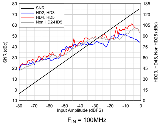
图 5-15. 交流性能与 A_{IN} 间的关系
