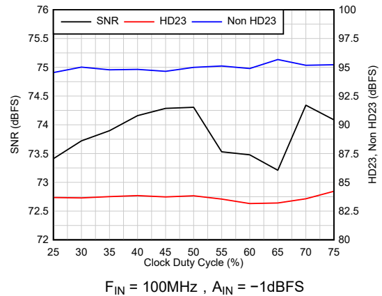
图 5-18. 交流性能与时钟占空比间的关系
