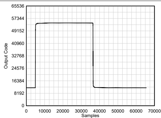
图 5-26. 脉冲响应
