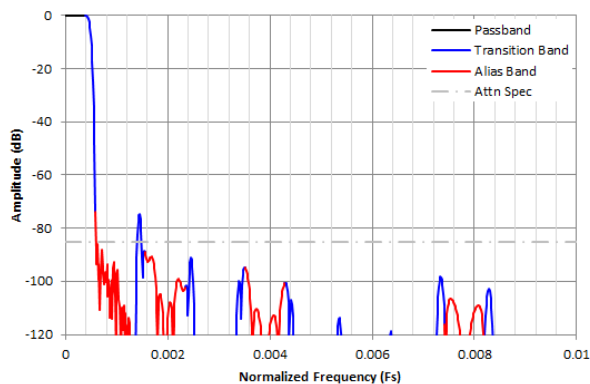
图 7-41. /1024 复数抽取滤波器响应
