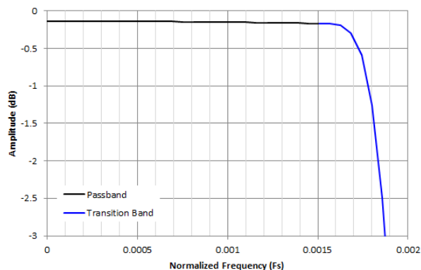
图 7-38. /256 抽取通带纹波响应
