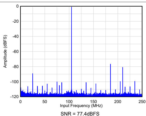
图 7-70. FFT - 2x AVG ( F_{IN} = 105\text{MHz} , A_{IN} = -1\text{dBFS} )
