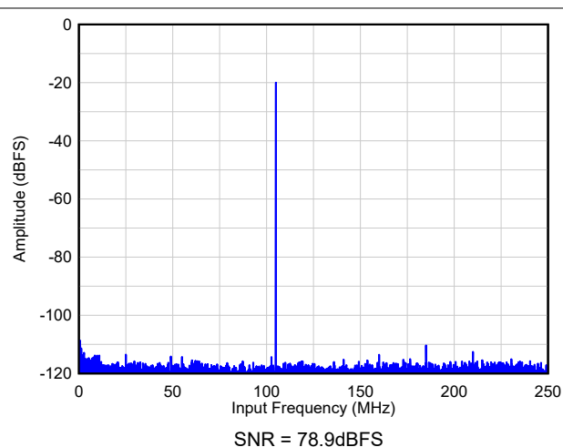
图 7-72. FFT - 2x AVG ( F_{IN} = 105\text{MHz} , A_{IN} = -20\text{dBFS} )
