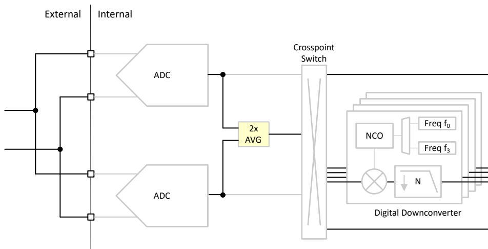
图 7-68. 数字通道平均示意图
