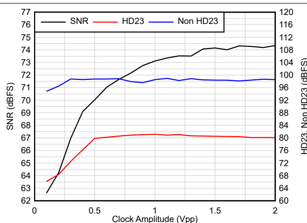
图 7-13. 交流性能与时钟振幅间的关系 F_S = 250\text{MSPS} 、 F_{IN} = 240\text{MHz} 、 A_{IN} = -1\text{dBFS}
