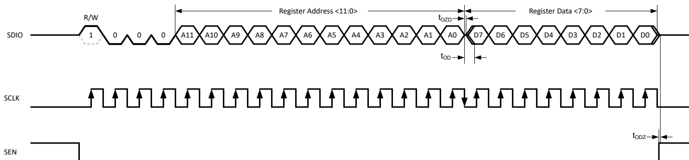
图 7-74. 串行寄存器读取时序图
