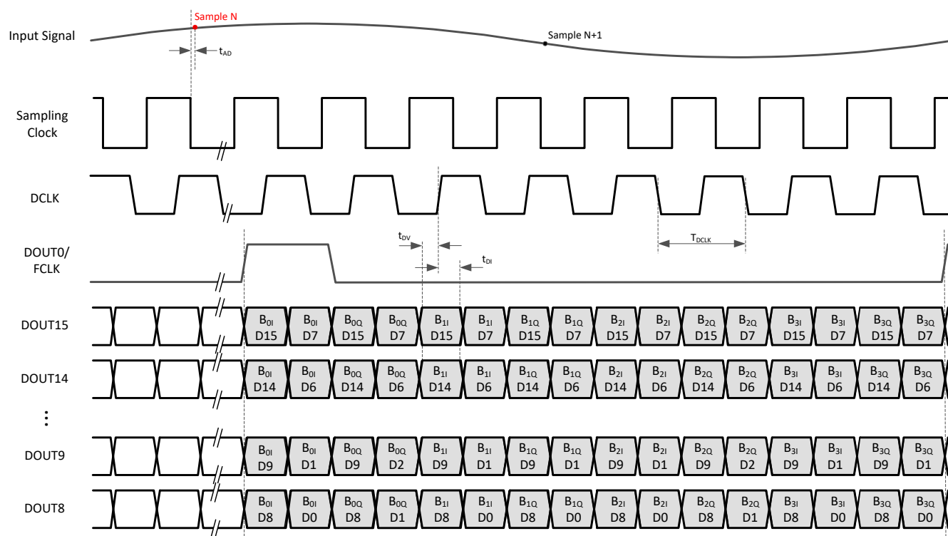
图 6-2. 时序图：串行 LVDS (示例：四频带、16 位、/8 复数抽取)
