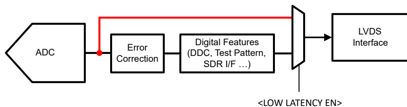
图 7-65. 低延迟模式
