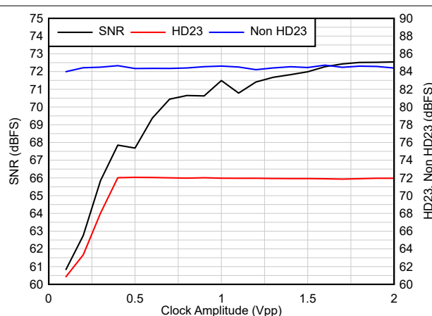
图 7-11. 交流性能与时钟振幅间的关系 F_S = 500\text{MSPS} 、 F_{IN} = 400\text{MHz} 、 A_{IN} = -1\text{dBFS}
