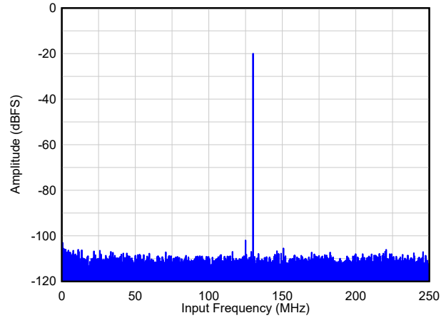
图 8-5. FFT2 : DDC 旁路, A_{IN} = -20\text{dBFS}
