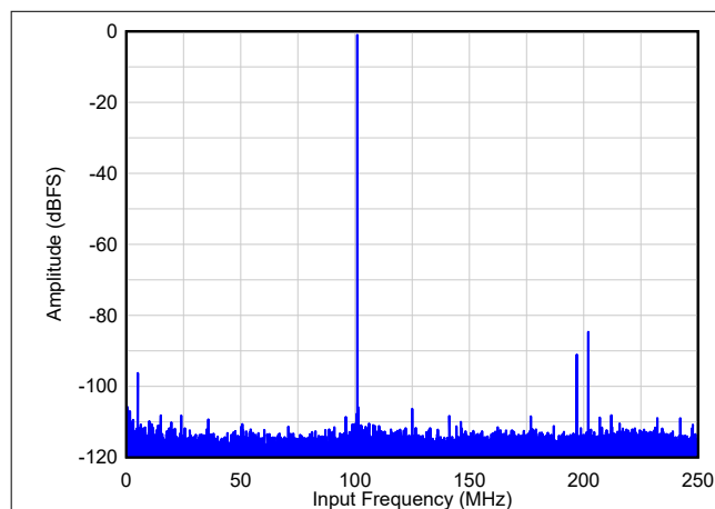
图 7-66. FFT : F_{IN} = 105\text{MHz} ，正常模式
