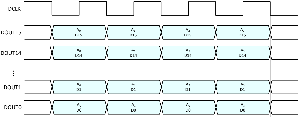
图 7-56. SDR LVDS 模式下的输出数据格式 ( CHA 有效 )
