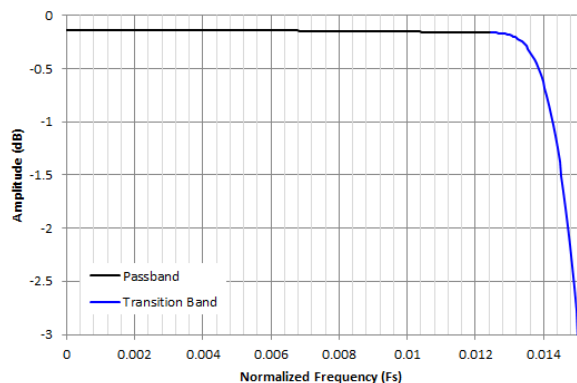
图 7-32. /32 抽取通带纹波响应
