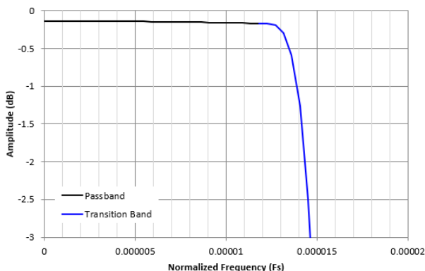
图 7-52. /32768 抽取通带纹波响应
