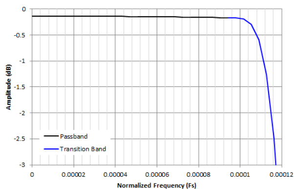
图 7-46. /4096 抽取通带纹波响应
