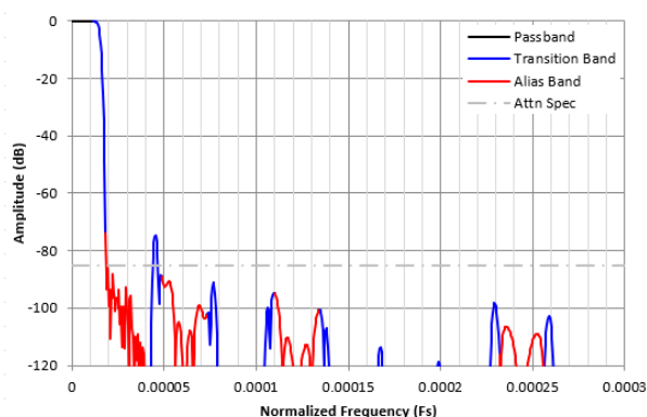
图 7-51. /32768 复数抽取滤波器响应
