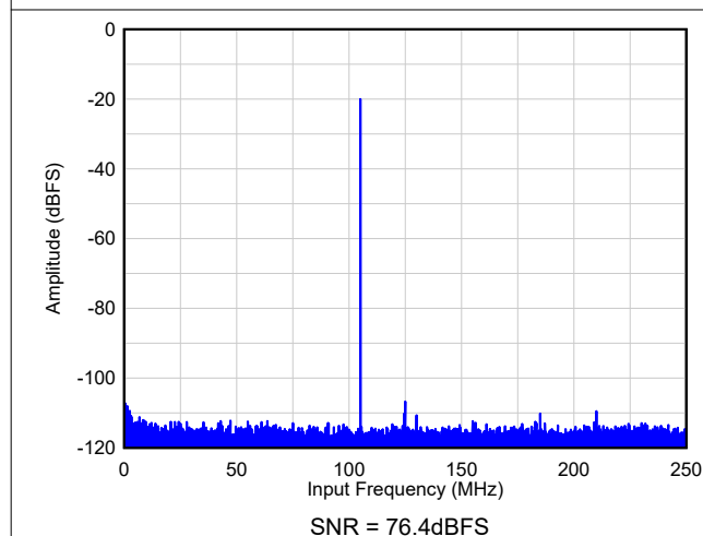
图 7-71. FFT - 无 AVG ( F_{IN} = 105\text{MHz} , A_{IN} = -20\text{dBFS} )
