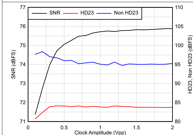
图 7-12. 交流性能与时钟振幅间的关系 F_S = 250\text{MSPS} 、 F_{IN} = 100\text{MHz} 、 A_{IN} = -1\text{dBFS}
