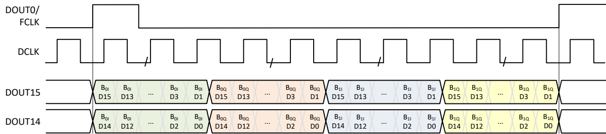
图 7-59. 示例 3 的 SLVDS 帧组装
