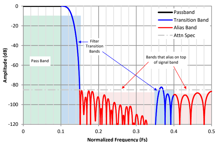
图 7-22. 抽取滤波器图的解释
