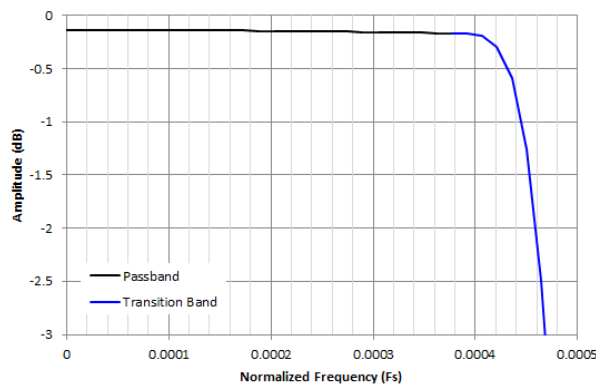
图 7-42. /1024 抽取通带纹波响应
