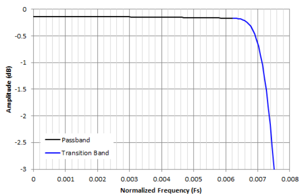
图 7-34. /64 复数抽取通带纹波响应
