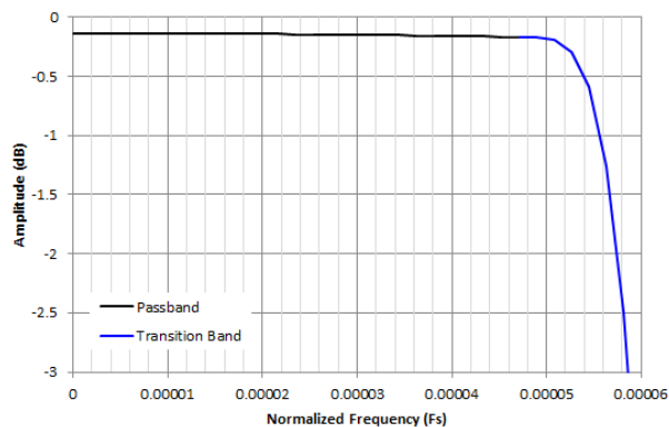
图 7-48. /8192 抽取通带纹波响应
