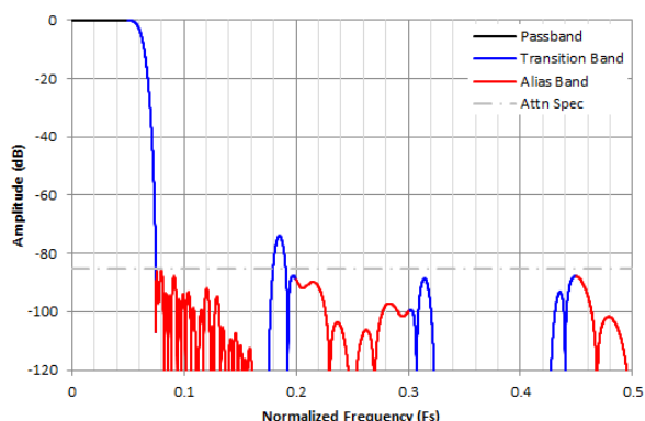
图 7-27. /8 复数抽取滤波器响应
