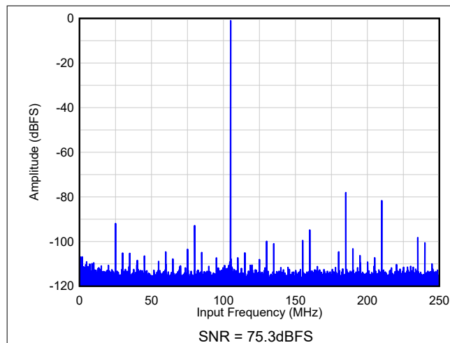
图 7-69. FFT - 无 AVG ( F_{IN} = 105\text{MHz} , A_{IN} = -1\text{dBFS} )
