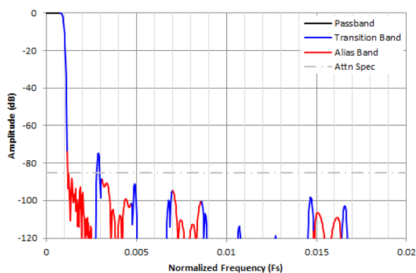
图 7-39. /512 复数抽取滤波器响应
