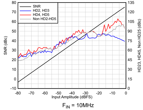
图 5-14. 交流性能与 A_{IN} 间的关系
