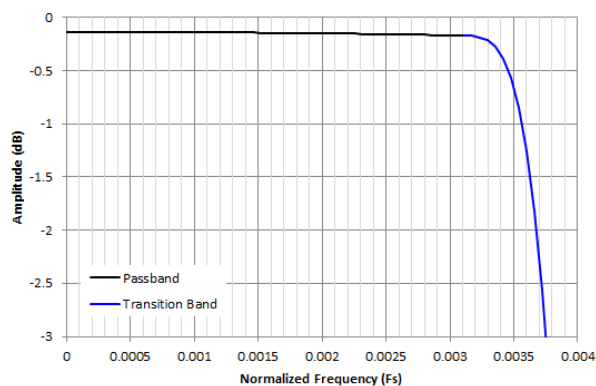
图 7-36. /128 抽取通带纹波响应
