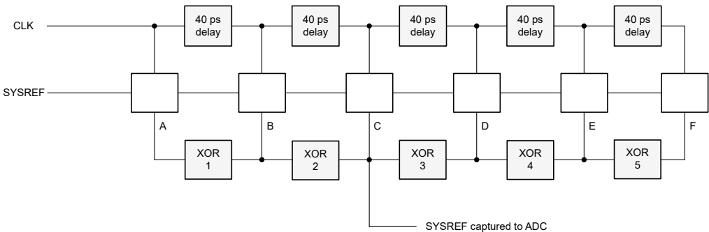
图 7-16. SYSREF 检测电路
