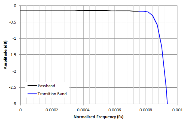
图 7-40. /512 抽取通带纹波响应
