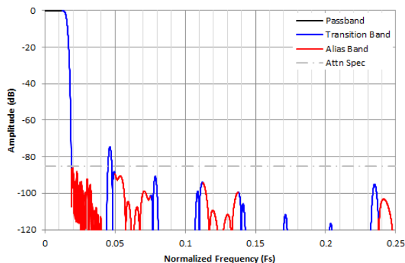
图 7-31. /32 复数抽取滤波器响应
