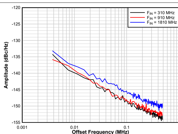
图 7-9. 振幅噪声示例
