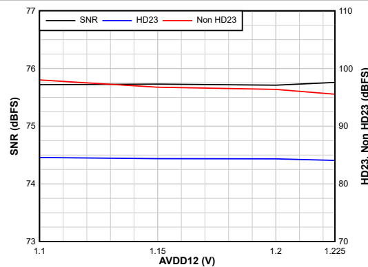
图 5-20. 交流性能与 AVDD12 间的关系
