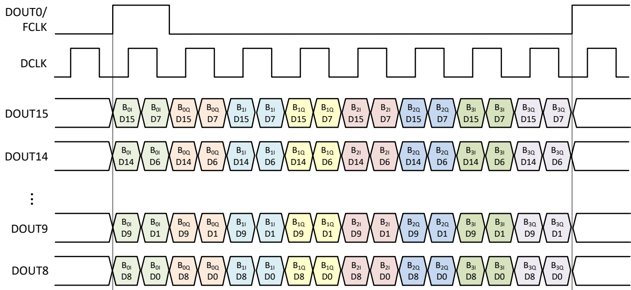
图 7-60. 示例 4 的 SLVDS 帧组装
