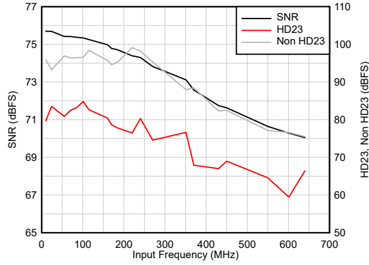
图 5-13. 交流性能与 F_{IN} 间的关系
