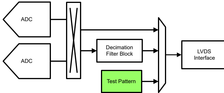
图 7-64. 测试图形发生器
