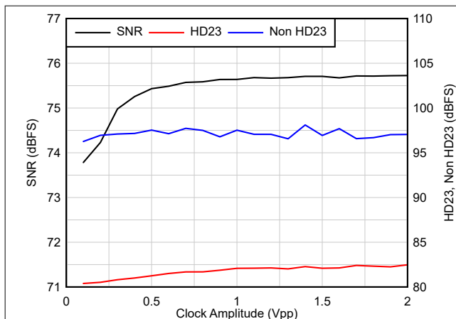
图 7-10. 交流性能与时钟振幅间的关系 F_S = 500\text{MSPS} 、 F_{IN} = 100\text{MHz} 、 A_{IN} = -1\text{dBFS}
