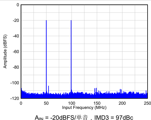
图 5-39. F_{IN} = 445\text{MHz}/455\text{MHz} 时的双音 FFT
