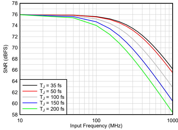
图 8-2. SNR 与 T_{\text{Jitter}} 与 F_{\text{IN}} 间的关系
