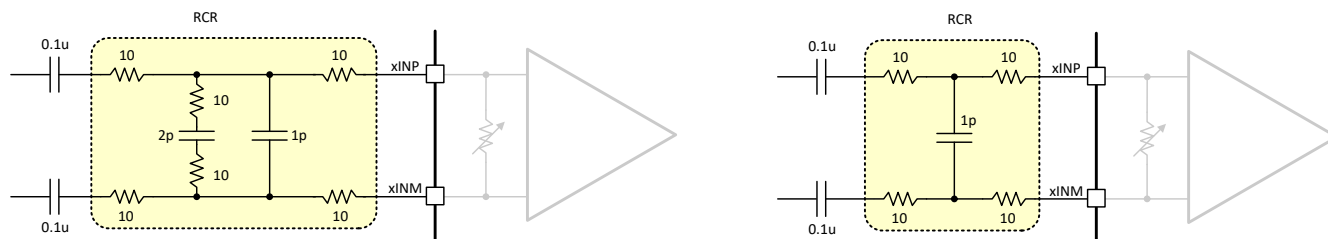
图 7-6. F_{IN} < 500\text{MHz} (左) 和 F_{IN} > 500\text{MHz} (右) 的外部 RCR
