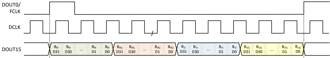
图 7-61. 示例 5 的 SLVDS 帧组装
