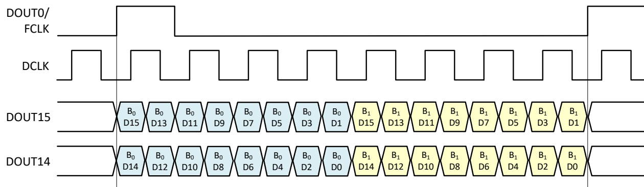
图 7-57. 示例 1 的 SLVDS 帧组装
