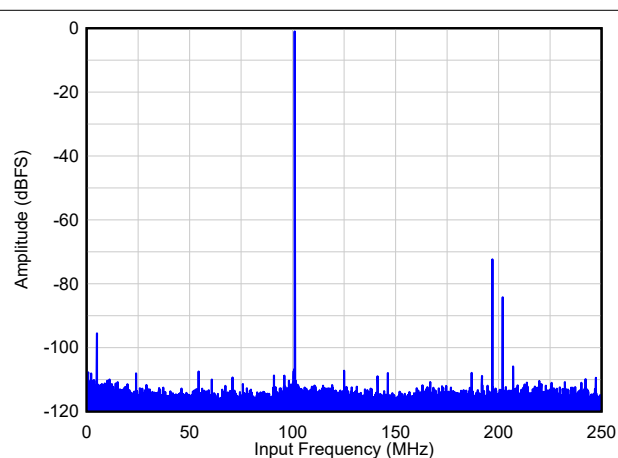
图 7-67. FFT : F_{IN} = 105\text{MHz} ，低延迟模式
