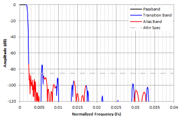
图 7-37. /256 复数抽取滤波器响应
