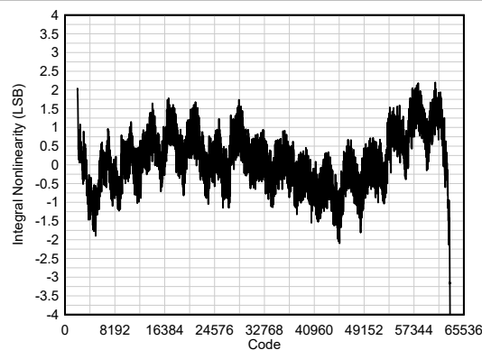
图 5-52. INL
