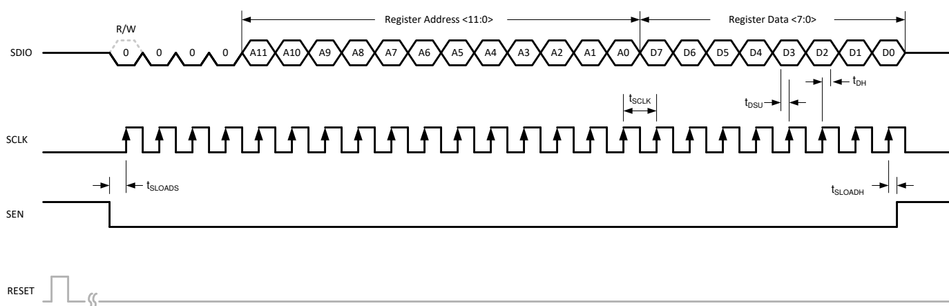
图 7-73. 串行寄存器写入时序图
