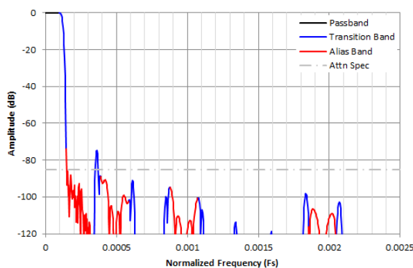
图 7-45. /4096 复数抽取滤波器响应
