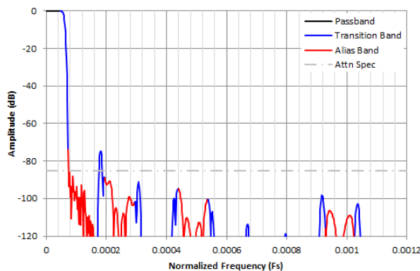
图 7-47. /8192 复数抽取滤波器响应
