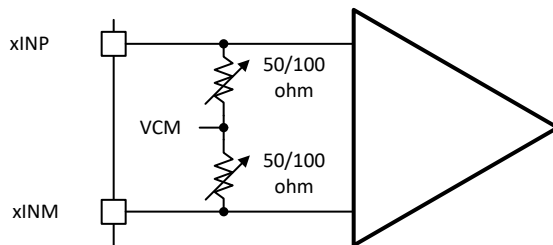
图 7-2. 模拟输入内部端接
