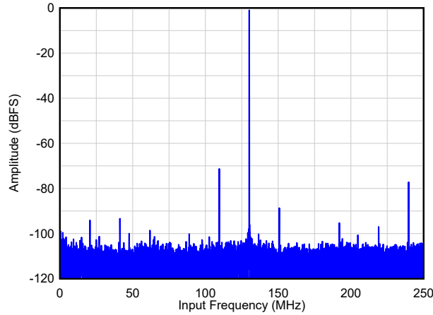
图 8-4. FFT1 : DDC 旁路, A_{IN} = -1\text{dBFS}
