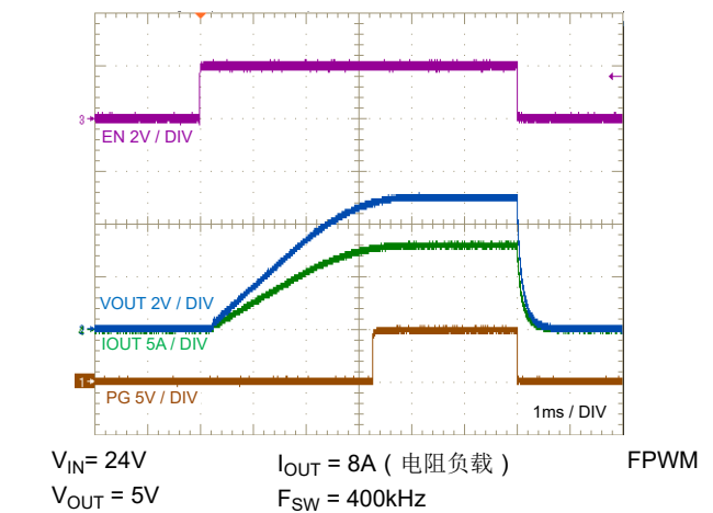
图 7-14. EN 启动特性
