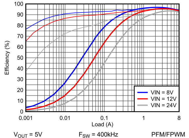
图 7-10. 效率与 I_{OUT} 间的关系，对数标度
