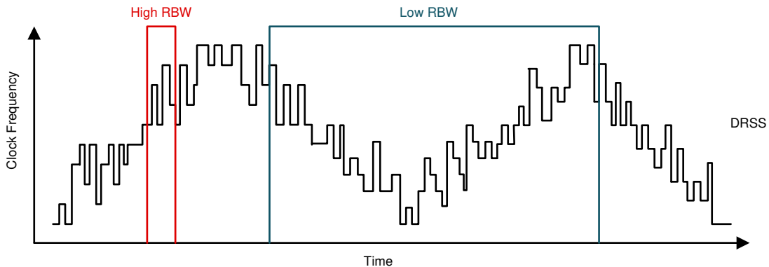
图 6-3. 双随机展频实现
