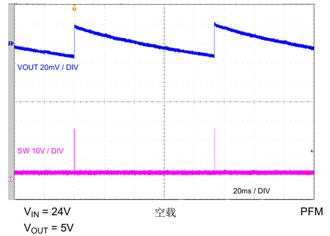
图 7-12. PFM 开关
