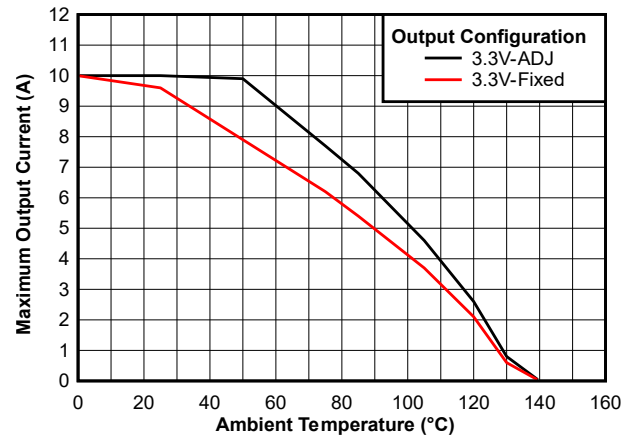
图 7-5. 最大输出电流与环境温度间的关系
