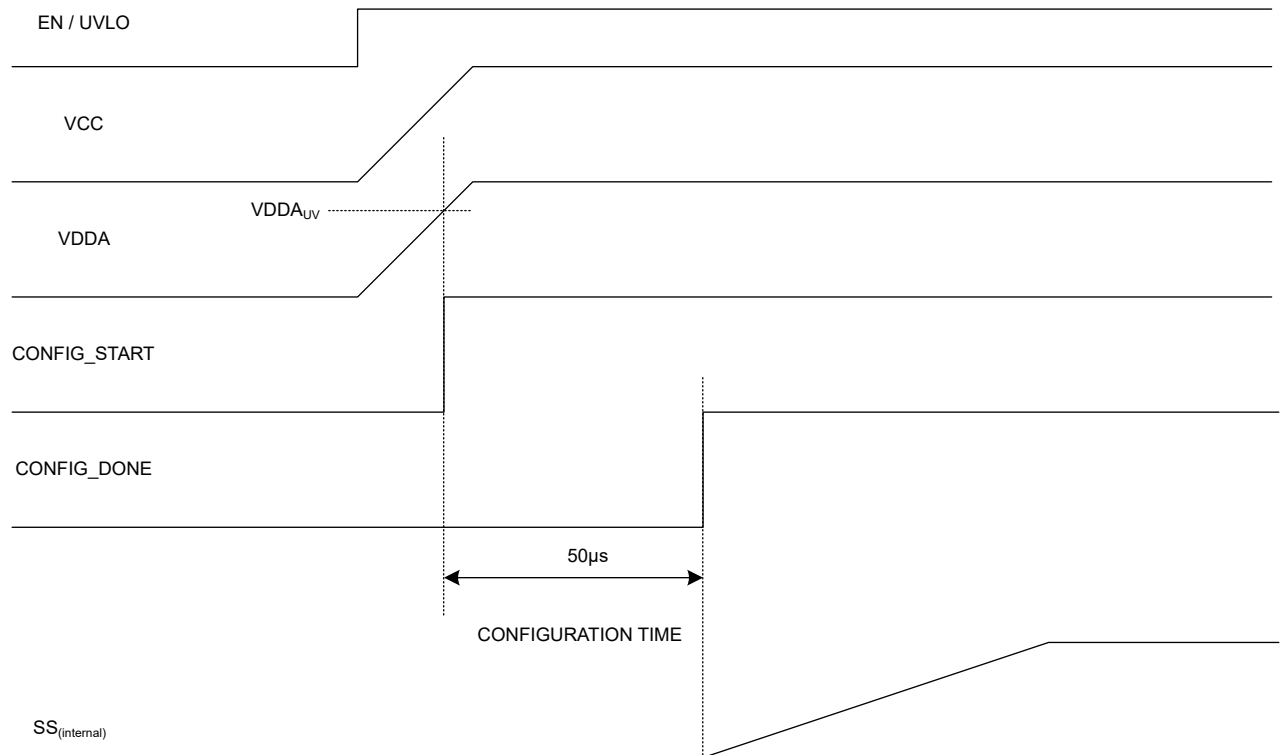
图 6-5. 配置时序
