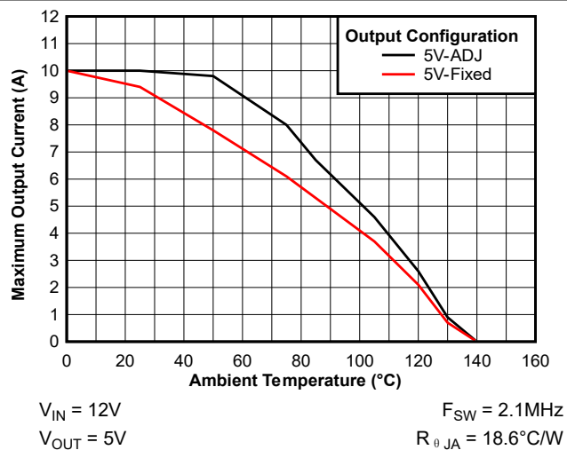
图 7-11. 最大输出电流与环境温度间的关系
