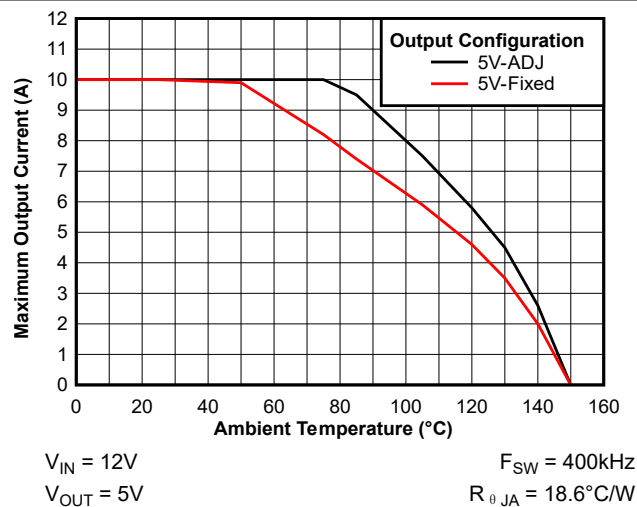
图 7-10. 最大输出电流与环境温度间的关系
