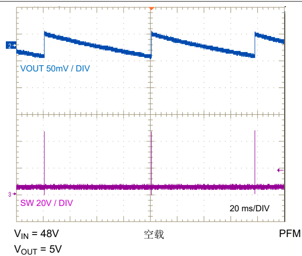
图 7-16. PFM 开关
