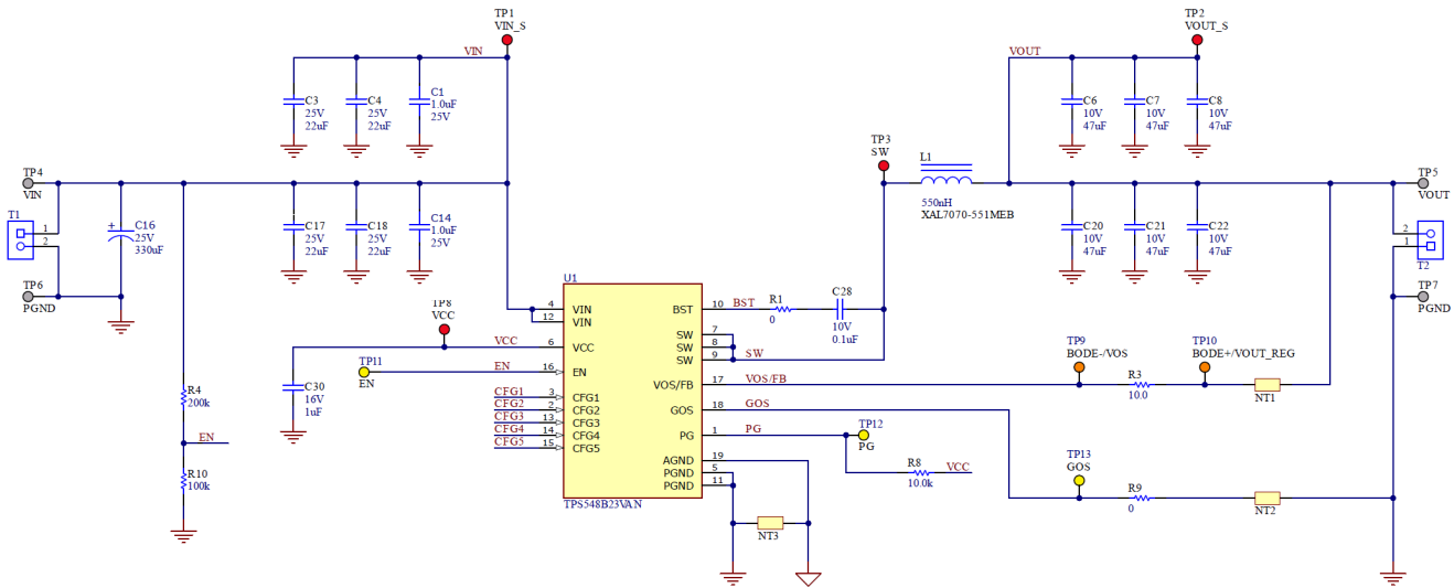
图 8-1. 应用电路图
