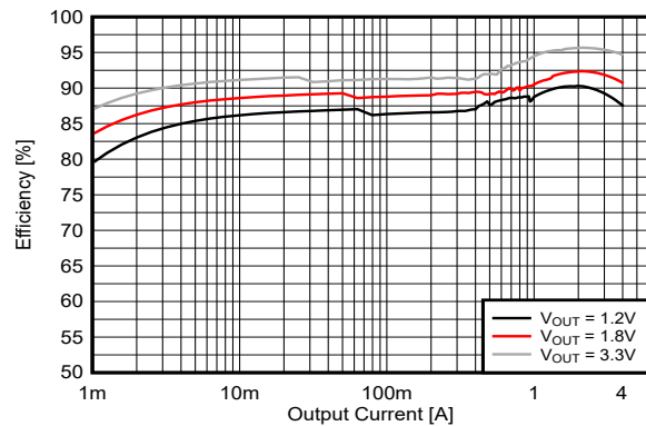
效率与输出电流间的关系曲线 ( V_{IN} = 5\text{V} 时 )
