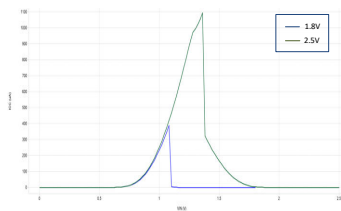
图 5-1. 电源电流与输入电源电压 ( 1.8V 至 2.5V ) 间的关系
