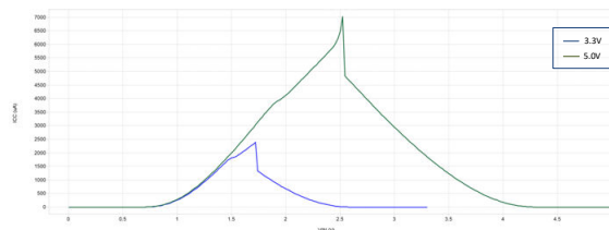
图 5-2. 电源电流与输入电源电压 ( 3.3V 至 5.0V ) 间的关系
