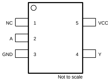
图 4-2. SN74LVC1G16-Q1 DCK 封装，5 引脚 SOT-SC70 (顶视图)
