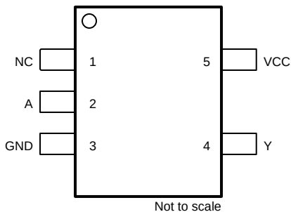
图 4-1. SN74LVC1G16 DBV 封装，5 引脚 SOT-23 (顶视图)
