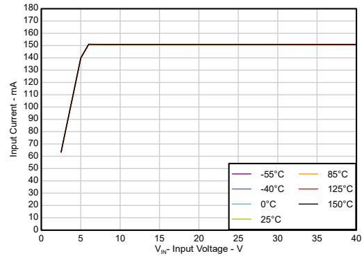
图 5-2. 输入电流与输入电压间的关系
