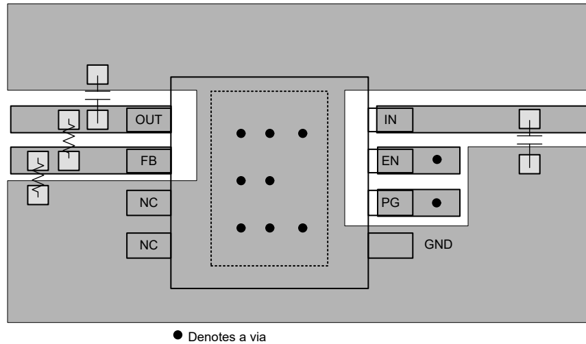
图 7-6. SOIC (D) 封装可调节输出
