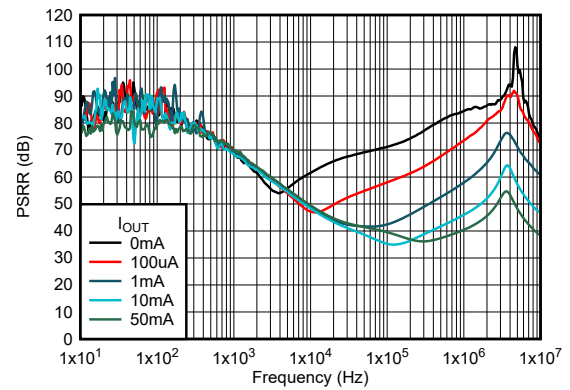
图 5-26. 波纹抑制与频率
