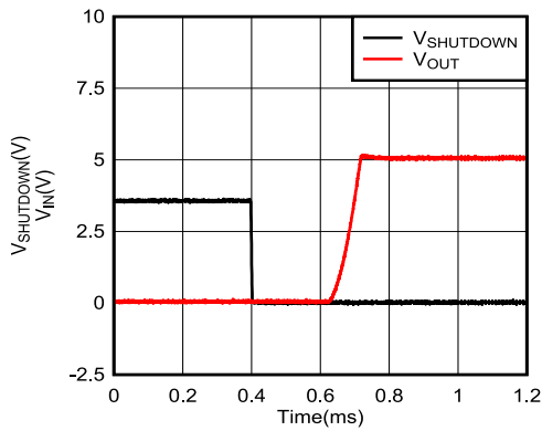
图 5-25. 使能瞬态响应与时间之间的关系
