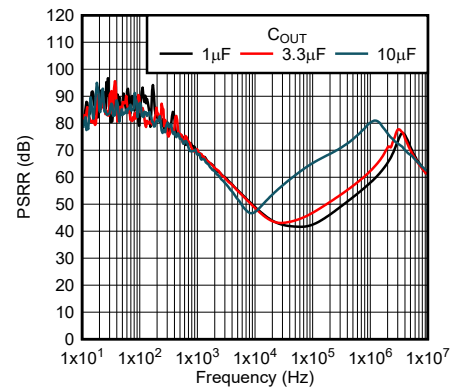
图 5-26. 波纹抑制与频率
