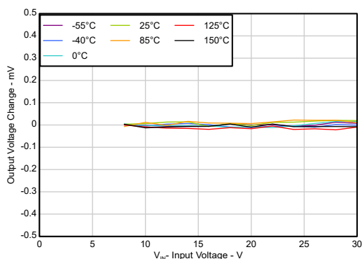
图 5-19. 线性调整率与输入电压间的关系
