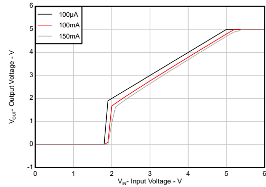
图 5-16. PG 比较器输出与输入电压间的关系
