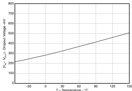
压降电压与温度间的关系
