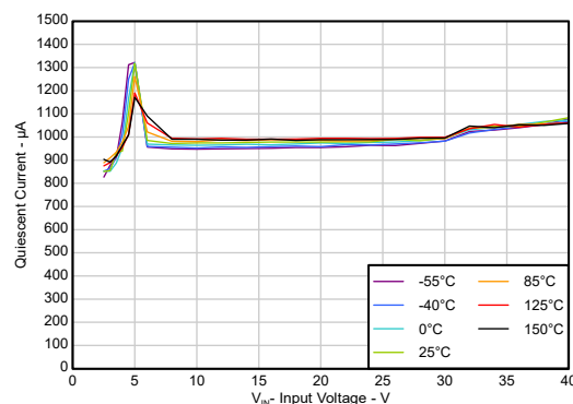
图 5-8. 静态电流与输入电压间的关系 ( I_{OUT} = 150mA )
