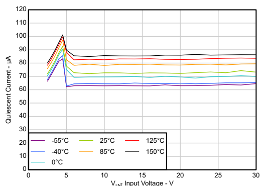
图 5-7. 静态电流与输入电压间的关系 ( I_{OUT} = 1mA )
