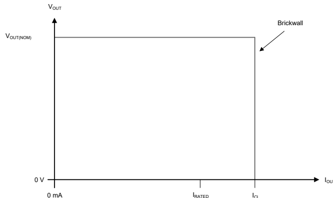
图 6-3. 电流限制
