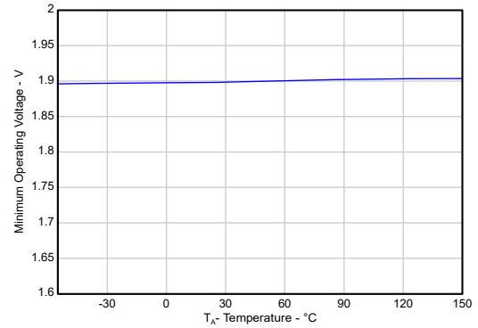
图 5-14. 最低工作电压与温度间的关系
