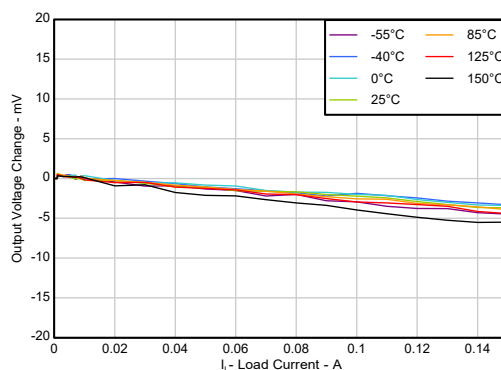
图 5-20. 负载调整率与负载电流间的关系
