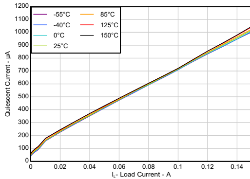
图 5-1. 静态电流与负载电流间的关系
