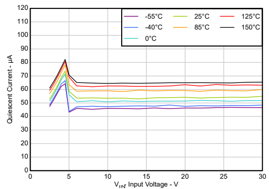
图 5-4. 输入电流与输入电压间的关系
