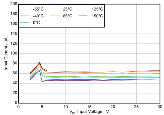
图 5-2. 输入电流与输入电压间的关系
