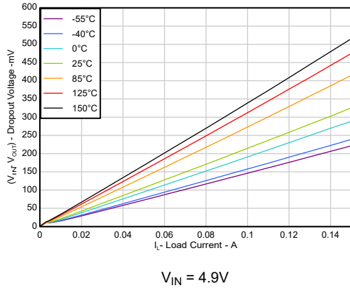
图 5-13. 压降电压与输出电流间的关系
