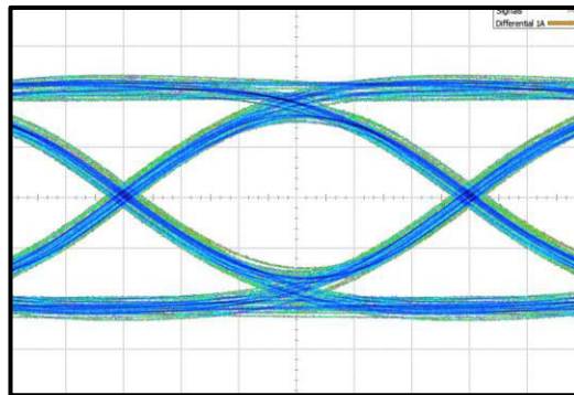
图 5-14. 在 10Gbps 时, 具有 12 英寸输入 PCB 布线的 USB 3.1 第 2 代眼图性能
