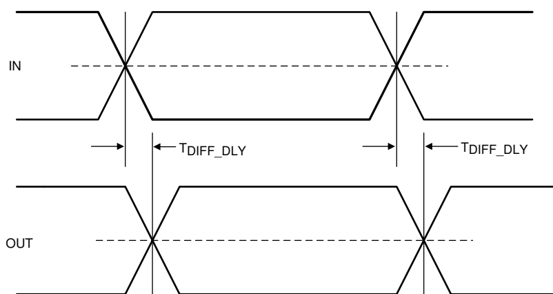
图 6-3. 传播延迟
