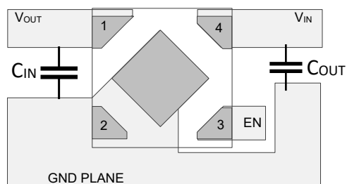
图 7-2. DQN 封装 (X2SON) 典型布局
