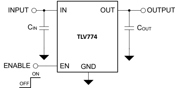
图 7-1. TLV774 典型应用
