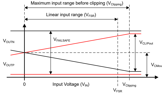
图 6-2. AMC0381D-Q1 的输入到输出传递曲线
