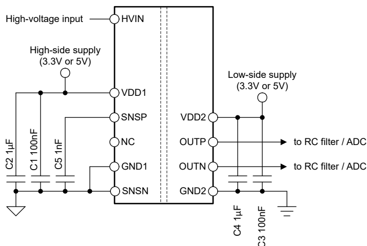
图 7-1. AMC0381D-Q1 去耦
