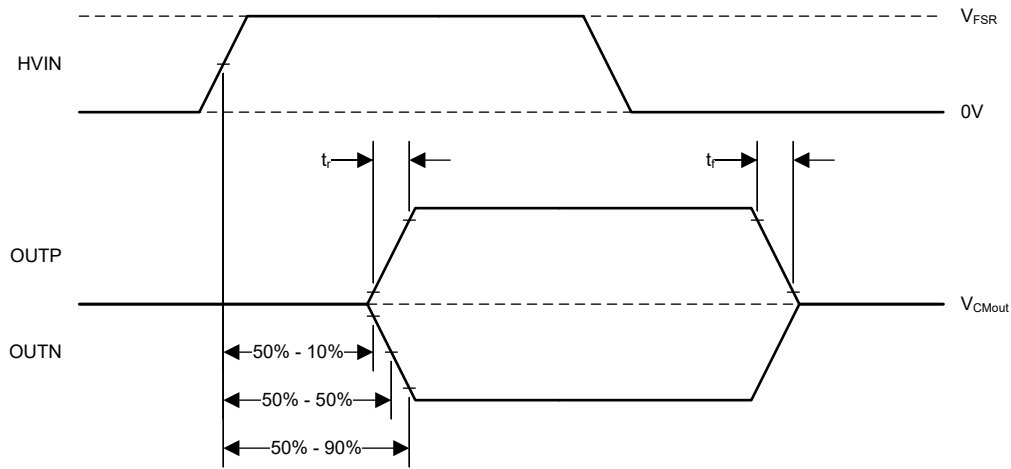
图 5-1. 上升、下降和延迟时间定义
