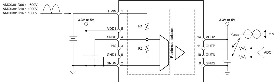
典型应用
