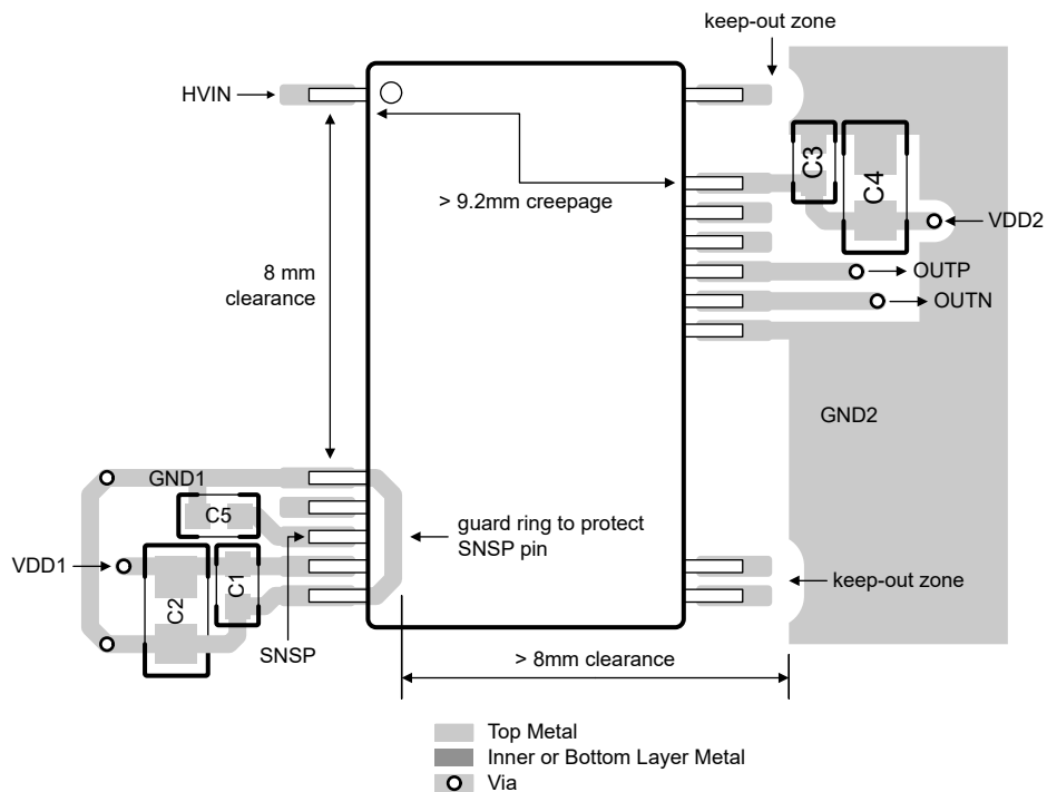
图 7-2. AMC0381D-Q1 的建议布局
