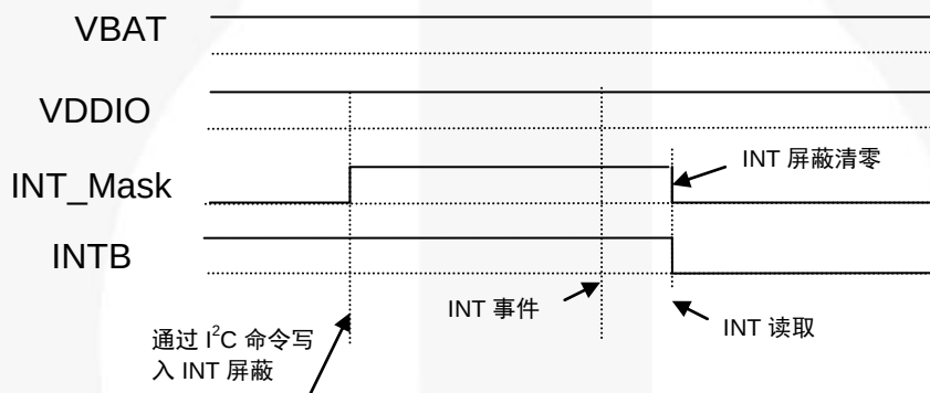
图 8. INT 屏蔽至 INTB 中断的时序图
