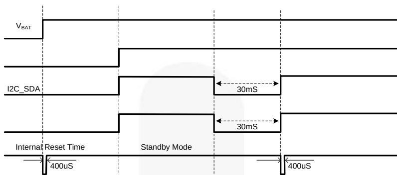
图 7. I 2 C 复位模式时序
