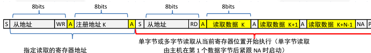
图 3. I 2 C 的写顺序
