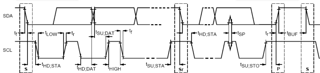
图 6. I 2 C 总线 ® 上全速模式器件时序定义
