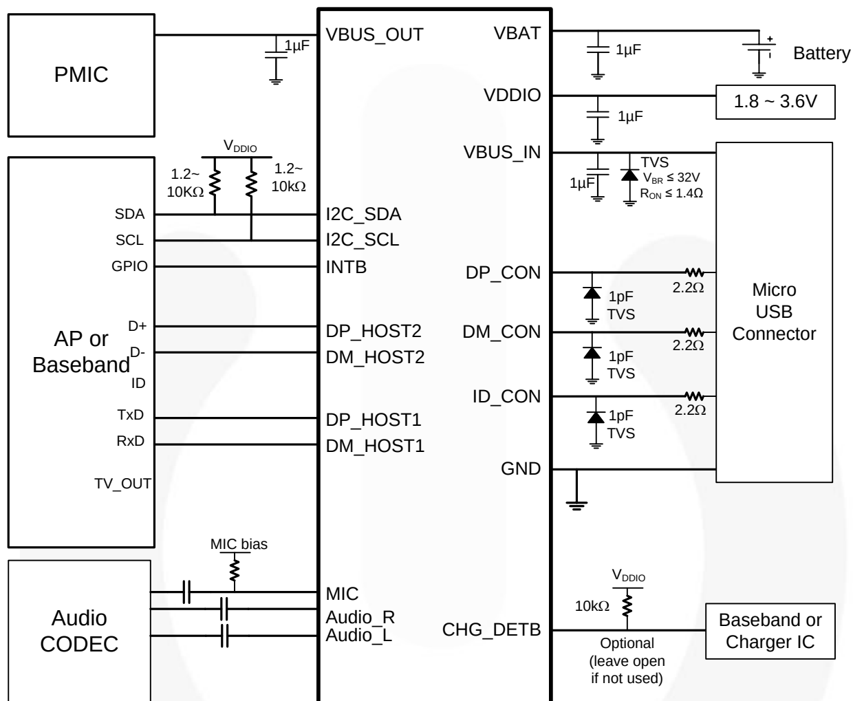
图 13. 参考原理图
