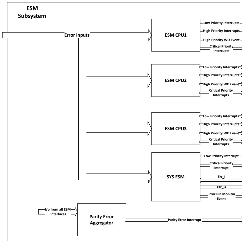
图 7-2. ESM-SS 方框图
