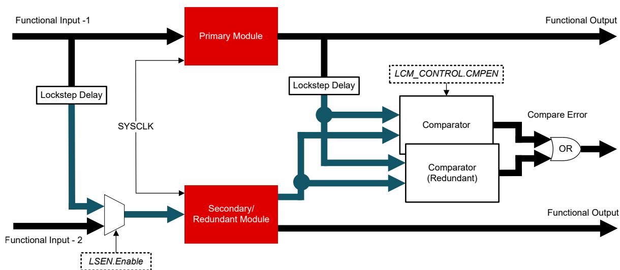
图 7-22. LCM 方框图
