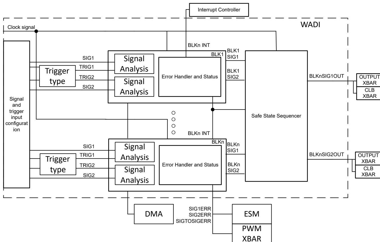
图 7-17. WADI 方框图
