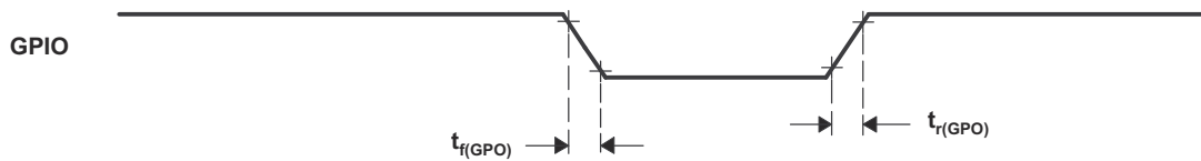
图 6-19. 通用输出时序
