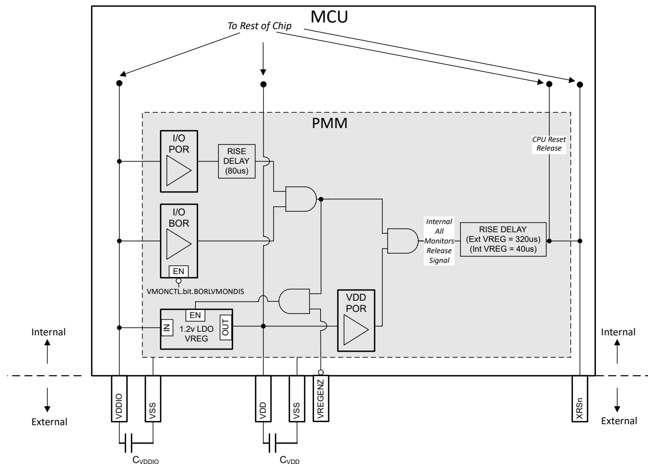
图 6-1. PMM 方框图
