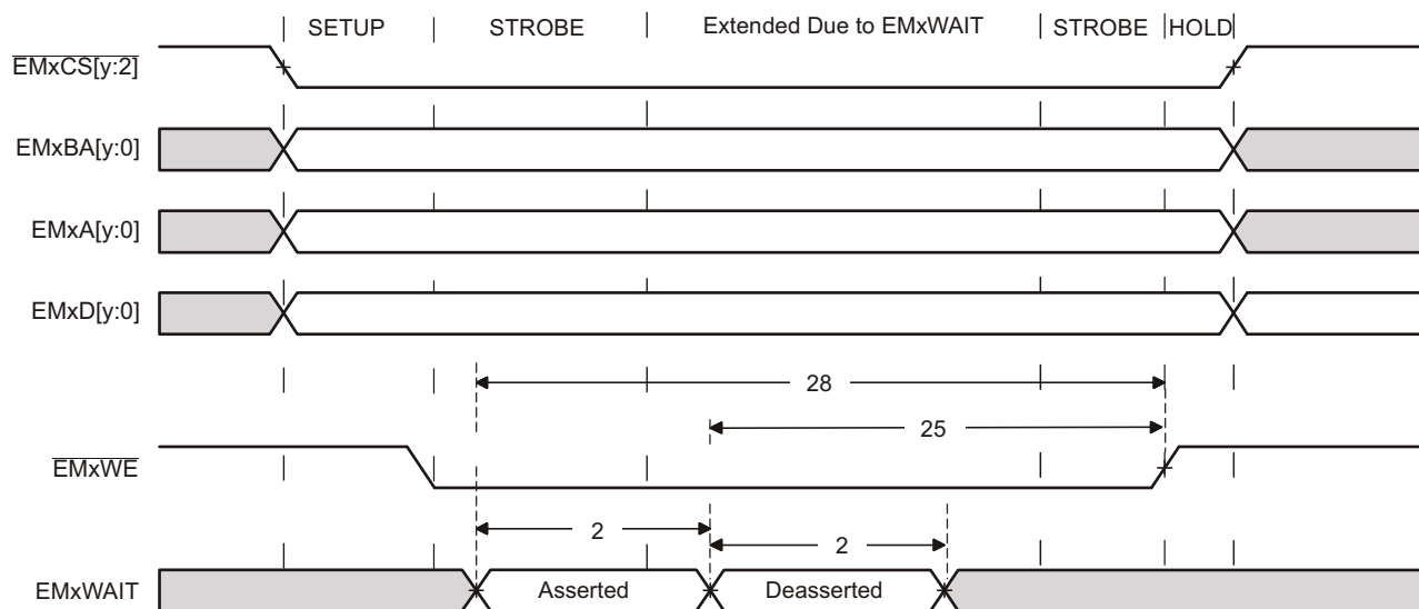
图 6-30. EMxWAIT 写入时序要求
