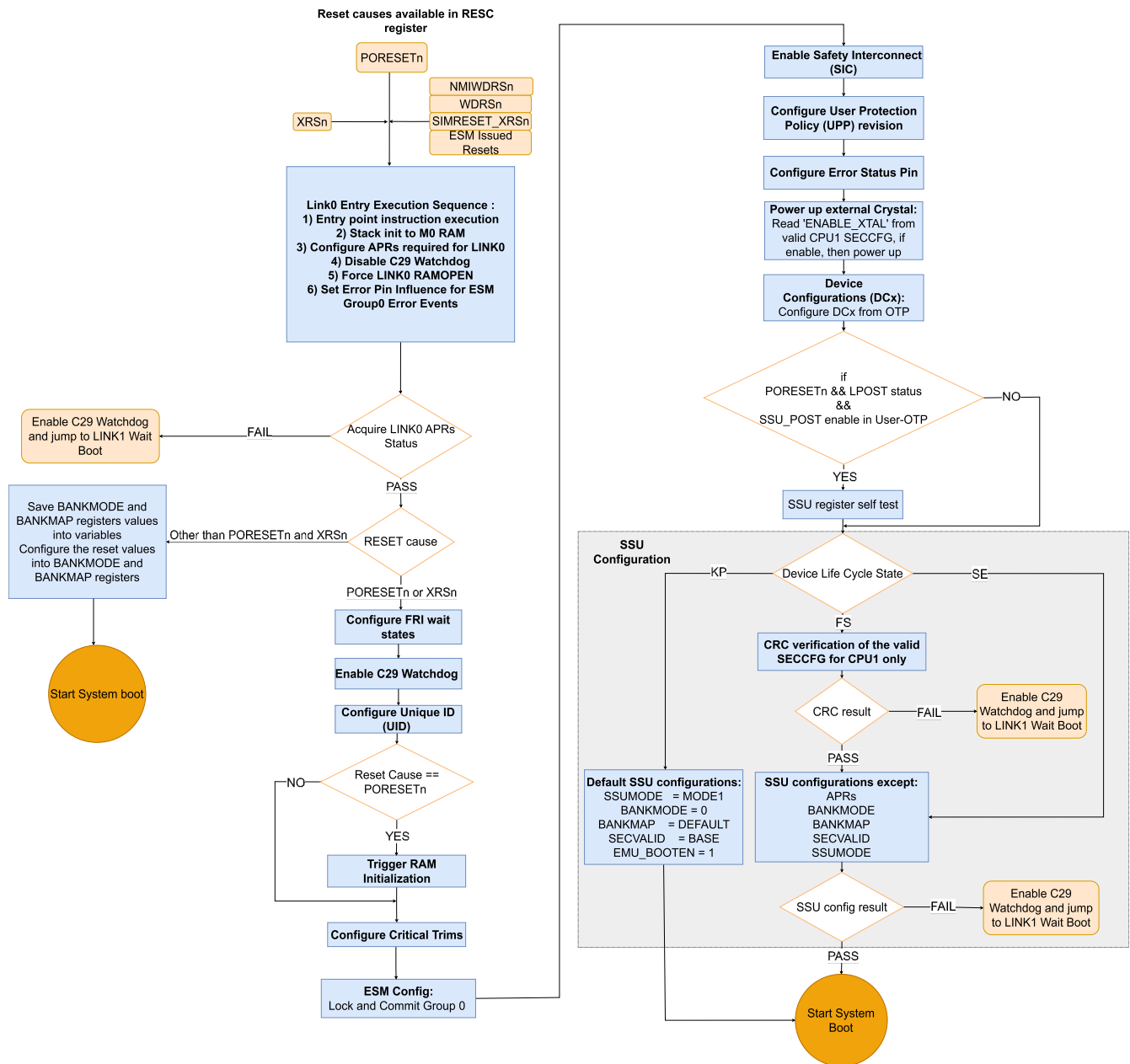
图 7-7. 从复位到系统启动的器件引导流程
