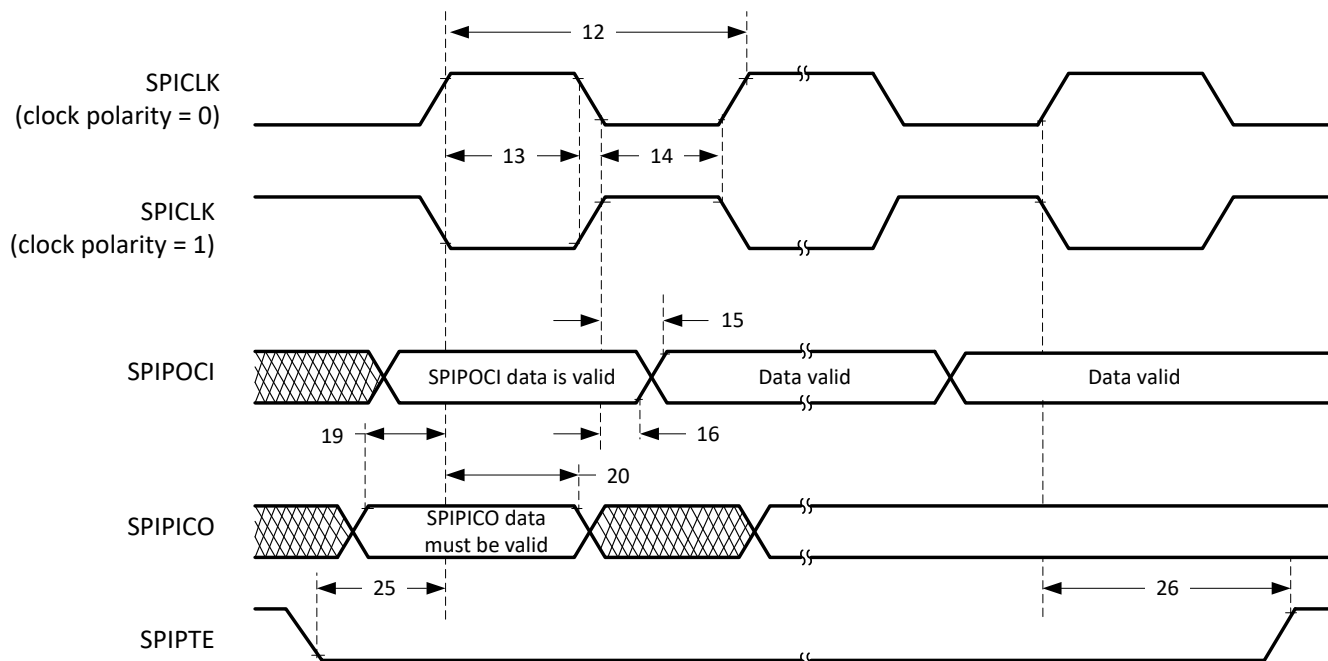
图 6-80. SPI 外设模式外部时序 (时钟相位 = 1)
