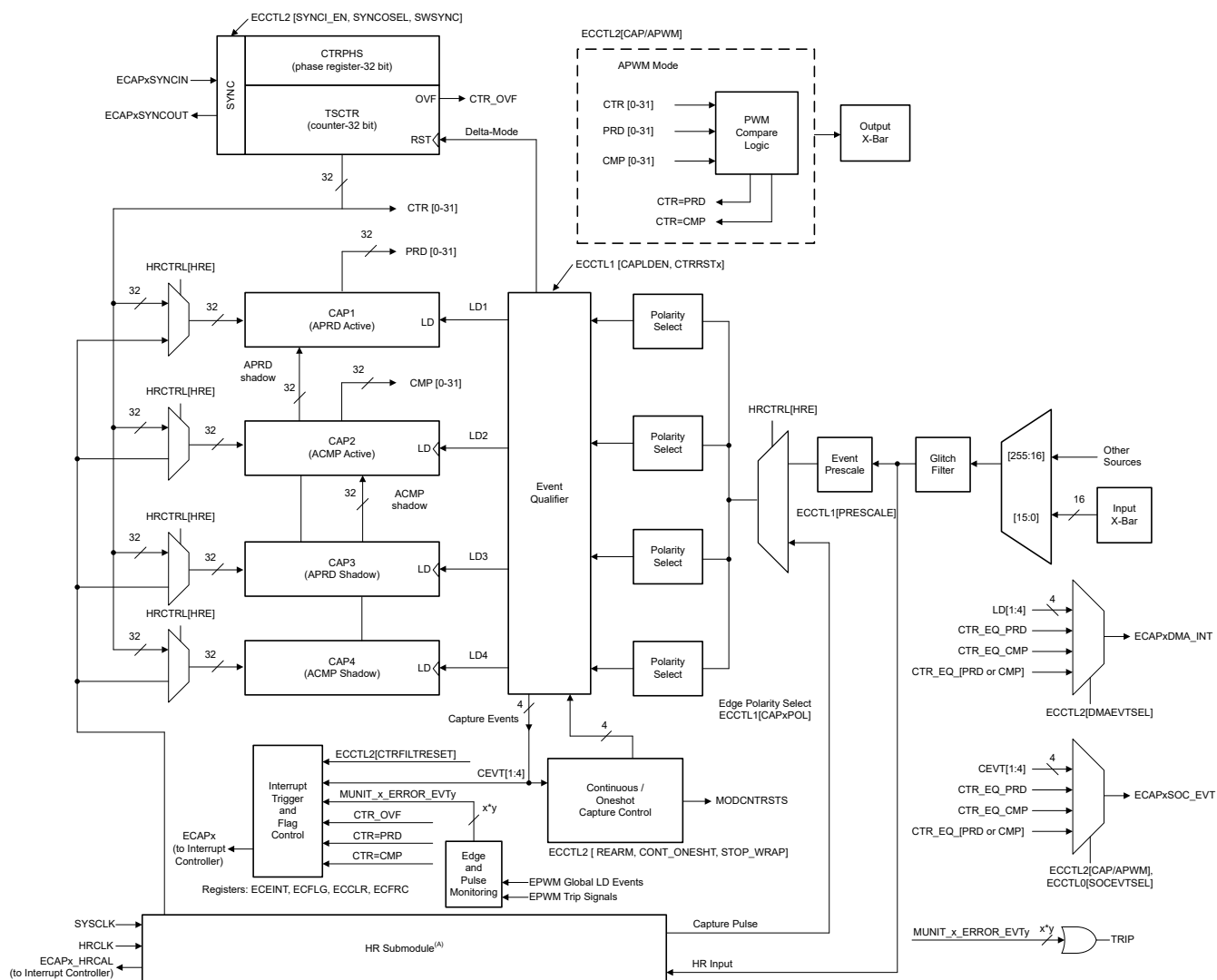
图 6-53. eCAP 方框图
