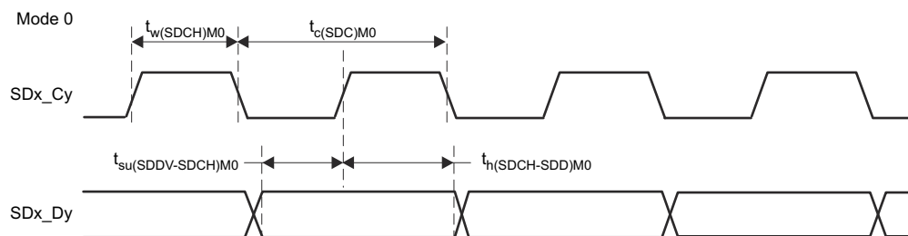
图 6-64. SDFM 时序图 - 模式 0
