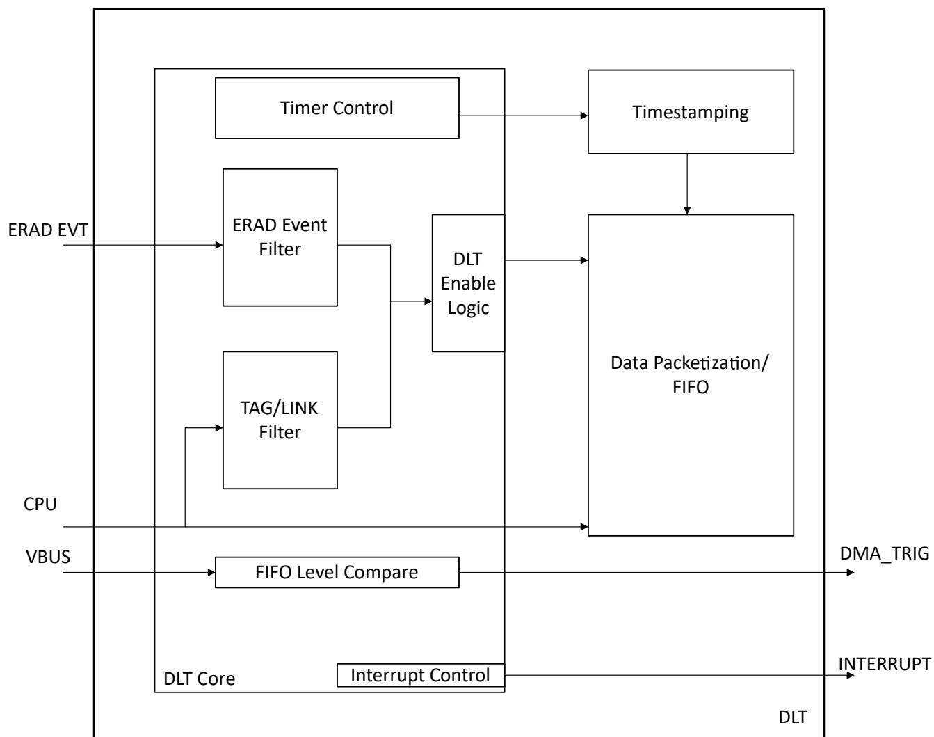
图 7-16. DLT 方框图
