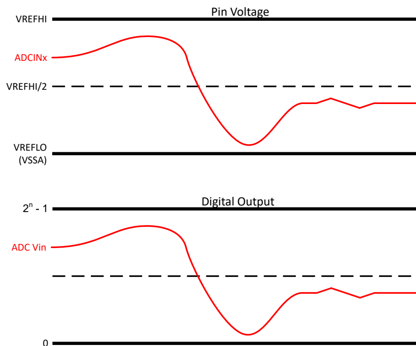
图 6-36. 单端信号模式
