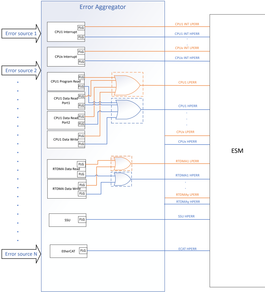
图 7-4. 错误聚合器接口
