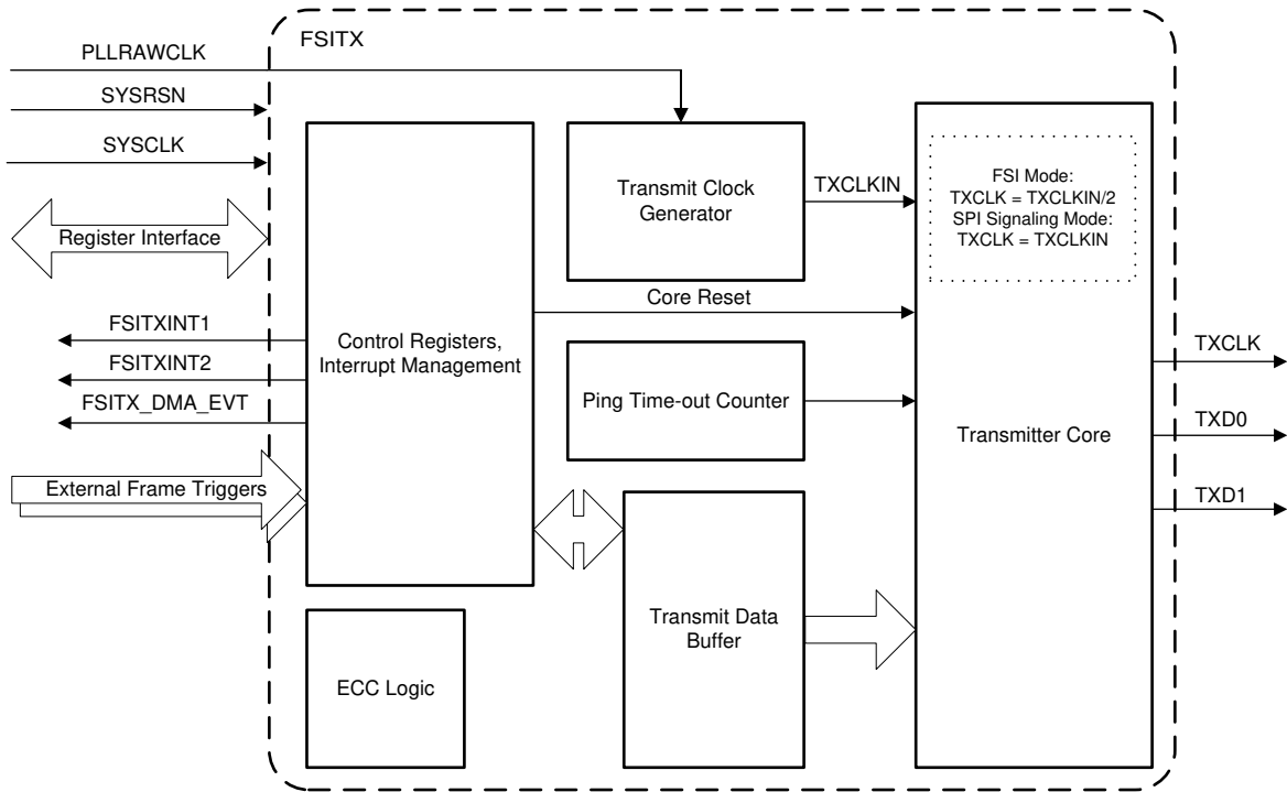
图 6-67. FSITX 方框图
