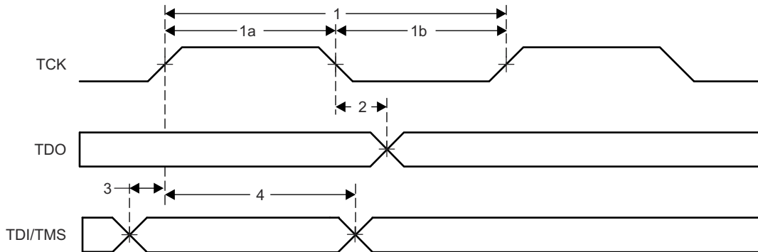
图 6-17. JTAG 时序
