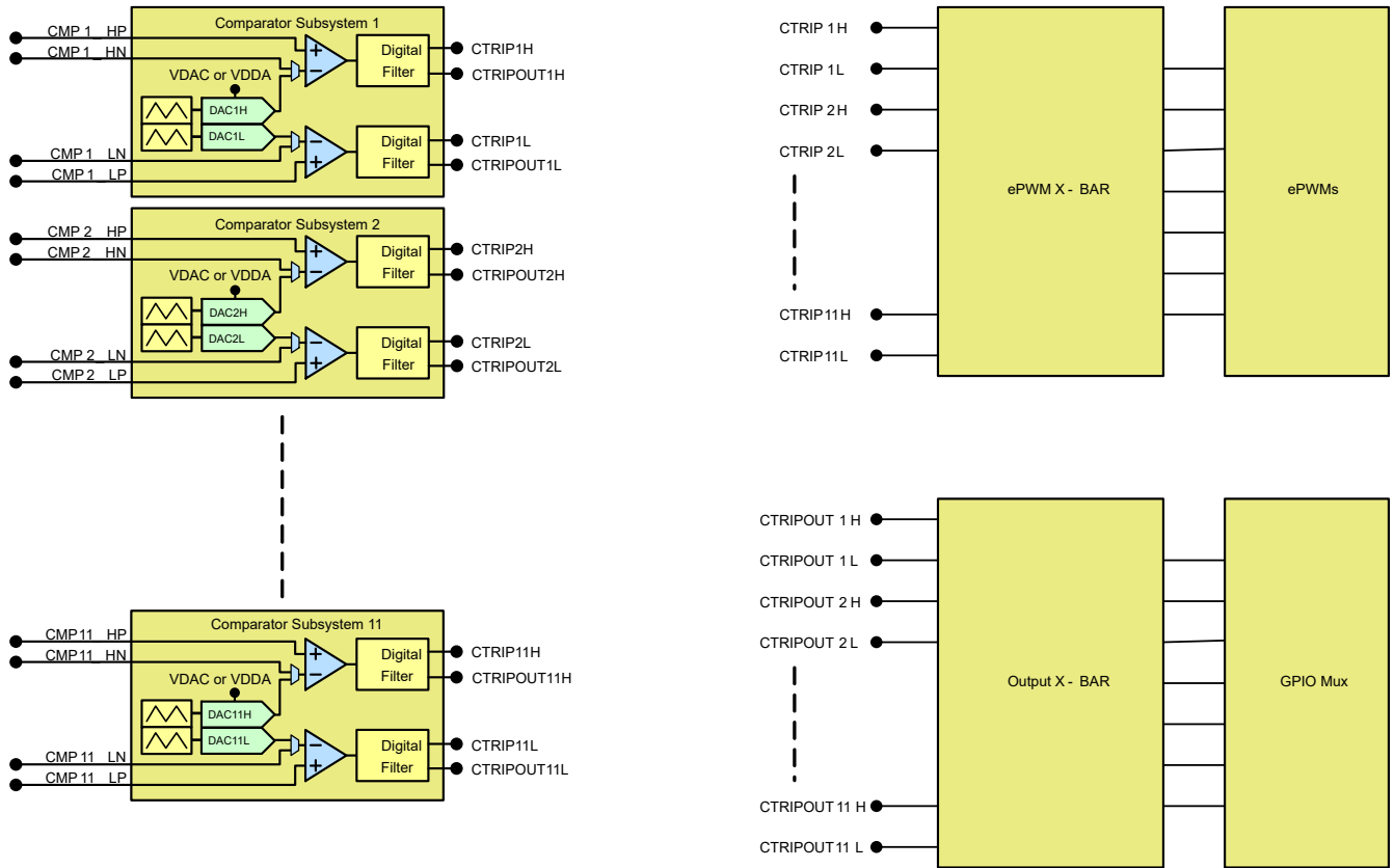
图 6-44. CMPSS 连接
