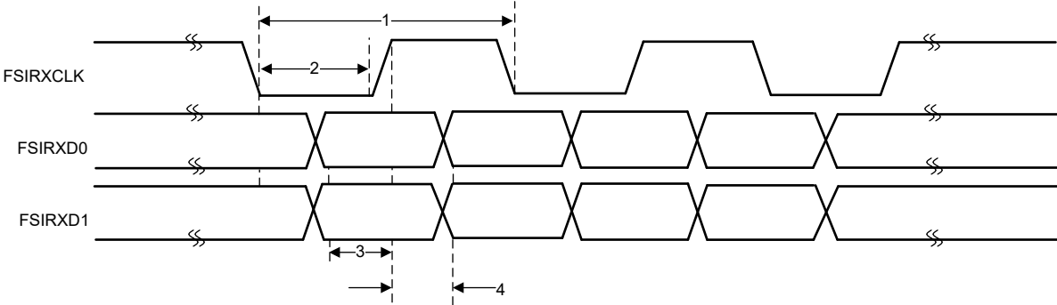
图 6-71. FSIRX 时序
