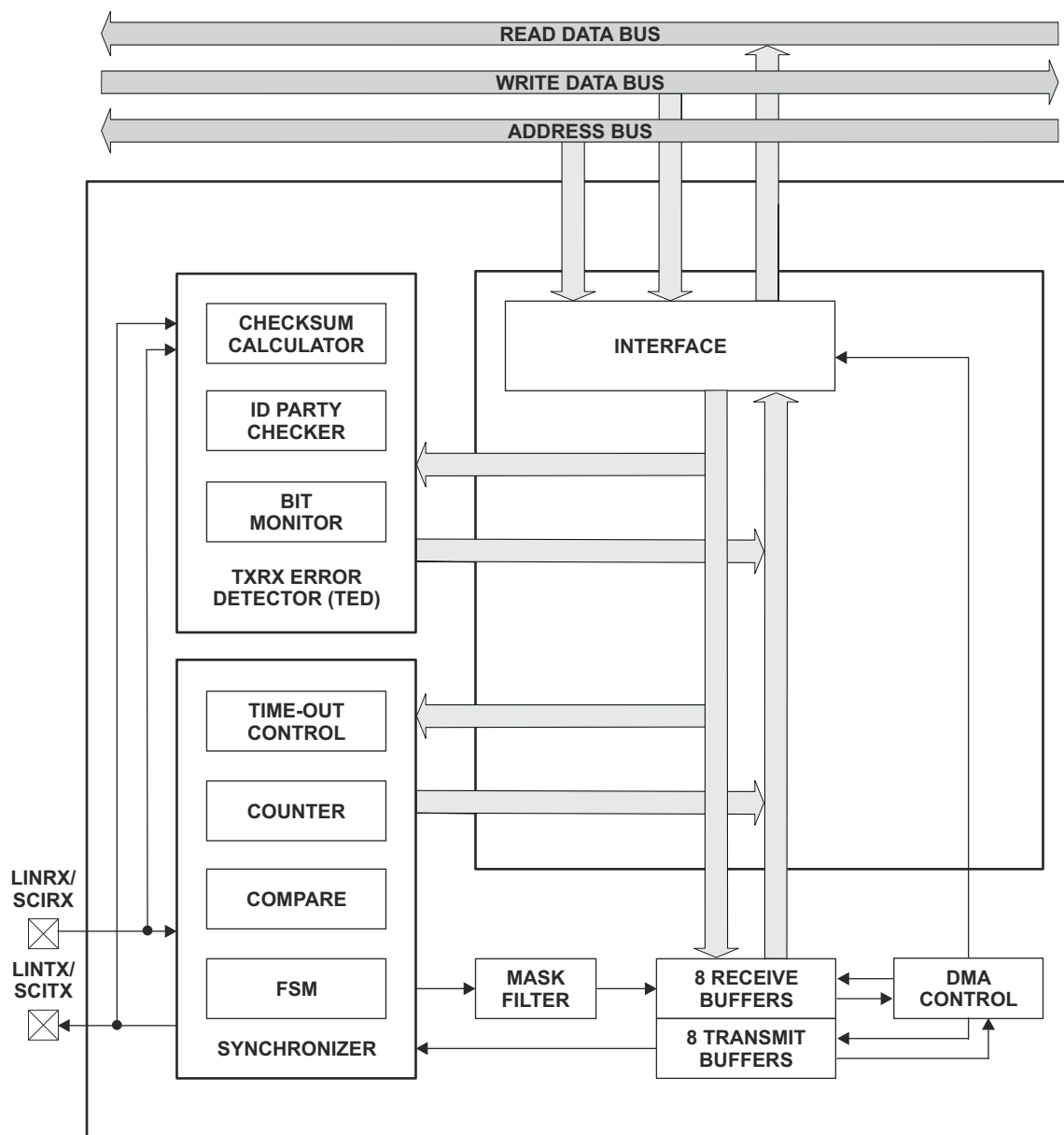
图 6-81. LIN 方框图
