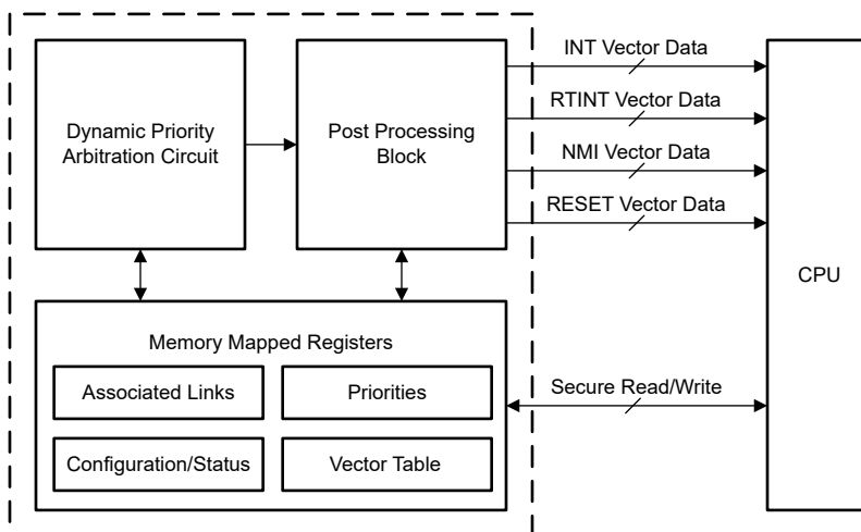
图 7-14. PIPE 架构
