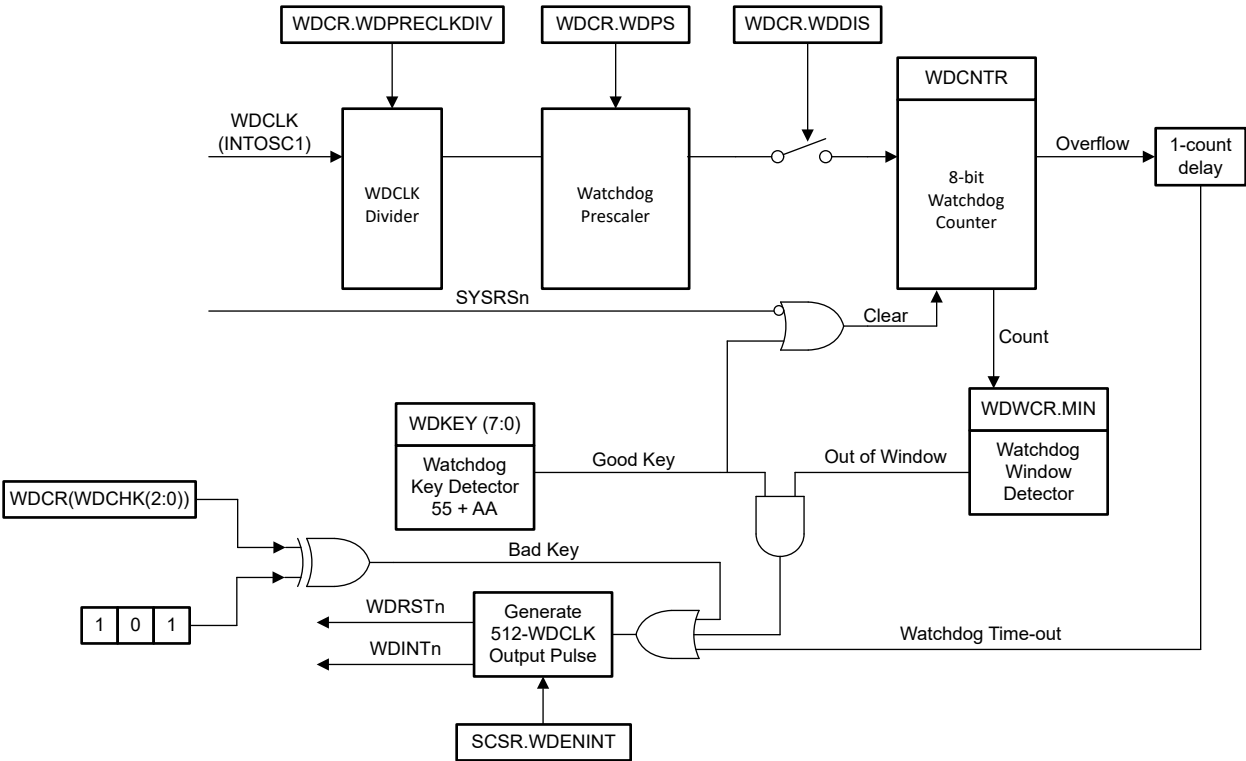
图 7-20. 窗口看门狗
