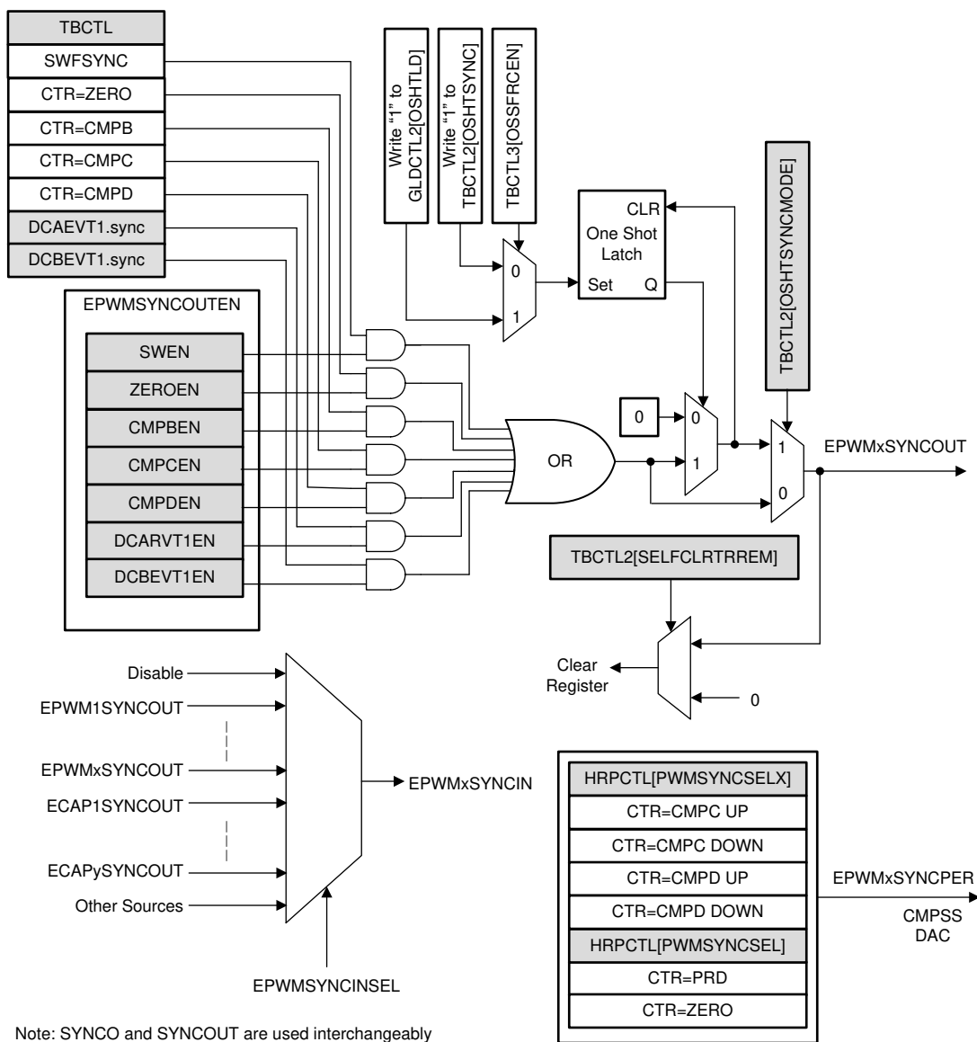
图 6-59. 同步链架构
