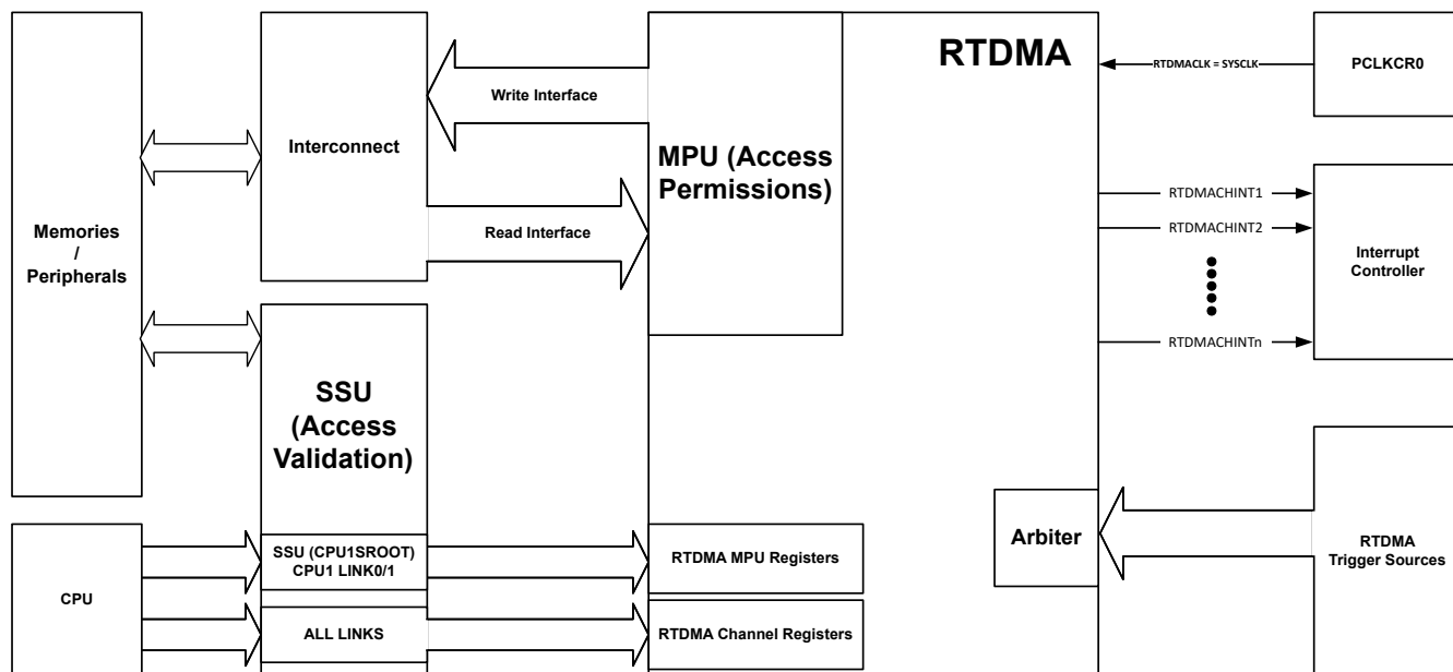
图 6-22. RTDMA 方框图
