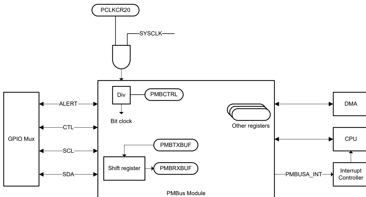
图 6-75. PMBus 方框图
