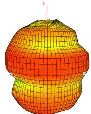
6525 MHz
