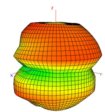
7125 MHz
