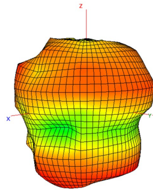
6525 MHz
