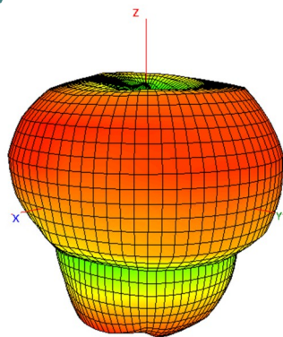
2450 MHz
