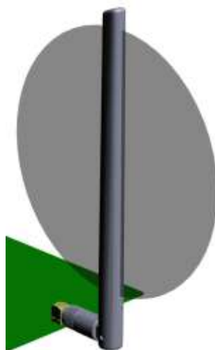
YZ-Plane Gain
