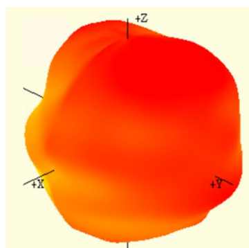
1217 MHz
