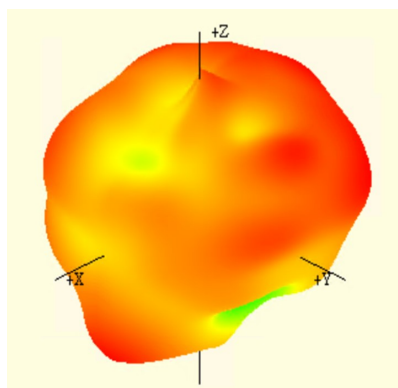
2400 MHz
