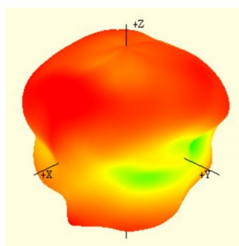
1164 MHz
