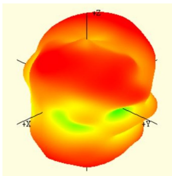
1217 MHz
