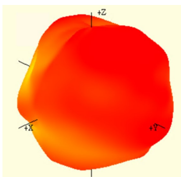
1227MHz
