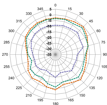
1164 MHz
