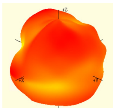
1164 MHz
