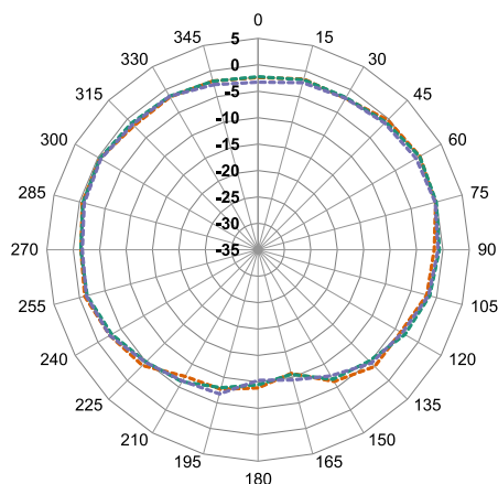
2450 MHz
