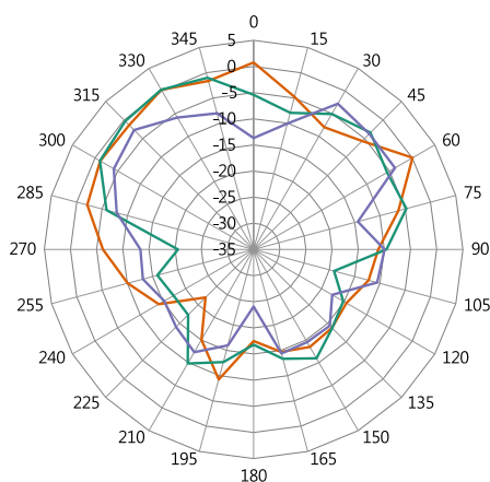
6525 MHz
