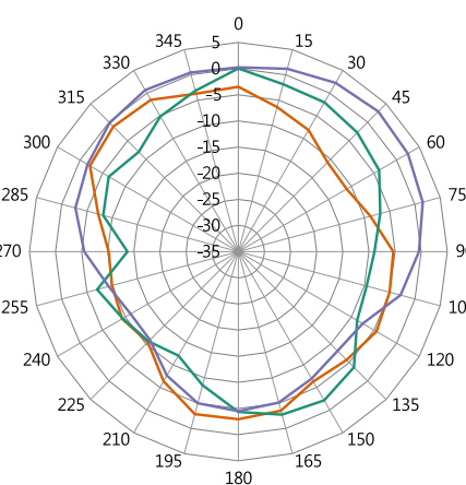
YZ-Plane Gain
