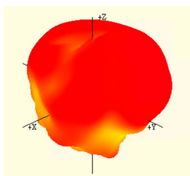
2450 MHz
