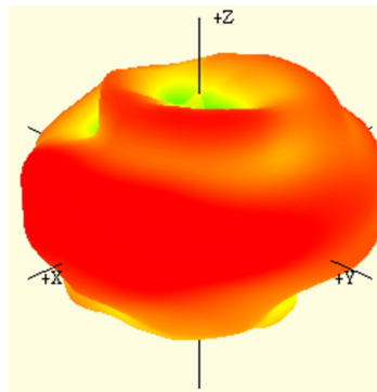
2200 MHz
