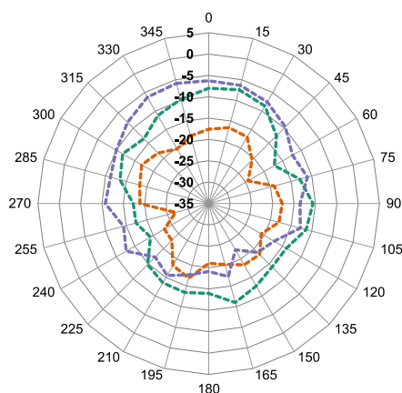
1164 MHz
