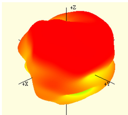
4200 MHz
