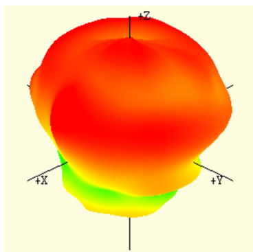
1217 MHz
