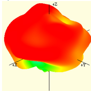
4200 MHz
