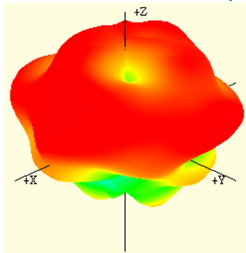
3300 MHz
