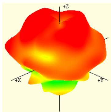
5925 MHz
