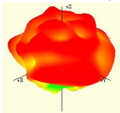
5925 MHz
