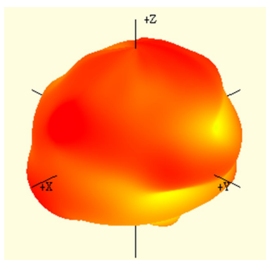
1217 MHz
