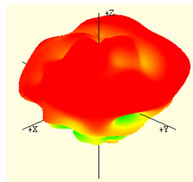
7125 MHz
