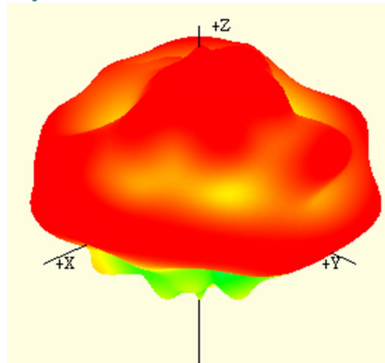
6525 MHz
