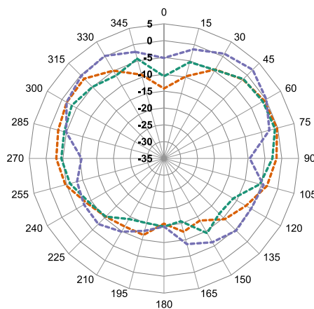
2200 MHz
