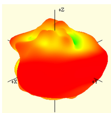
2400 MHz
