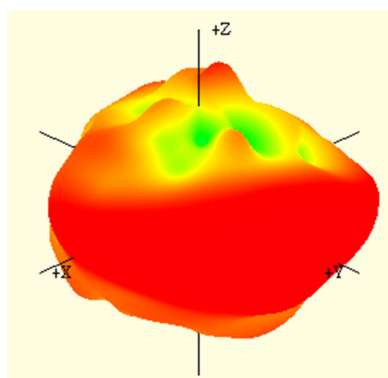
2450 MHz
