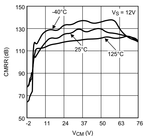
图 6-6. CMRR vs. V_{\text{CM}}
