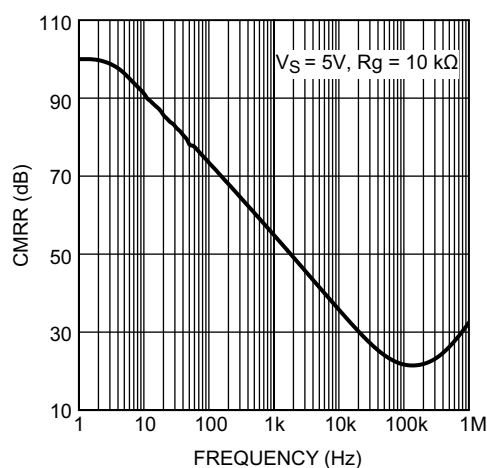
图 6-4. AC CMRR vs. Frequency
