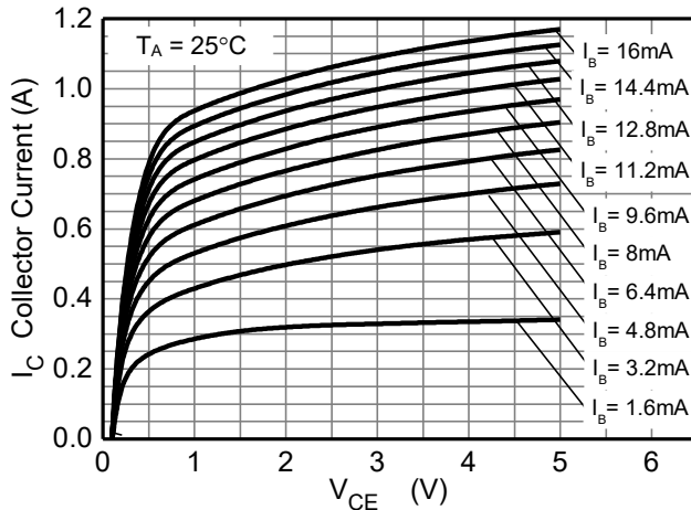
Fig.5 I_C v V_{CE} (BC817-16)
