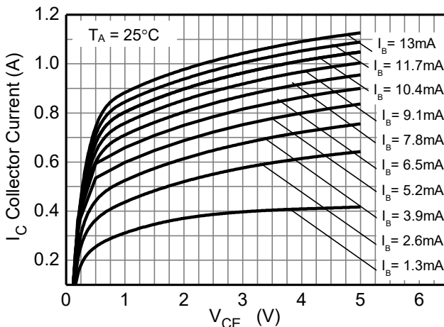
Fig.9 I_C v V_{CE} (BC817-25)
