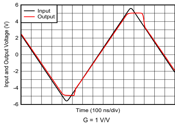
图 6-10. Input Overdrive Recovery
