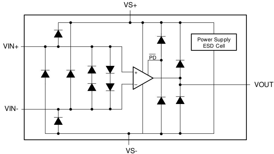
图 7-1. Internal ESD Protection
