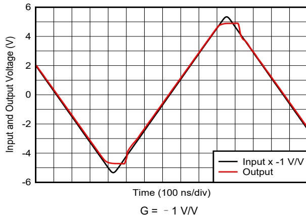
图 6-11. Output Overdrive Recovery
