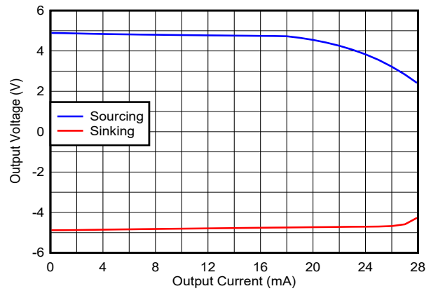
图 6-14. Output Voltage vs Load Current
