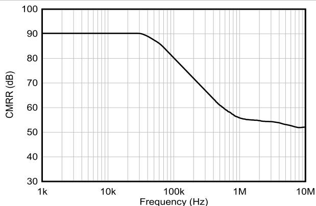
图 6-8. CMRR 与频率间的关系
