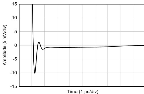
图 6-26. 小信号阶跃响应, G = 1
