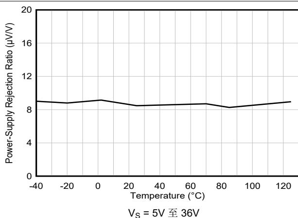
图 6-11. 电源抑制比与温度间的关系 (dB)
