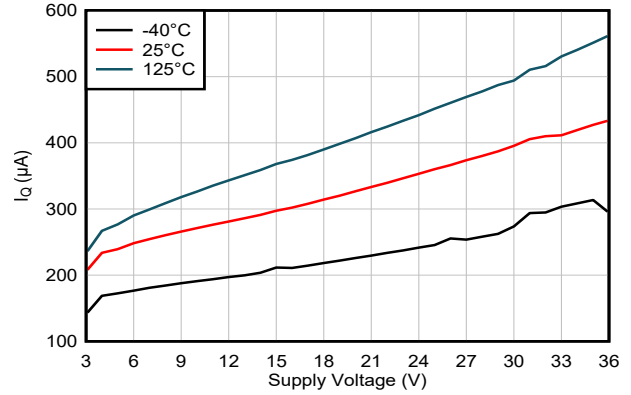
图 6-18. 静态电流与电源电压间的关系
