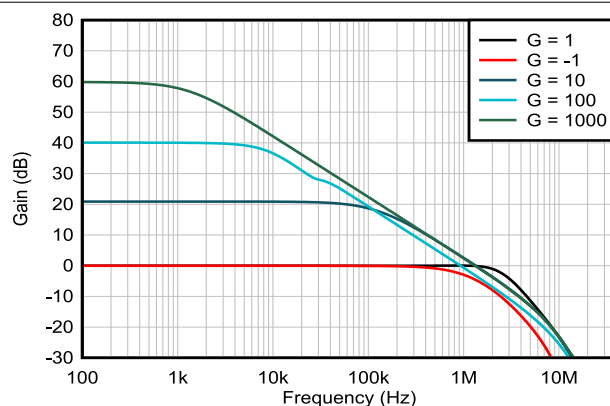
图 6-6. 闭环增益与频率间的关系
