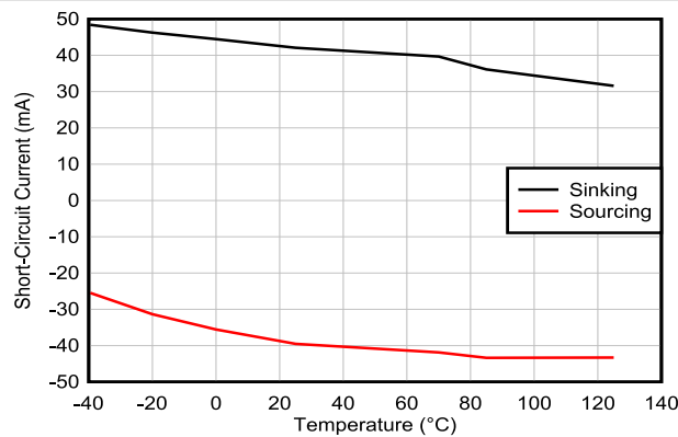
图 6-31. 短路电流与温度间的关系
