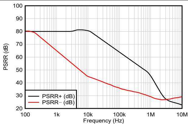
图 6-9. PSRR 与频率间的关系
